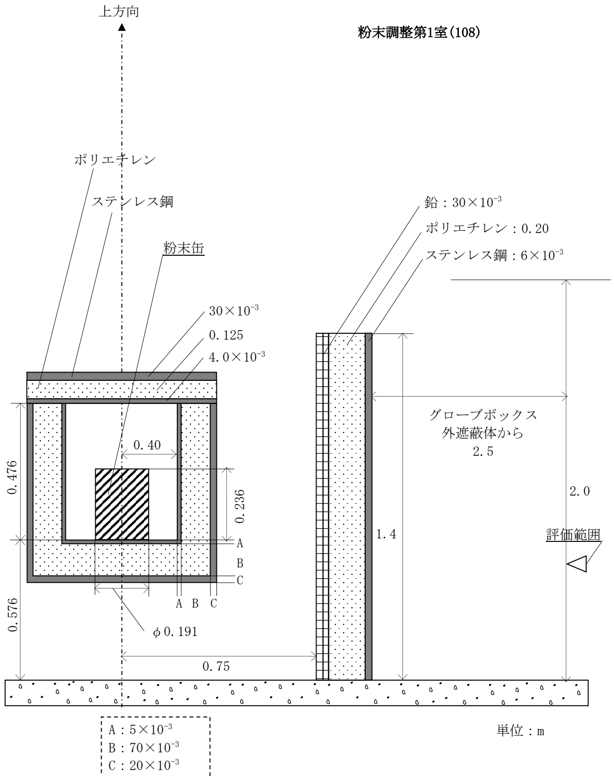
第2.2-1図(2) 原料MOX粉末缶一時保管装置 (北側) : 南方向線量率計算モデル図 (線源形状 : 有限円筒)
