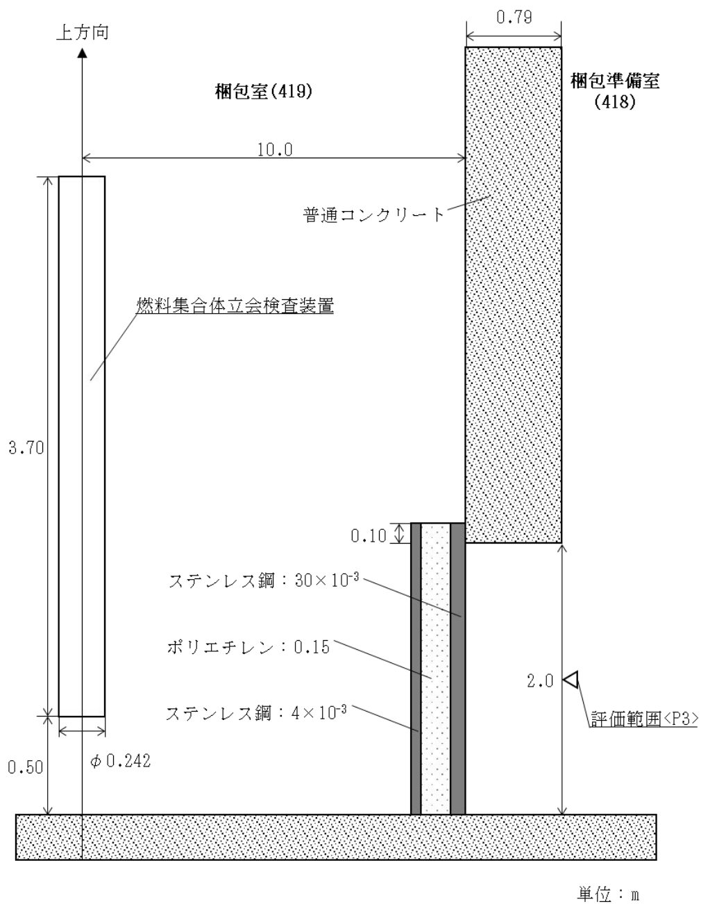
第2.2-1図(3) 燃料集合体立会検査装置：西方向線量率計算モデル図 (線源形状：有限円筒)
