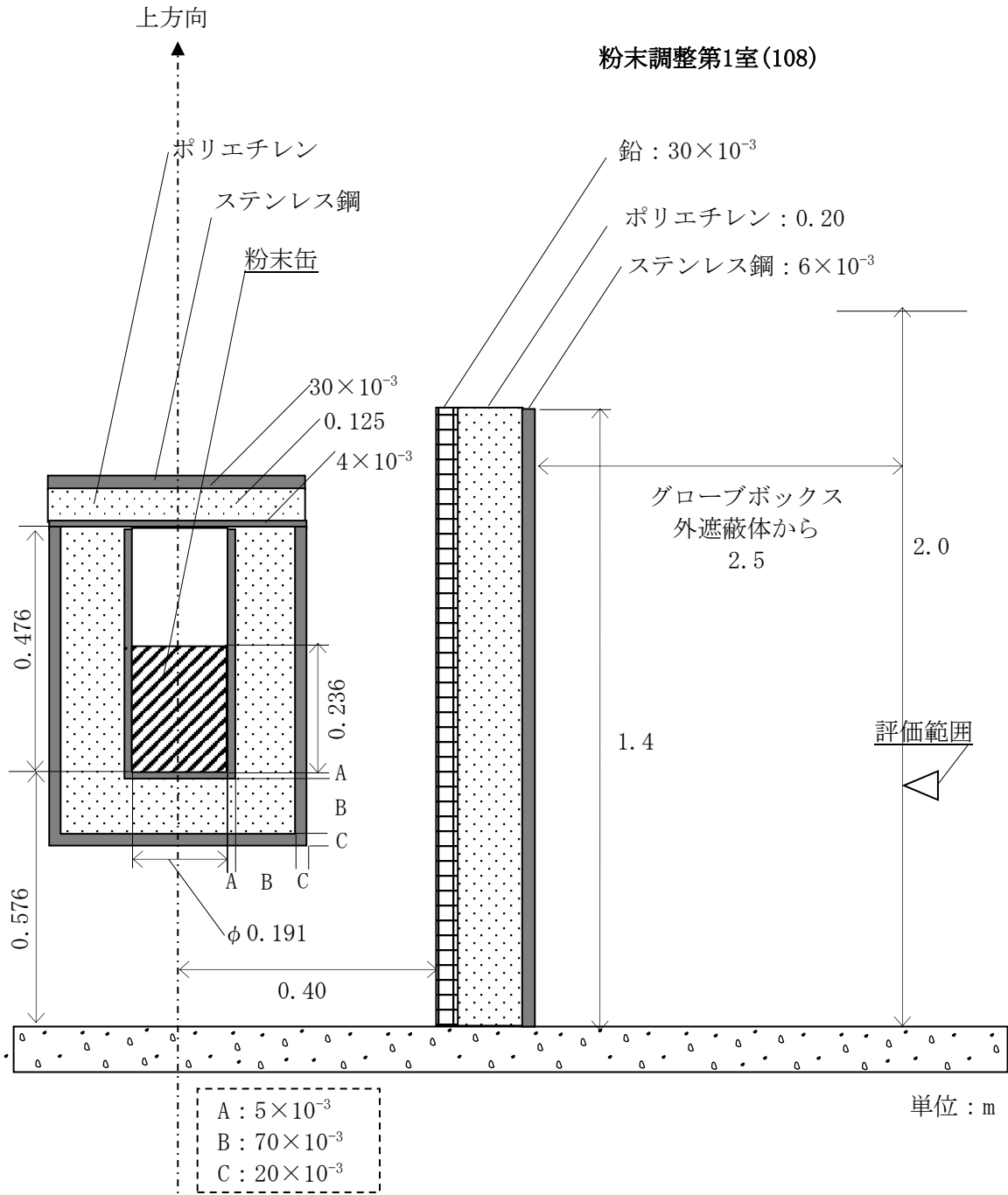
第2.2-1図(1) 原料MOX粉末缶一時保管装置(南側) : 南方向線量率計算モデル図 (線源形状 : 有限円筒)
