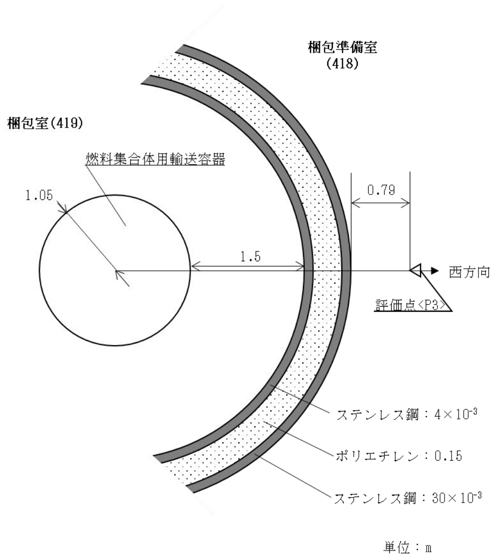
第2.2-1図(4) 燃料集合体用輸送容器：西方向線量率計算モデル図 (線源形状：球)
