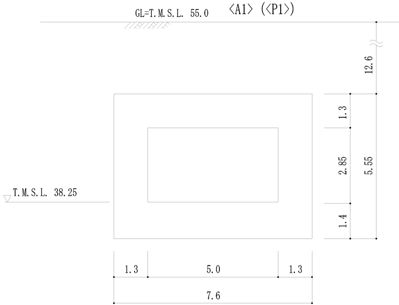
第 1-1 図(4) 貯蔵容器搬送用洞道の遮蔽計算代表点等
