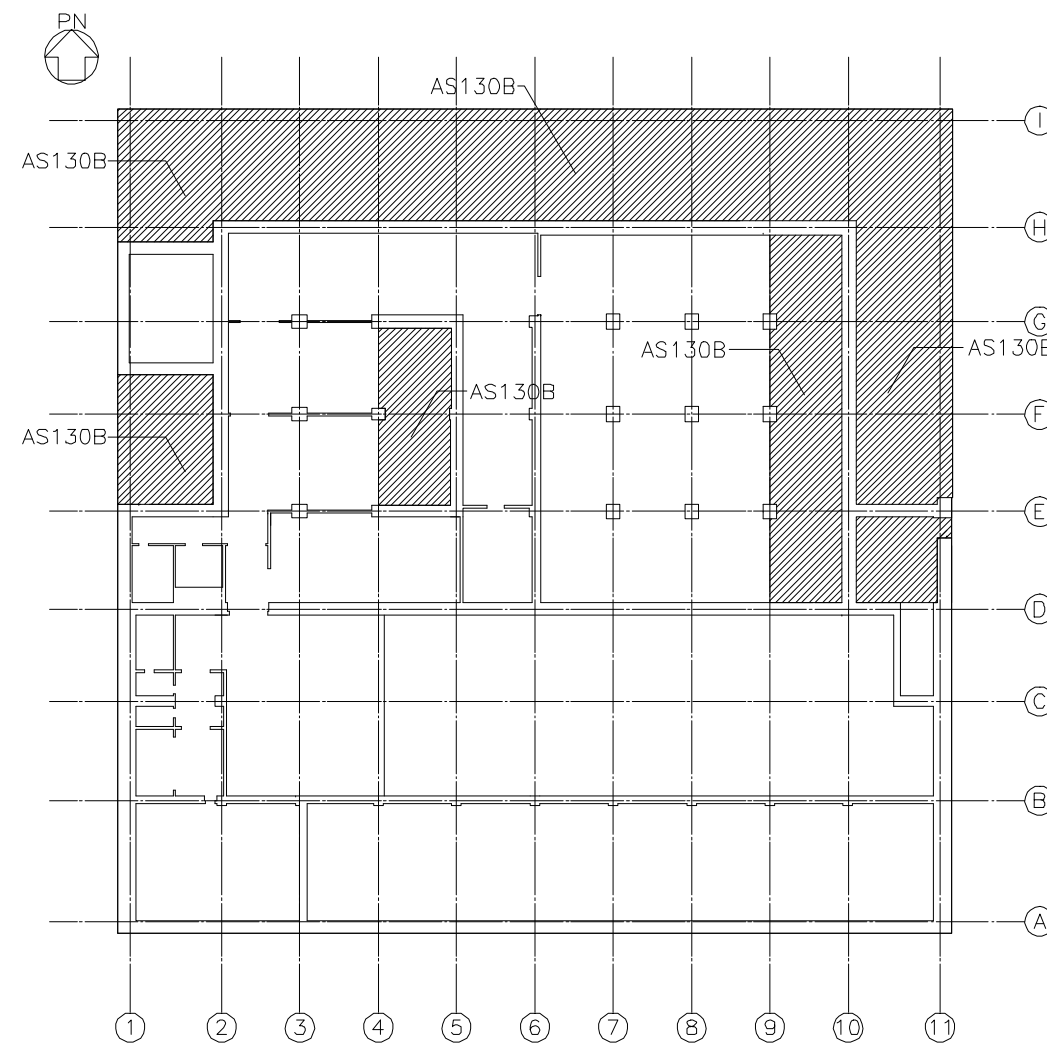
2階キープラン (T.P.61.60m) 注： は防護スラブを示す。
