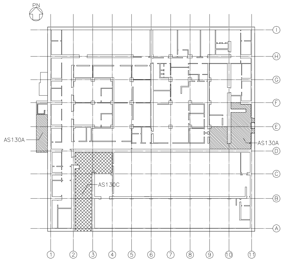
1階キープラン (T.P.55.60m) 注： は防護スラブを示す。
