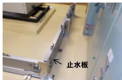
第2図 A-712 の影響評価に係る溢水経路の設定 (1/2)
