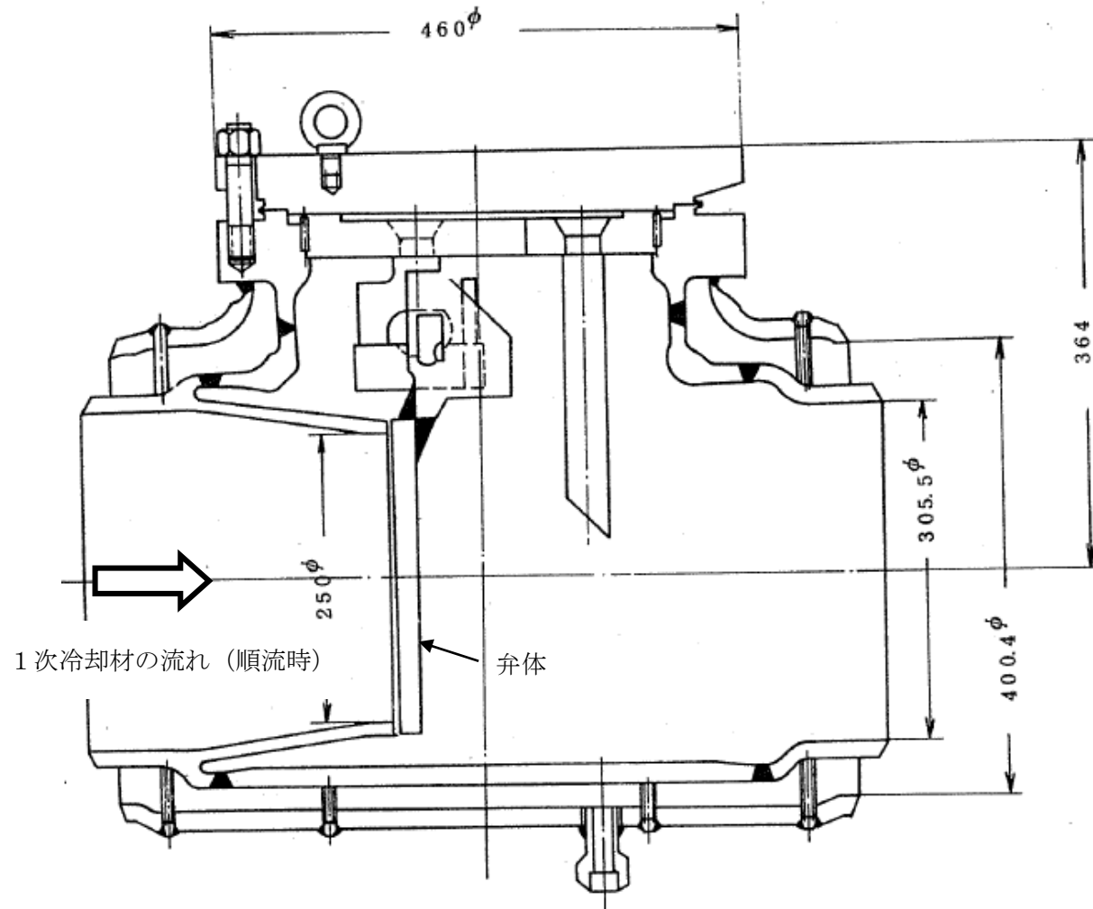
第1図 1次主冷却系逆止弁の構造
