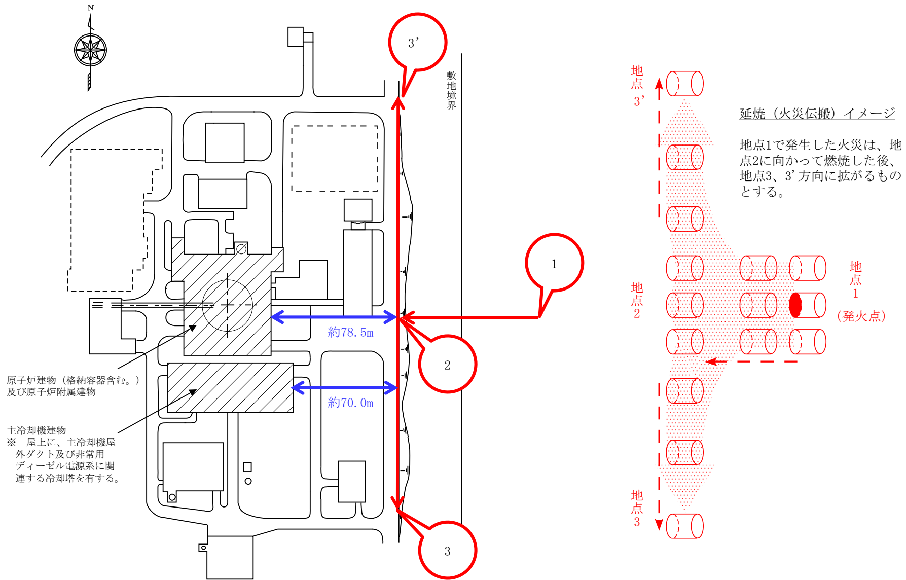
第1図 延焼 (火災伝搬) イメージ
