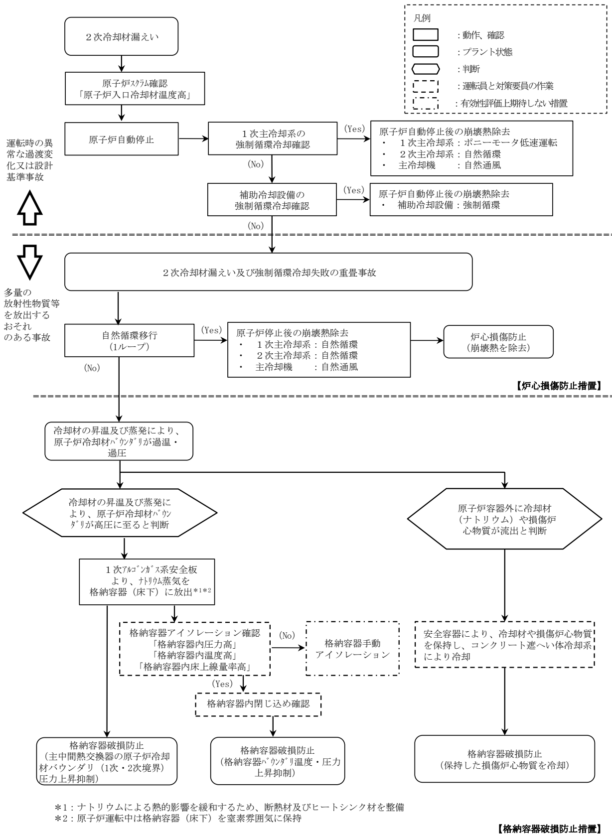
第 4.3.3.13.1 図 炉心損傷防止措置の対応手順の概要
