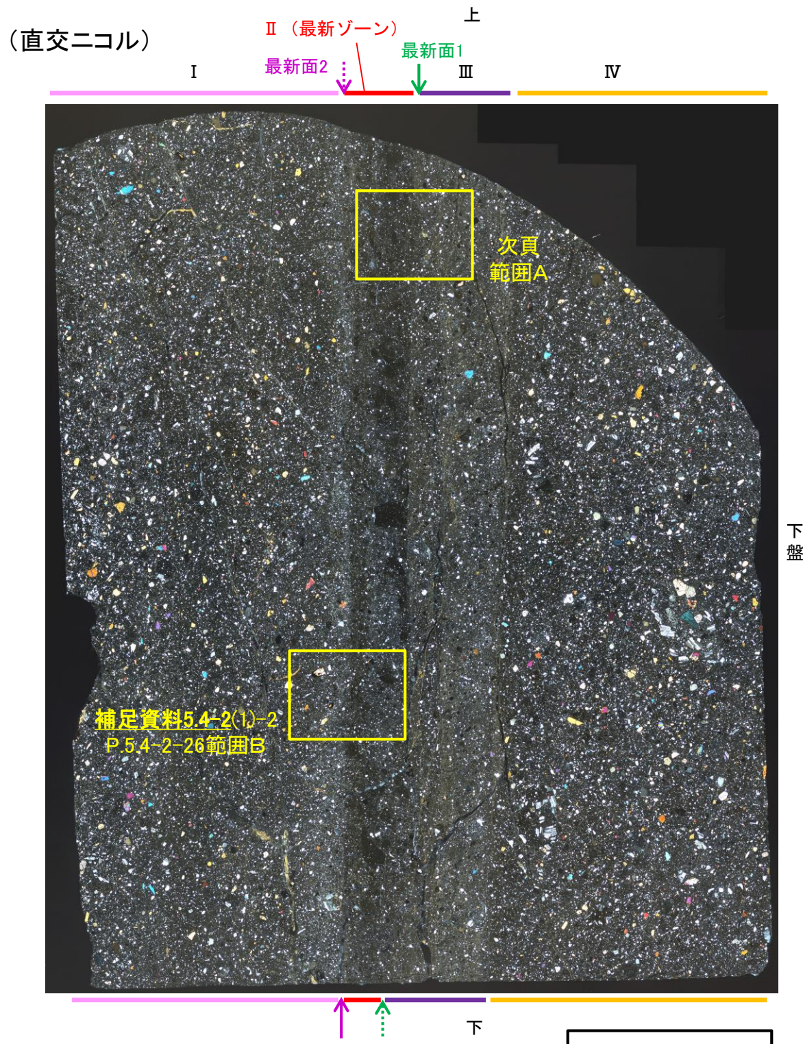
薄片①写真(H-6.6-1_71R)
