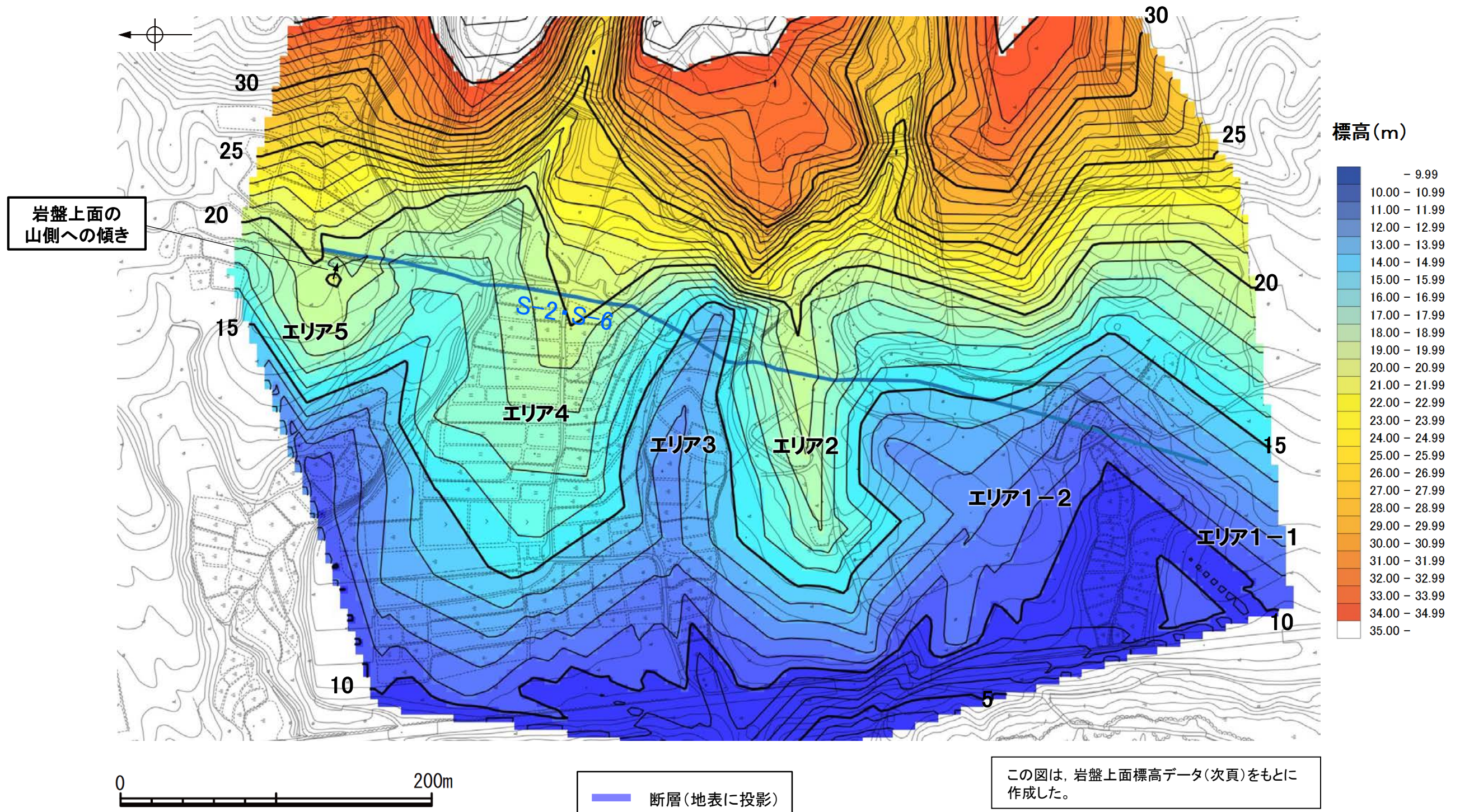
岩盤上面標高段彩図
