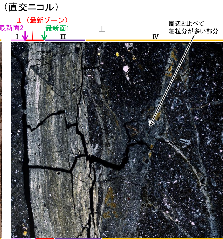
薄片①写真(M-12.5”_65R)(拡大)
