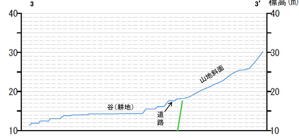
地形断面図(H:V=1:5)
