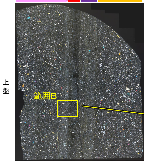
薄片①写真(H-6.6-1_71R)
