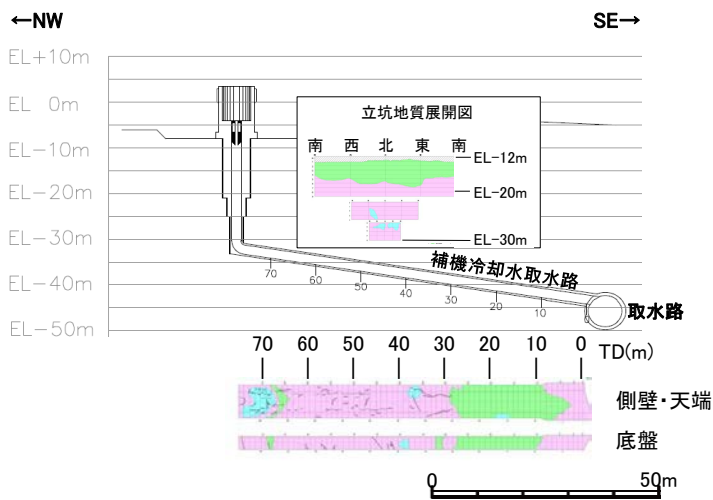
ⓑ-ⓑ' 断面図及び地質展開図
