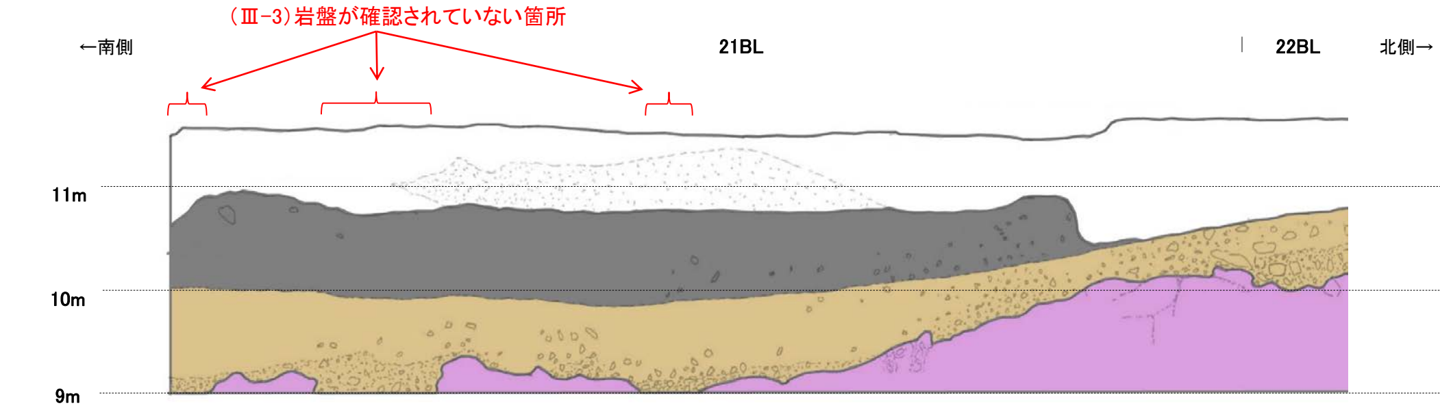
防潮堤設置時スケッチ[21BL, 22BL]①
