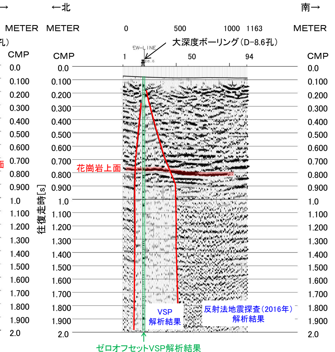
反射法地震探査(2016年)・VSP探査結果 (南北測線:時間断面)
