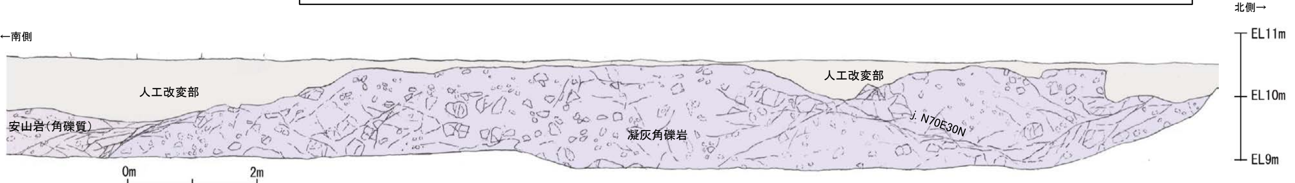
再掘削 ④トレンチ スケッチ
