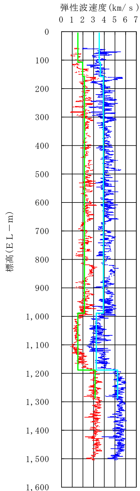
PS検層結果
