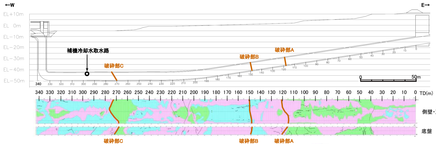
ⓐ-ⓐ' 断面図及び地質展開図(取水路)
