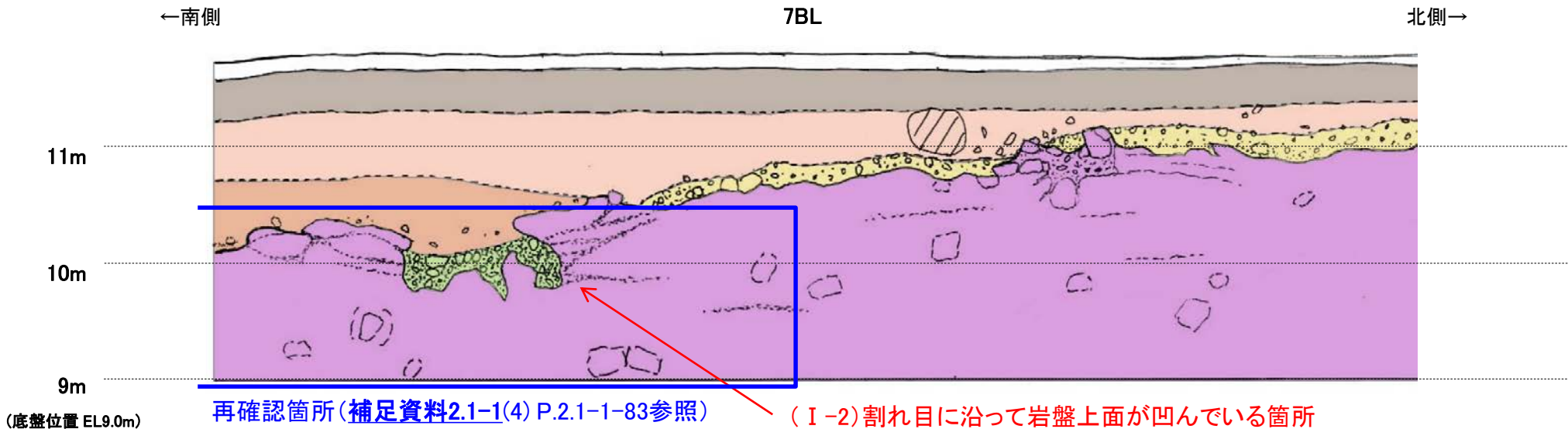
防潮堤設置時スケッチ[7BL]
