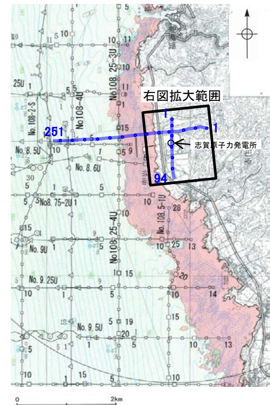
調査位置図(石川県, 1997に一部加筆)
