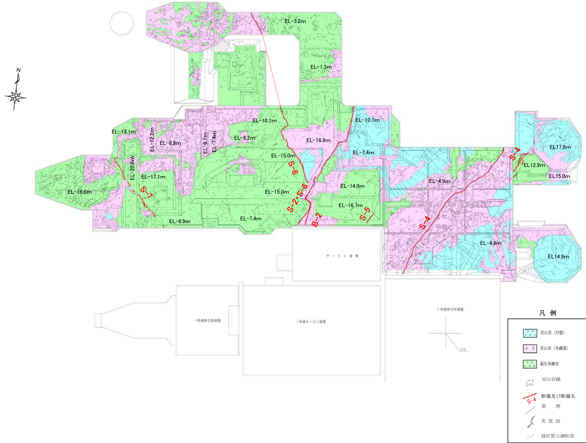
2号機基礎掘削面スケッチ
