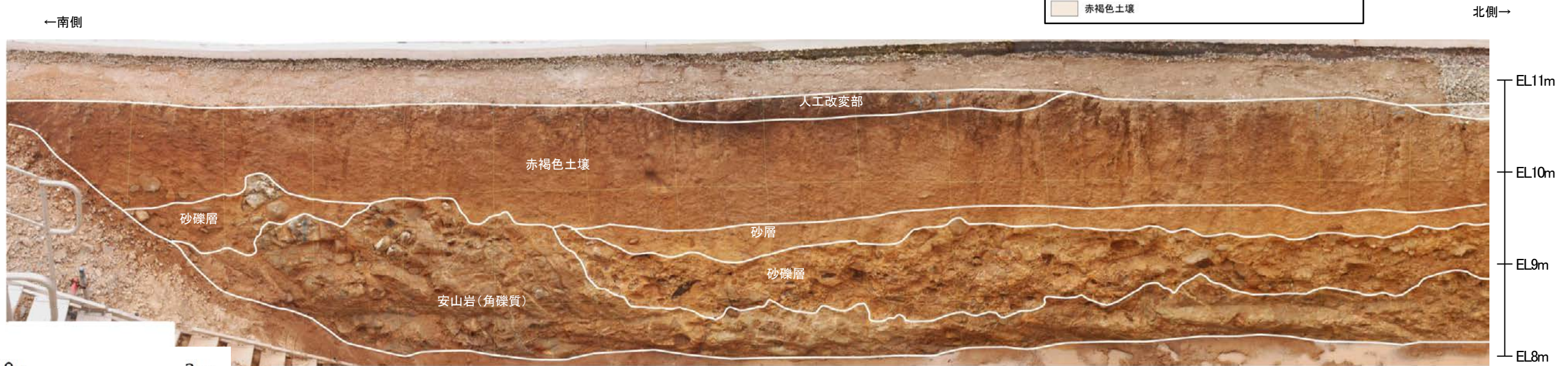
再掘削 ⑥トレンチ 写真
