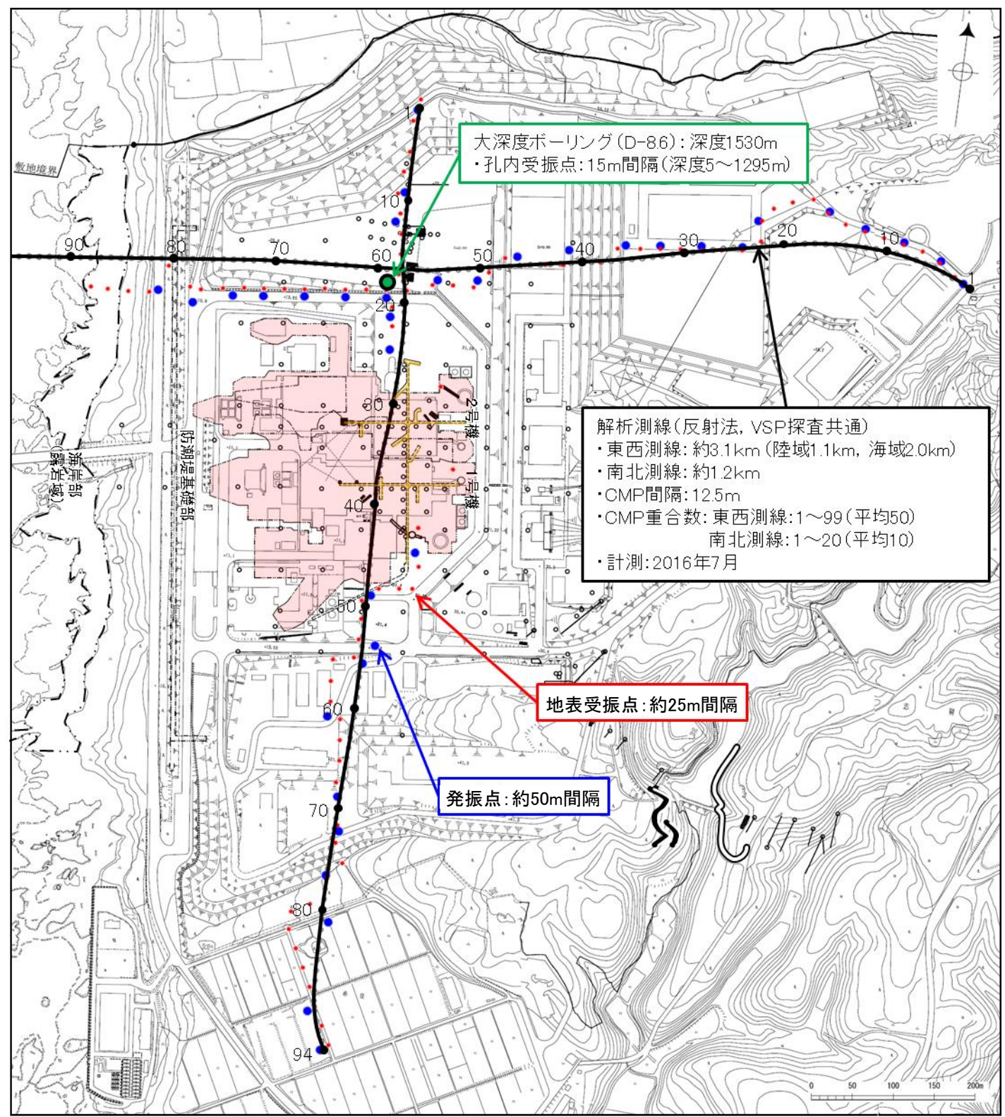
調査位置図(拡大範囲)
