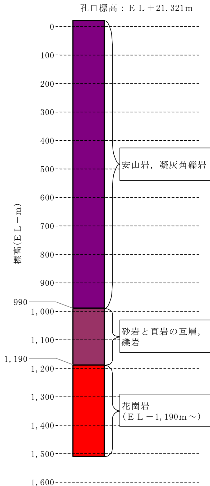
柱状概要図
