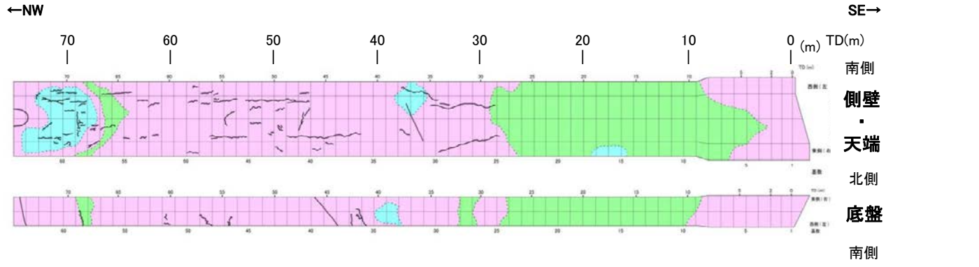
2号機補機冷却水取水路地質展開図
