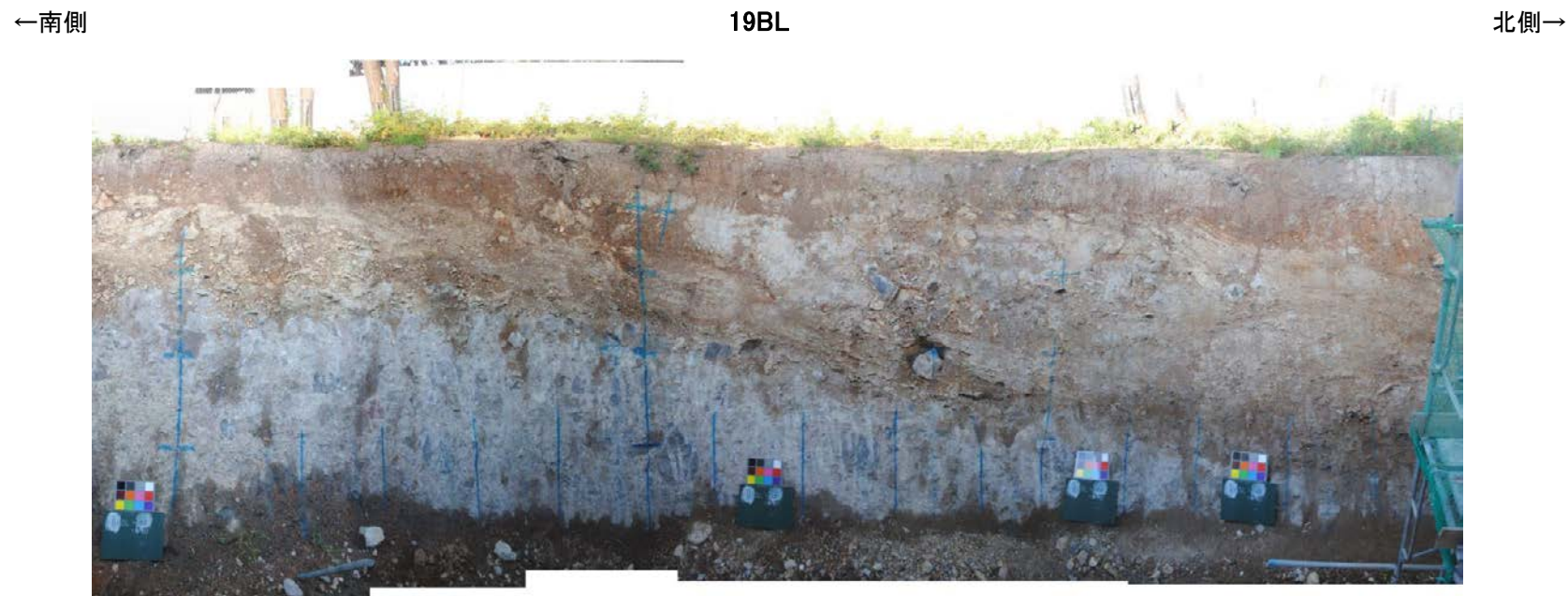
防潮堤設置時写真[19BL]
