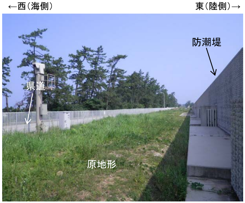
地盤改良工事前の写真 (原地形が残っている)
