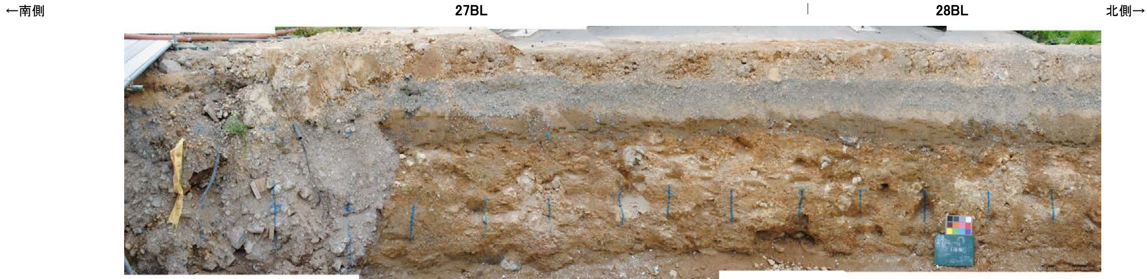
防潮堤設置時写真[27BL, 28BL]①
