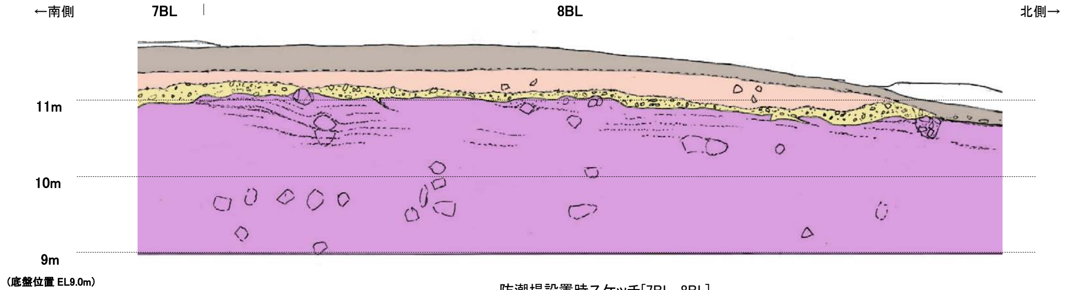
防潮堤設置時スケッチ[7BL, 8BL]
