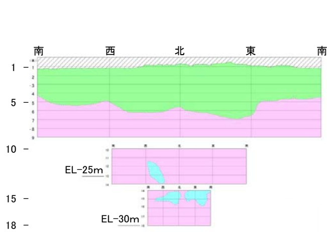
2号機取水路地質展開図
