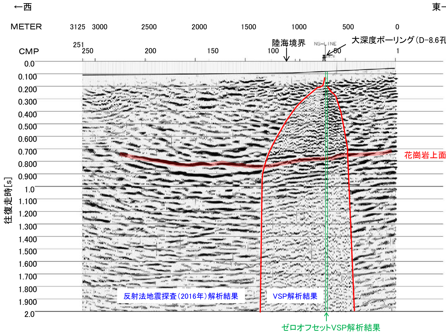
反射法地震探査(2016年)・VSP探査結果 (東西測線:時間断面)
