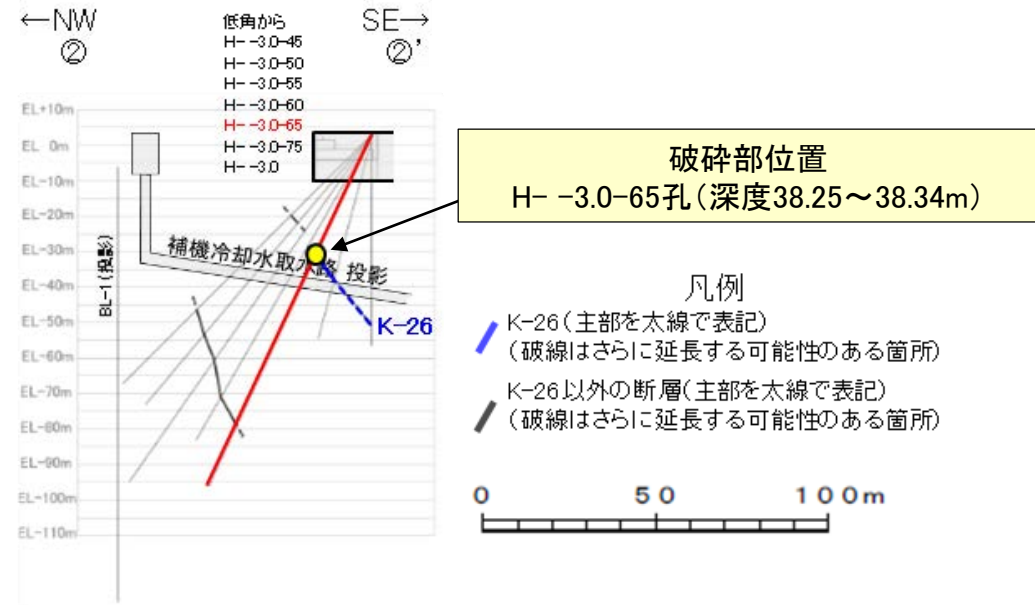
②-②' 断面図
