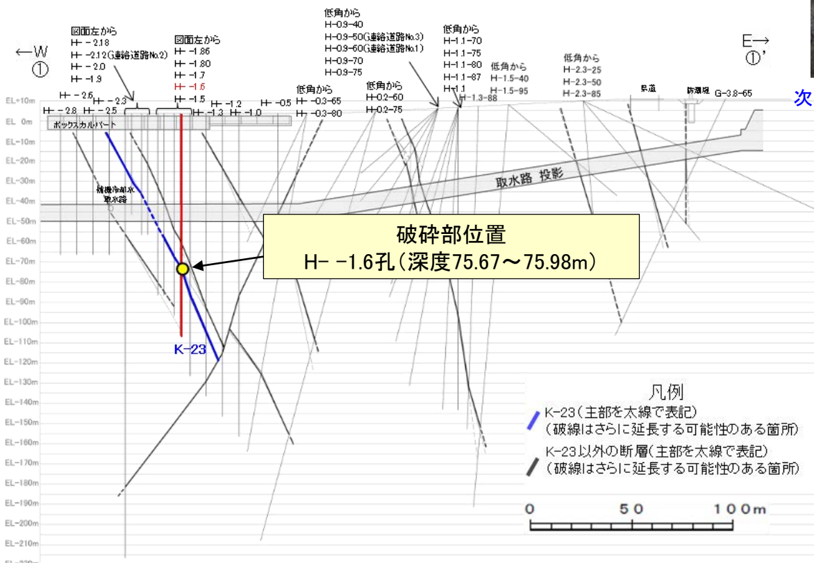
①-①'断面図
