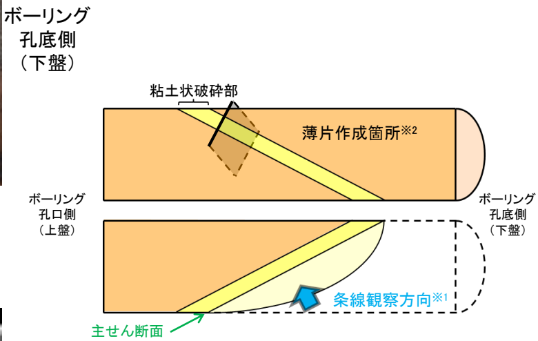
半割コア断面模式図 上: 薄片作成側 下: 条線観察側
