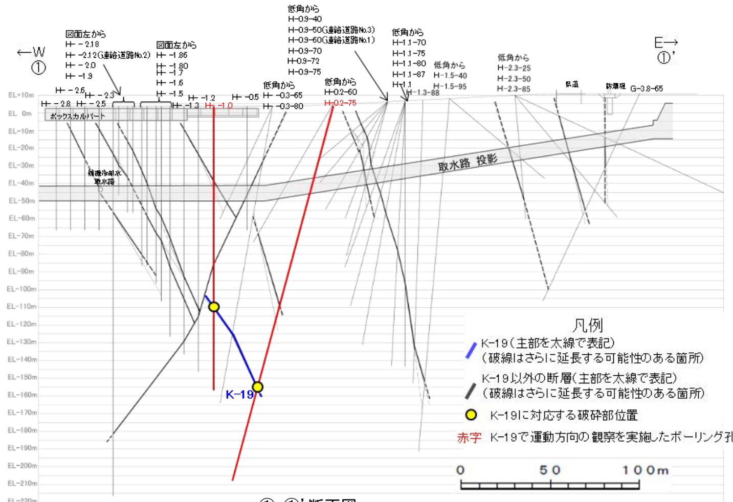
①-①' 断面図
