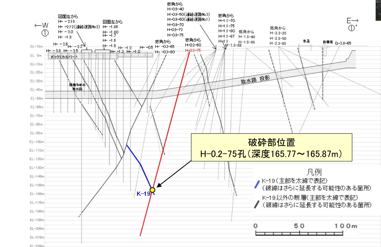
①-①' 断面図
