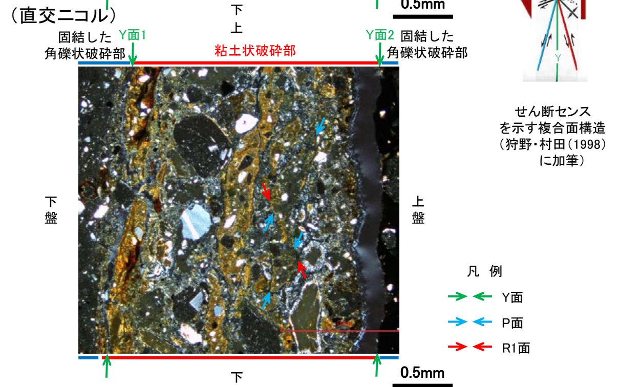
詳細観察範囲写真
