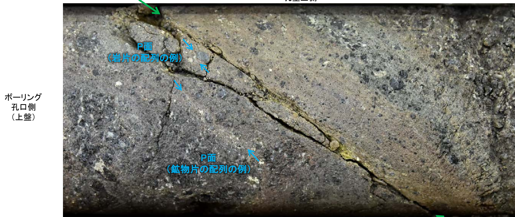
拡大範囲写真(右は構造等を加筆)
