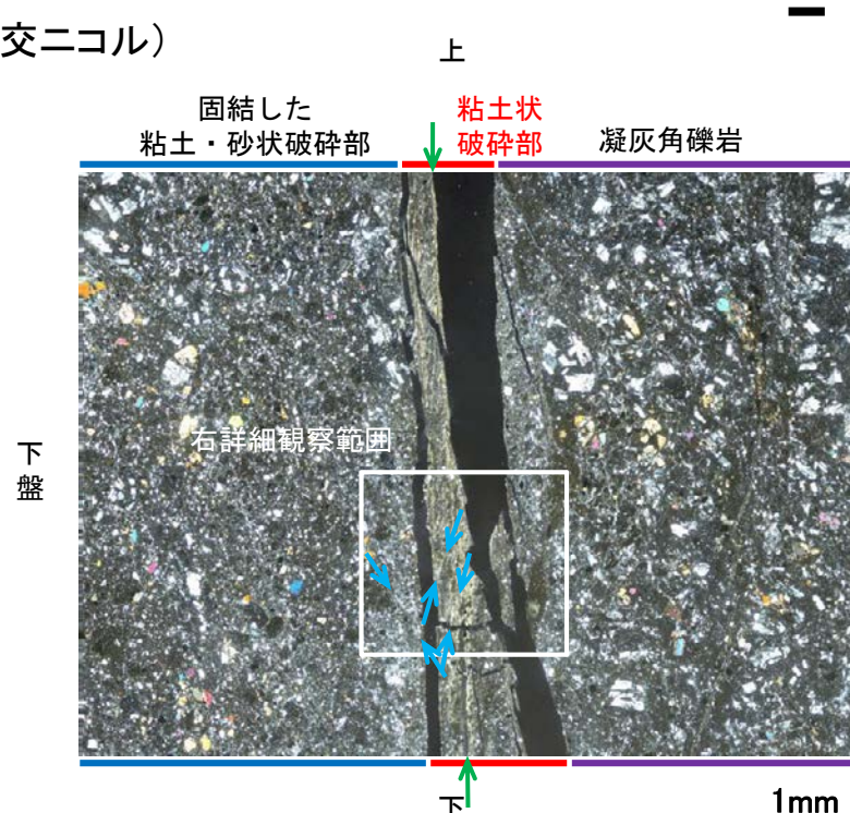
拡大範囲写真
