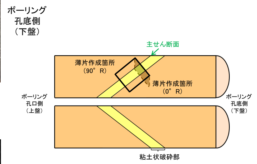
半割コア断面模式図
