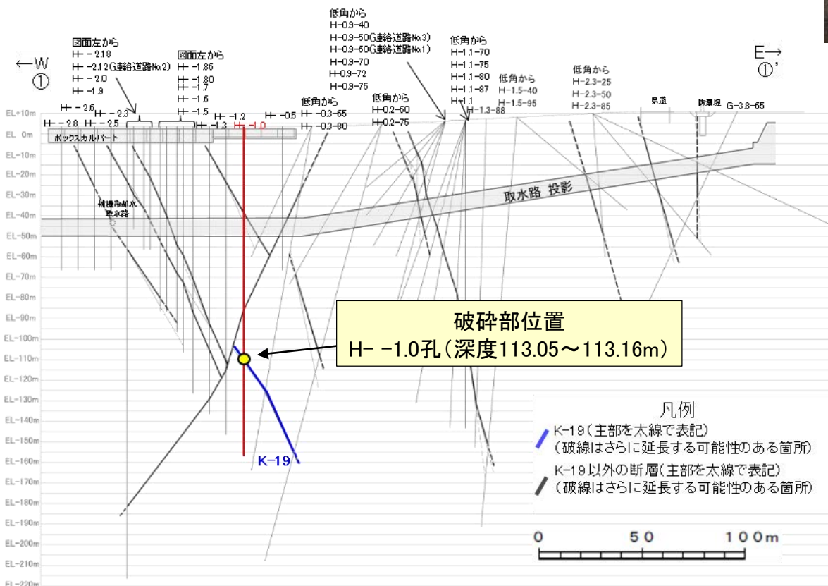
①-①' 断面図
