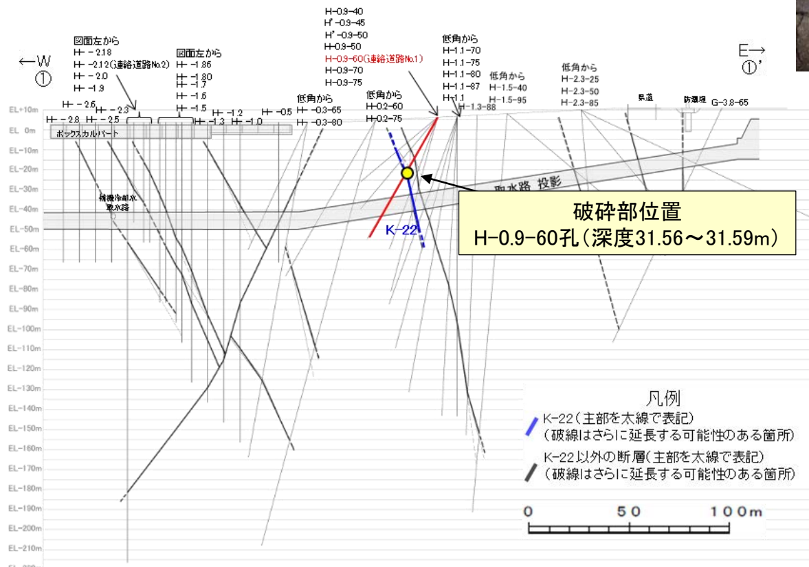
①-①'断面図
