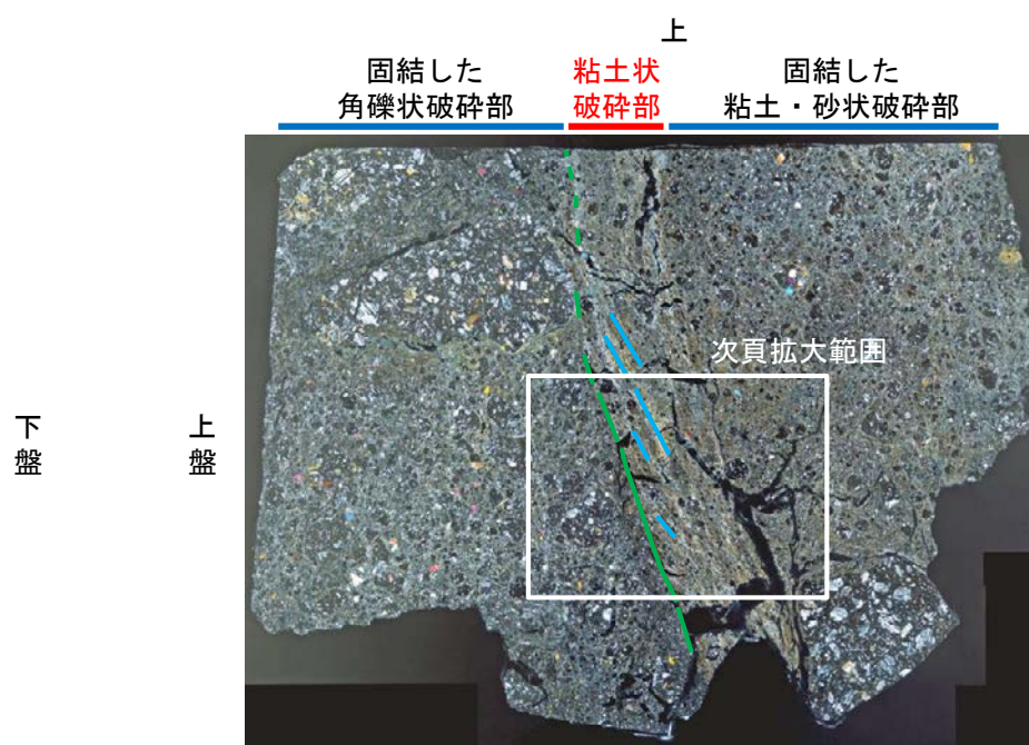
薄片写真(H-0.2-75_34R)(右は構造等を加筆)
