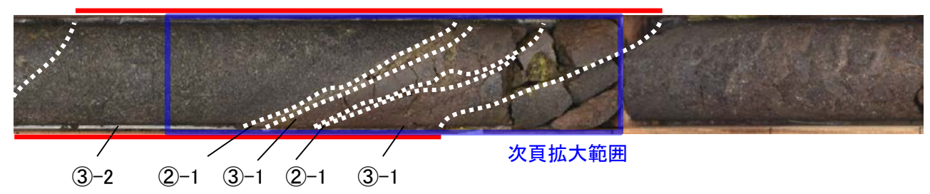
コア写真(H- -2.18孔, 破砕部区分を加筆)
