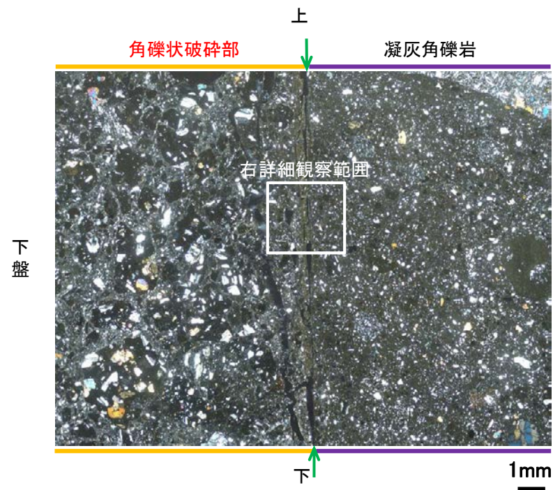
拡大範囲写真
