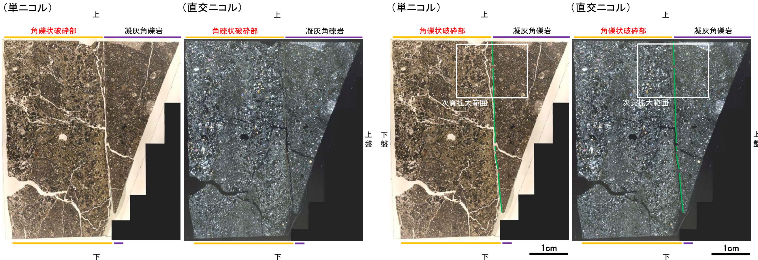
薄片写真(H-2.0_85R) (右は構造等を加筆)
