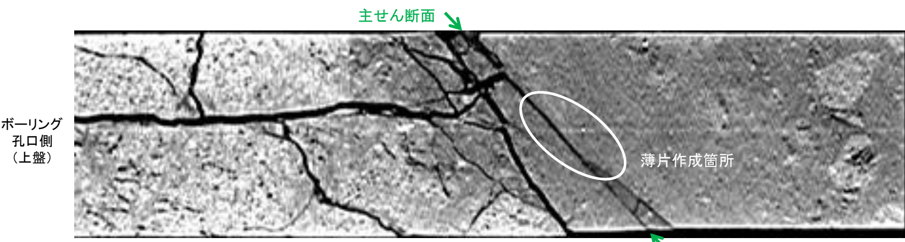
コア拡大写真(H-0.9-60孔)
