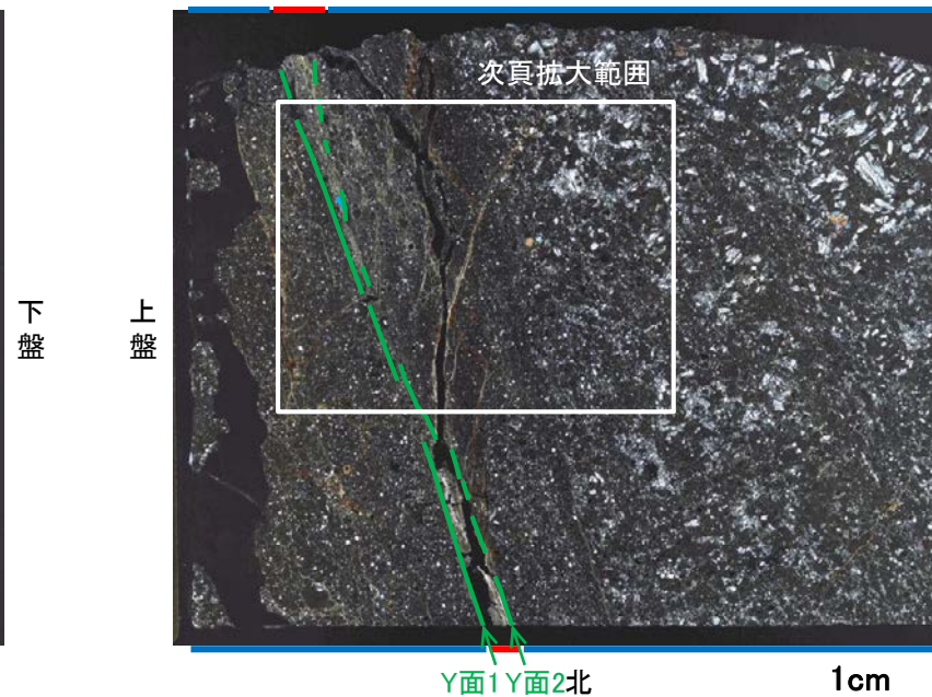
薄片写真(H-0.9-60_0R)(右は構造等を加筆)
