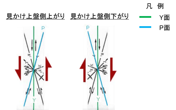
せん断センスを示す複合面構造 (狩野・村田(1998)に加筆)
