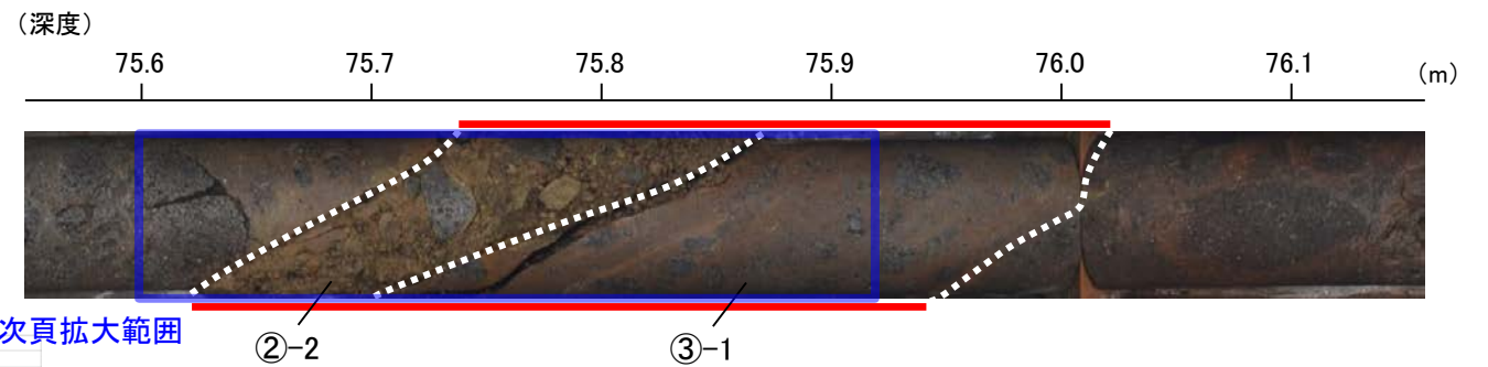
コア写真(H- -1.6孔, 破砕部区分を加筆)
