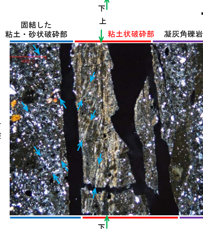
詳細観察範囲写真
