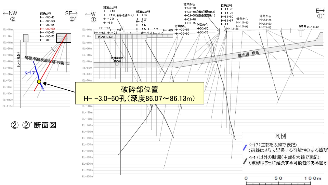
①-①' 断面図
