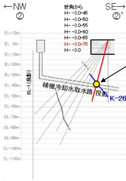
②-②' 断面図
