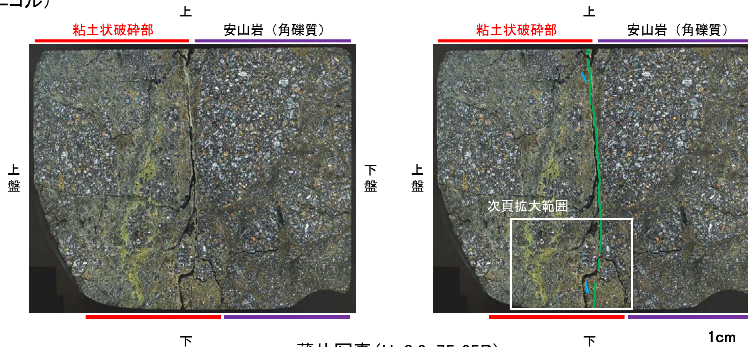
薄片写真(H-0.2-75_65R) (右は構造等を加筆)
