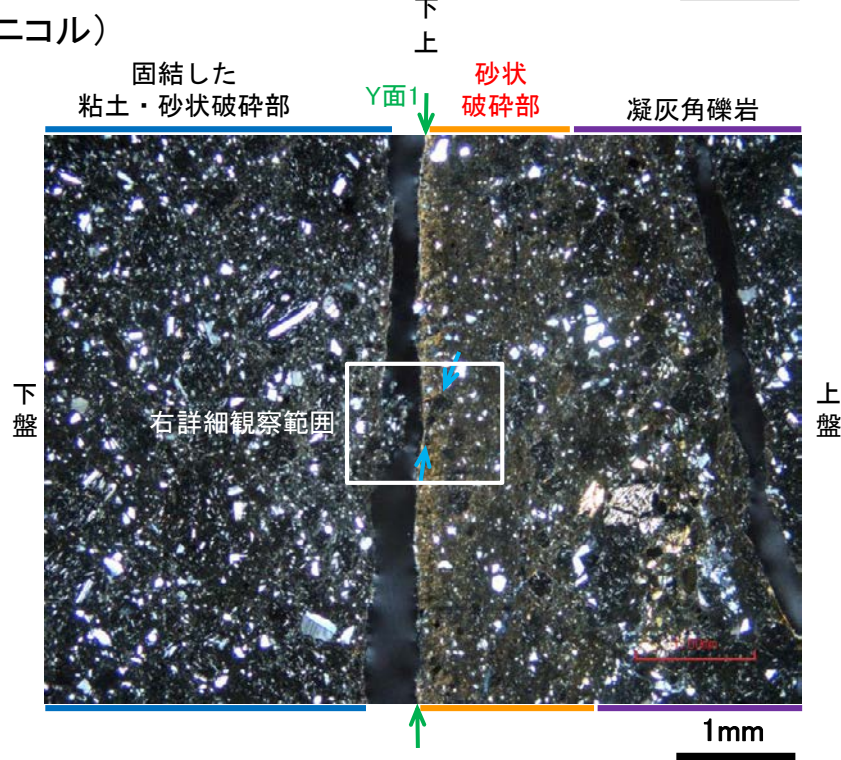
拡大範囲②写真
