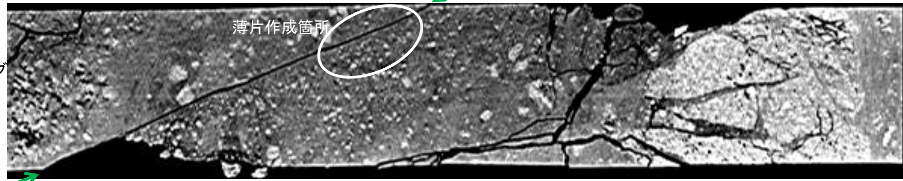
CT画像(H- -2.0孔)
