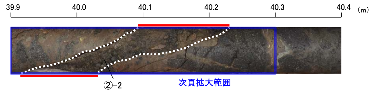
コア写真(H- -2.0孔, 破砕部区分を加筆)
