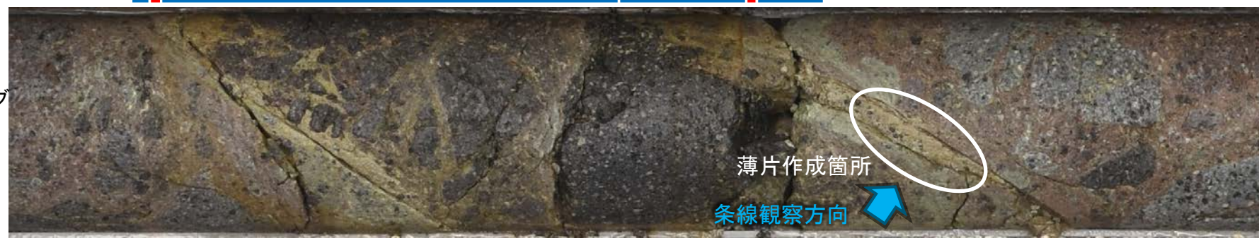
コア拡大写真(H- -3.0-75孔)
