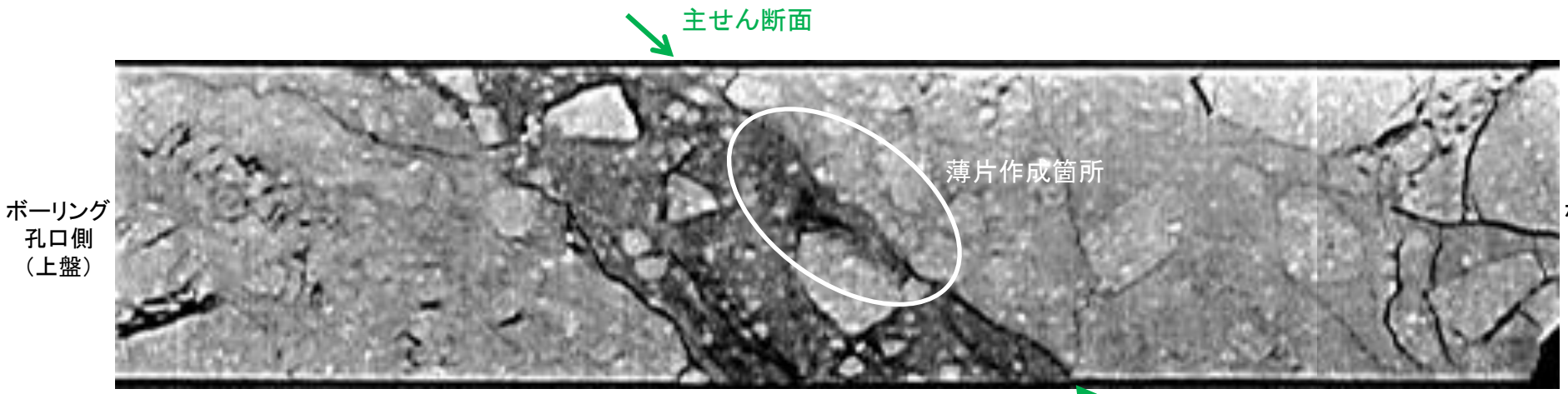
コア拡大写真(H-0.2-75孔)
