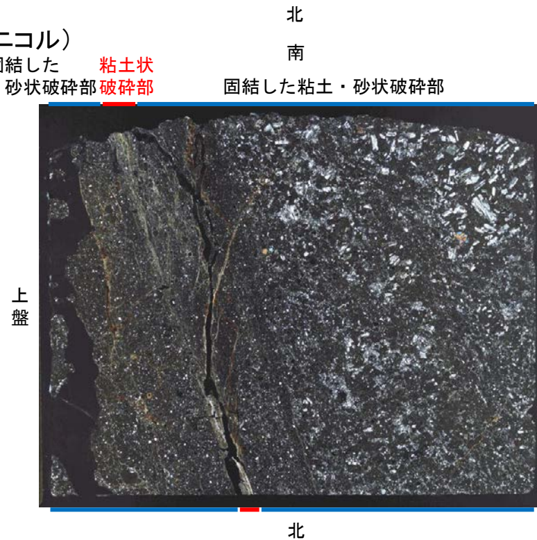
薄片写真(H-0.9-60_0R)(右は構造等を加筆)
