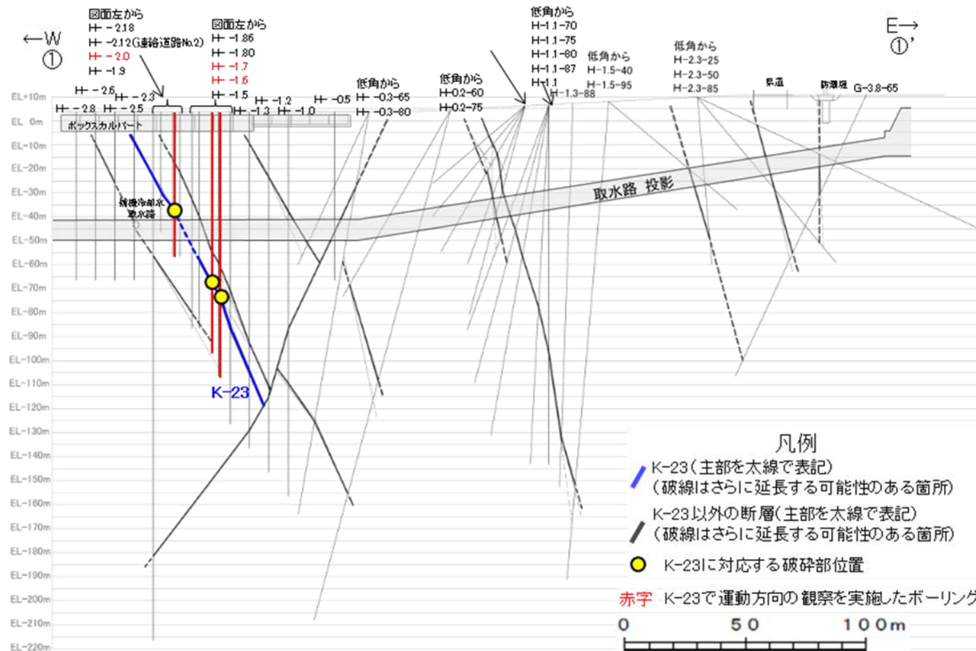
①-①' 断面図
