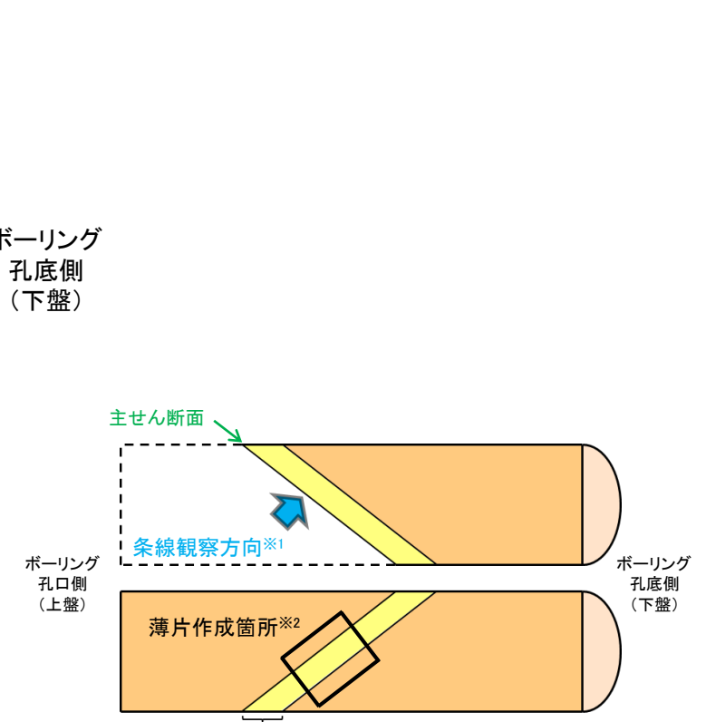
半割コア断面模式図 上: 条線観察側 下: 薄片作成側
