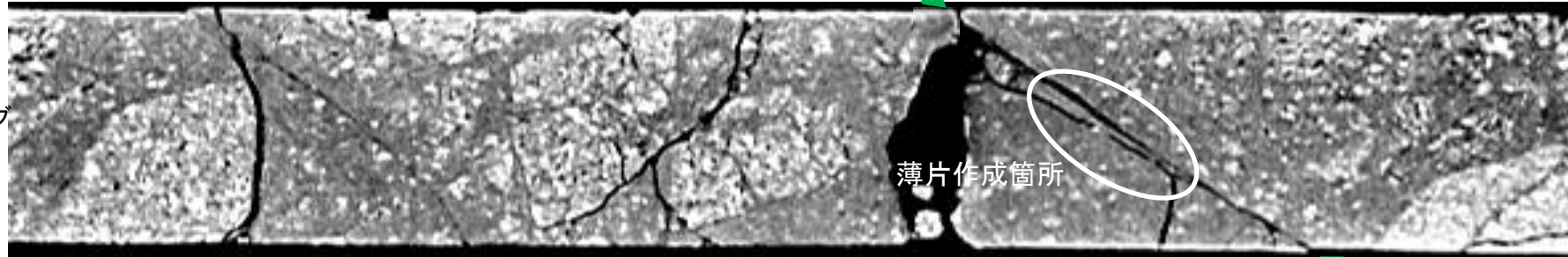
CT画像(H- -3.0-75孔)
