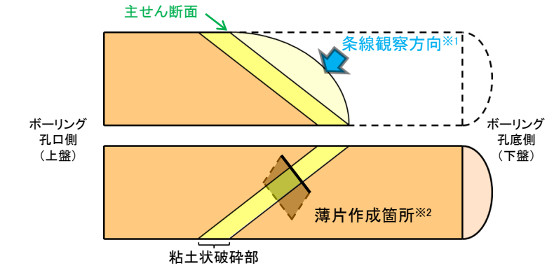
半割コア断面模式図 上: 条線観察側 下: 薄片作成側
