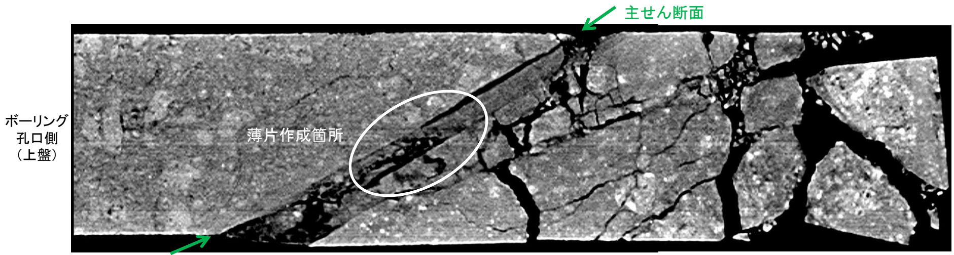
CT画像(H- -2.18孔)
