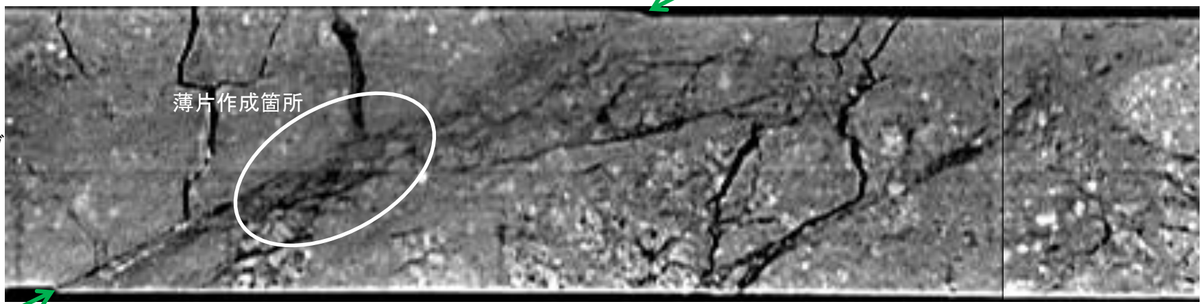
CT画像(H- -2.6孔)
