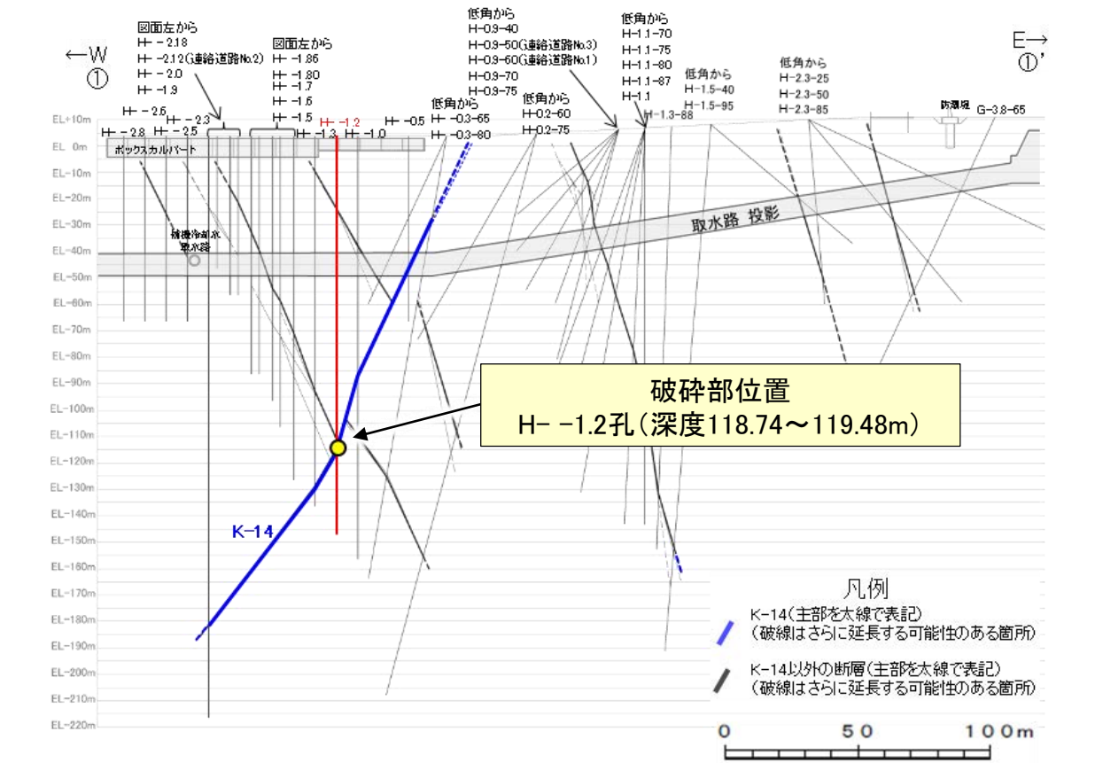
①-①'断面図
