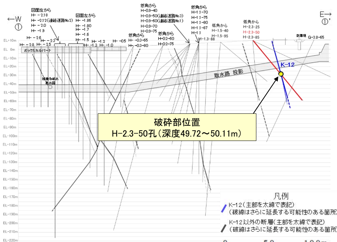
①-①'断面図
