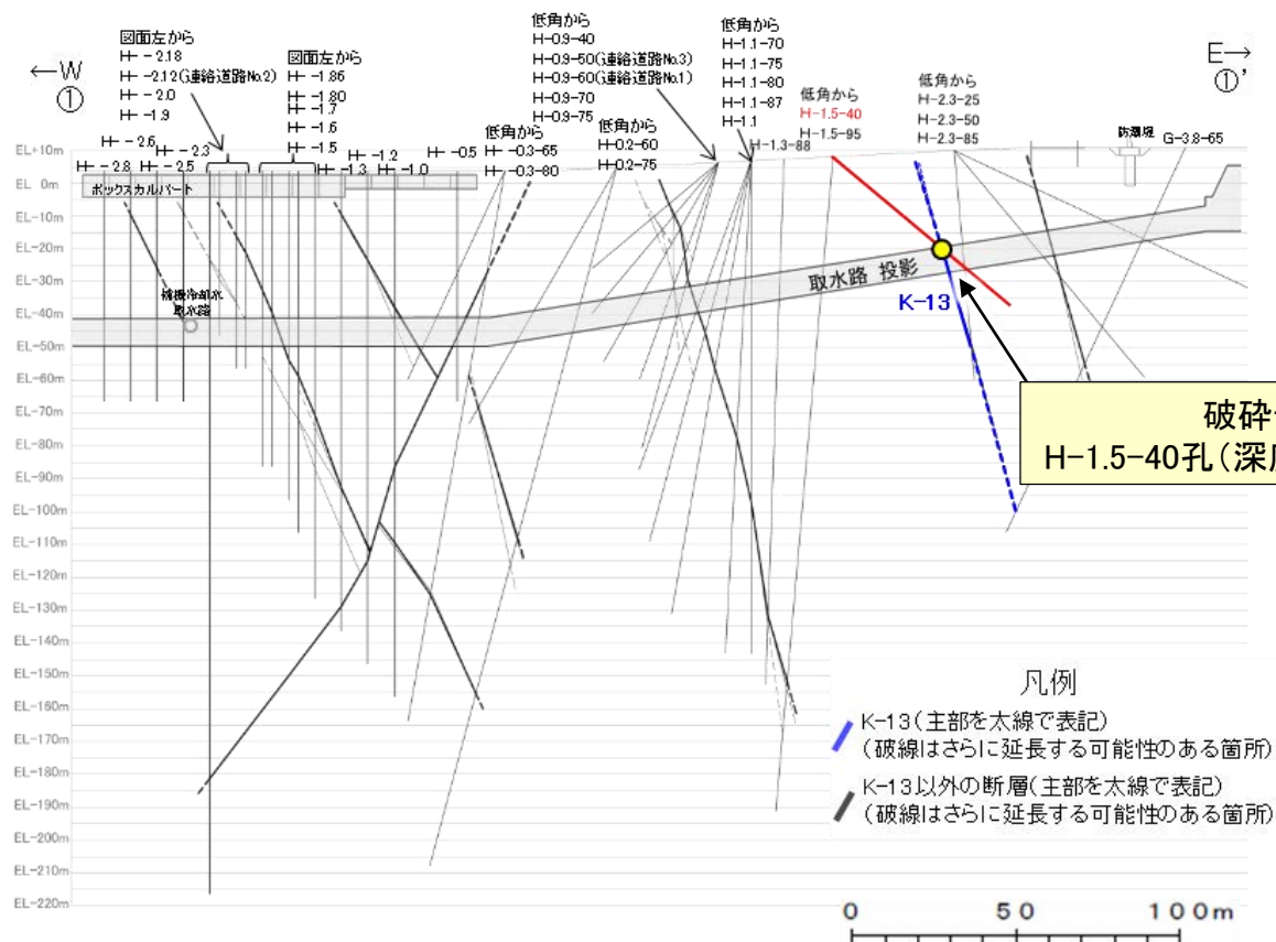
①-①'断面図
