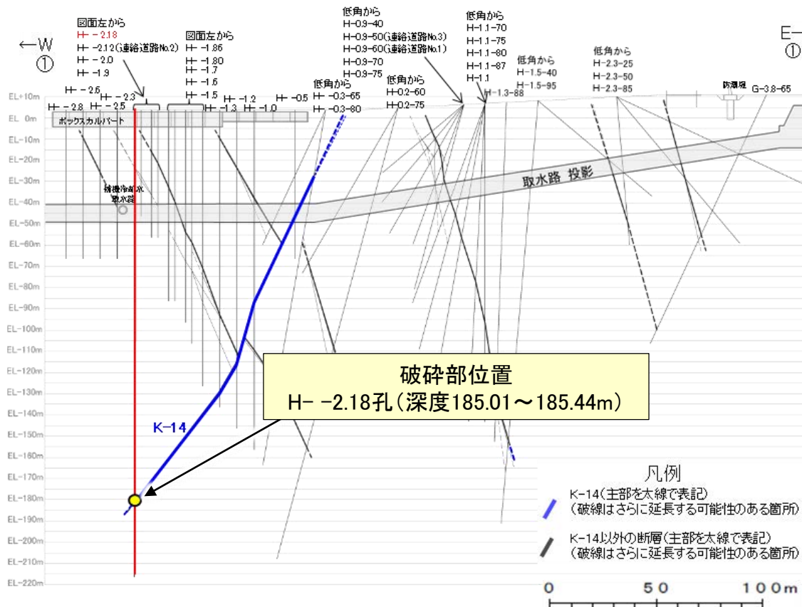
①-①' 断面図
