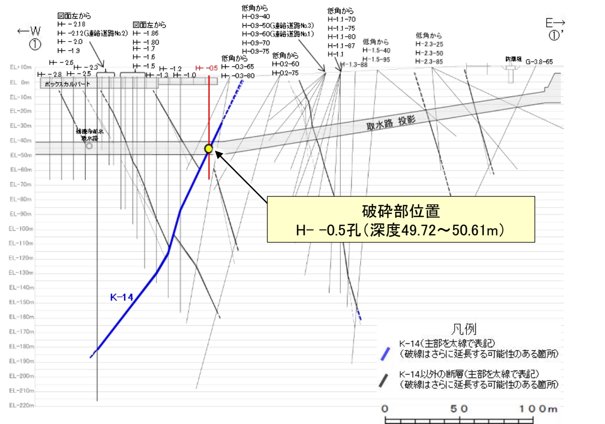
①-①' 断面図
