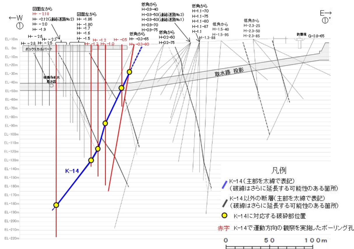
①-①' 断面図
