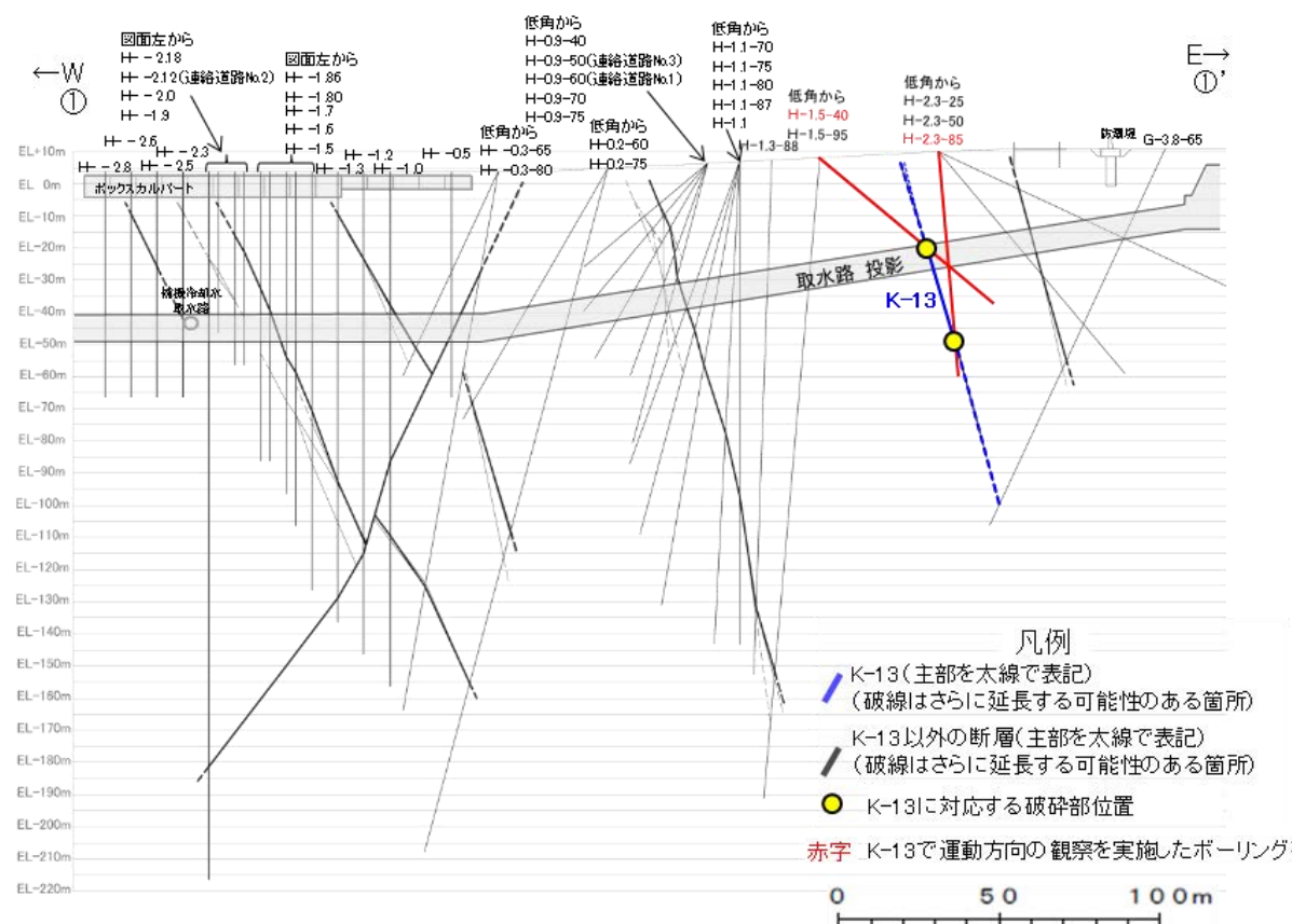
①-①' 断面図
