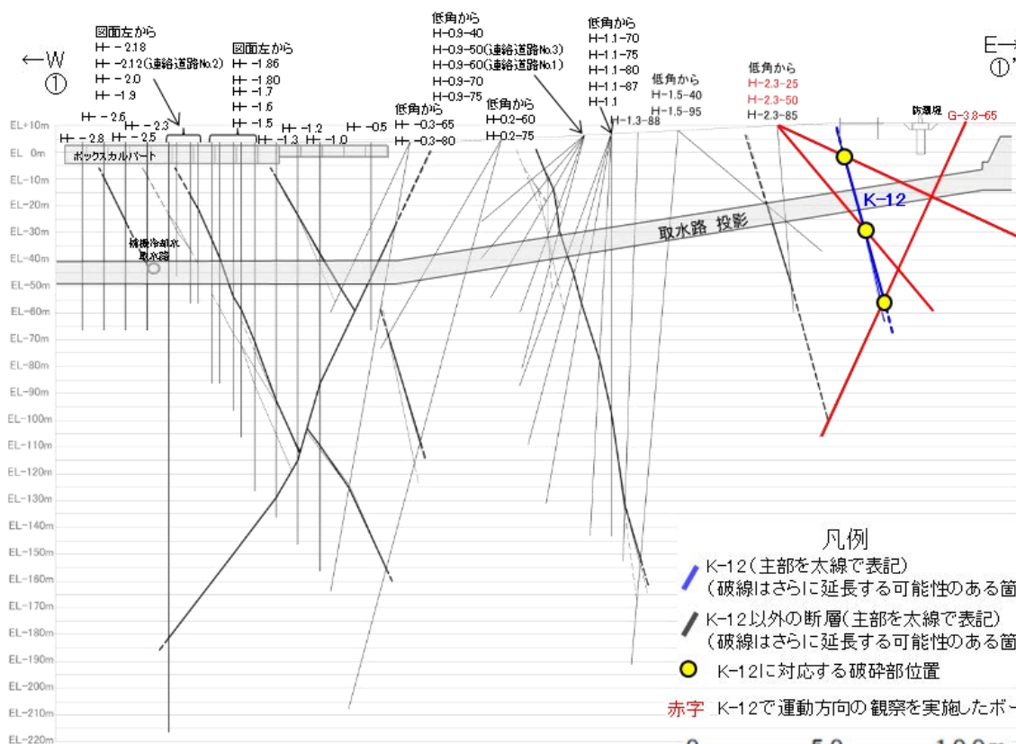
①-①' 断面図
