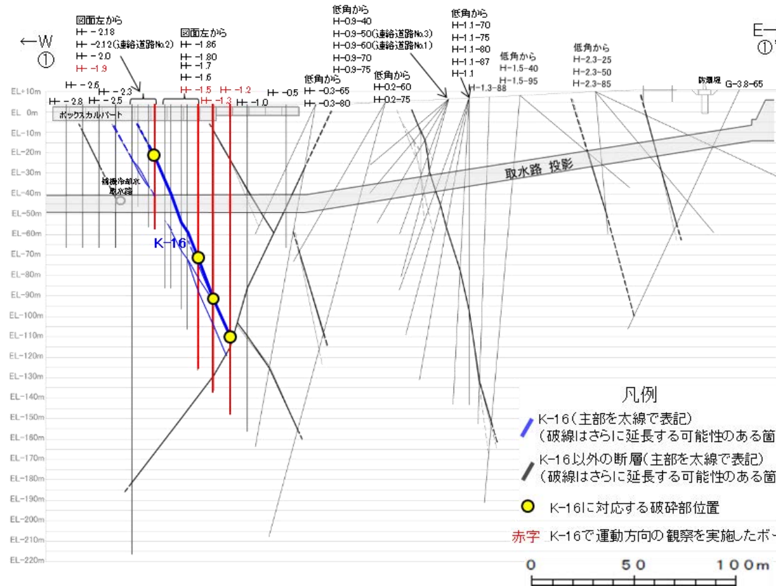
①-①' 断面図
