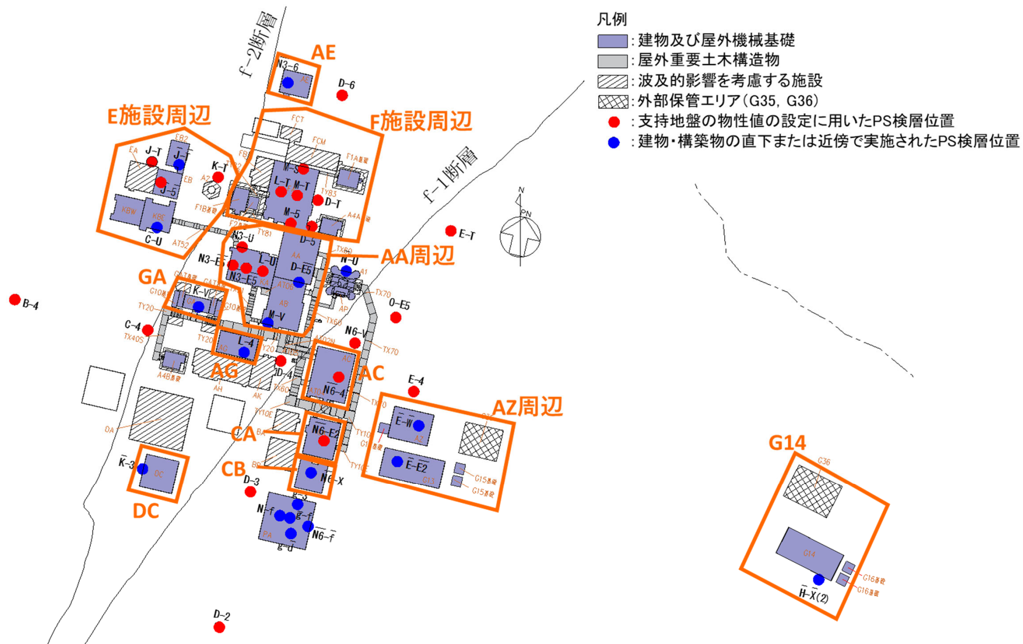
図 PS検層位置図
