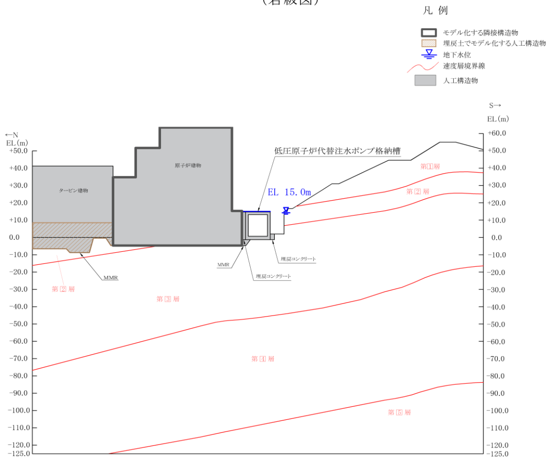
(岩級図)
