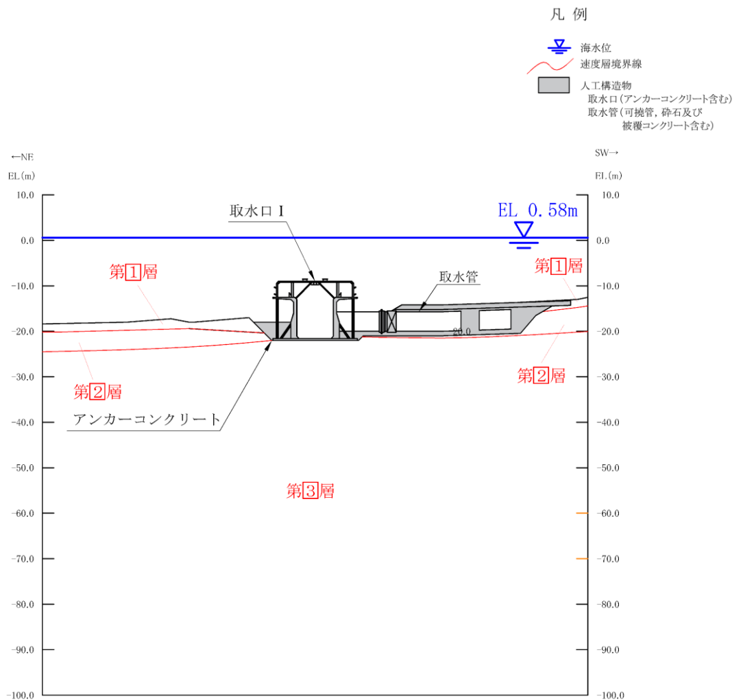
(速度層図)
