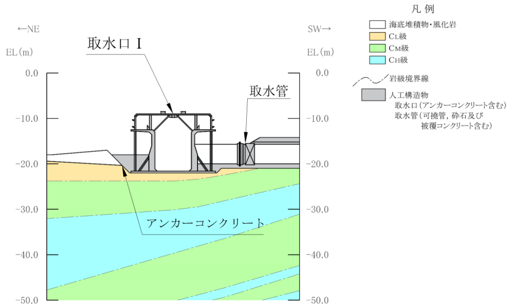
(岩級図)
