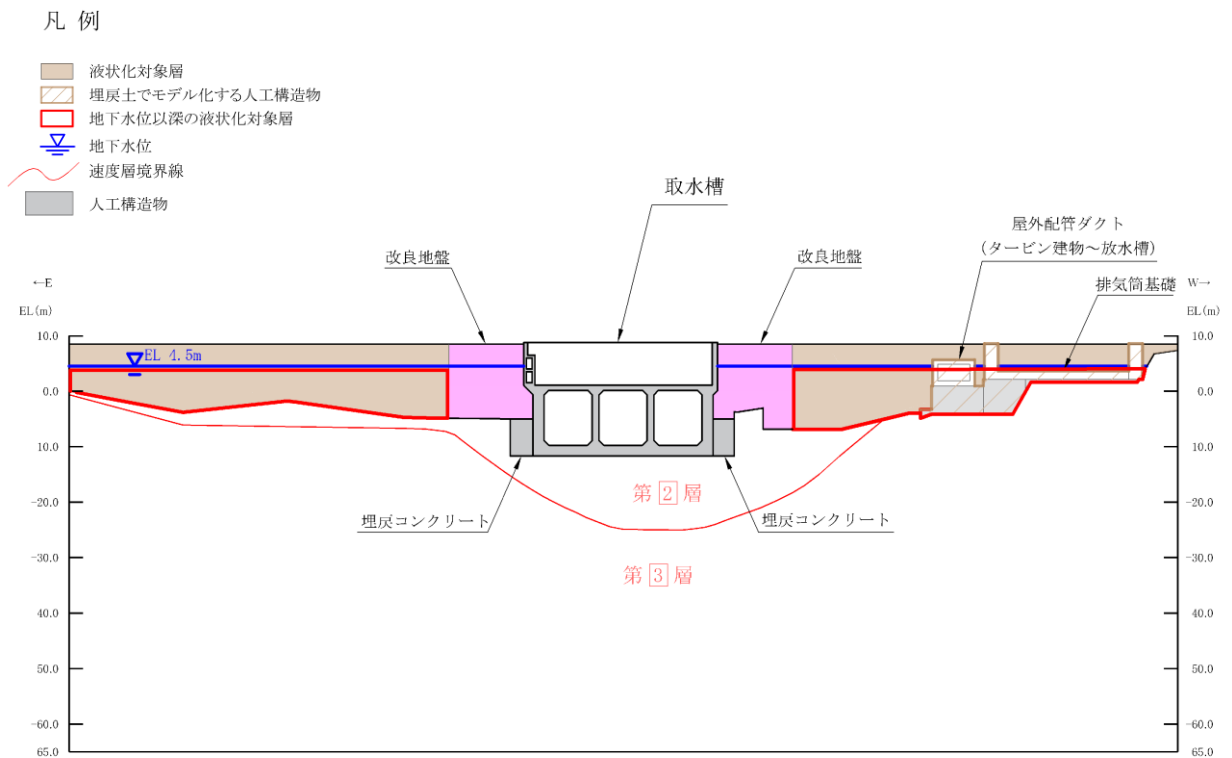
図 4.3-2(22) 取水槽【B-B断面】 地質断面図 (⑤有効応力解析)
