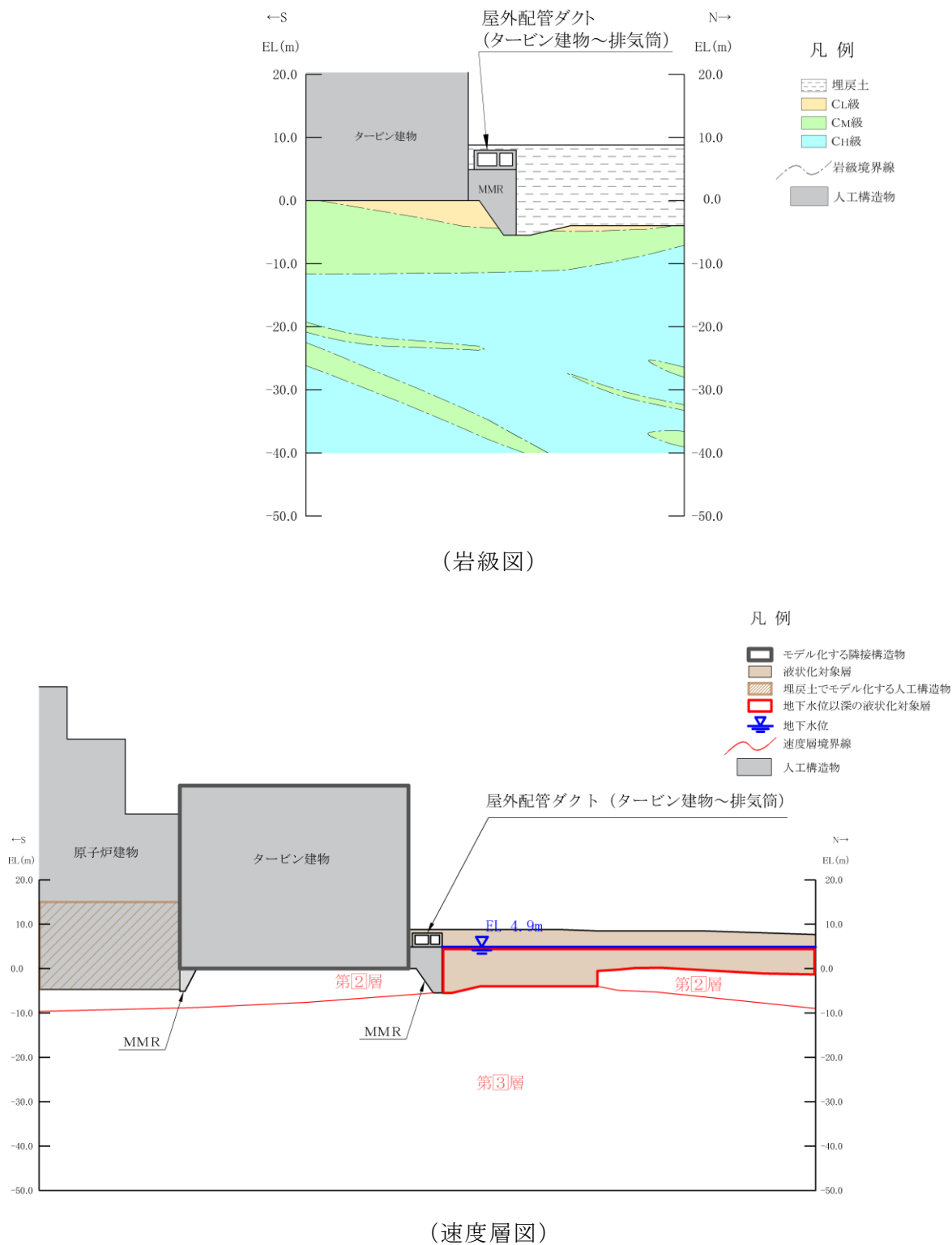
図 4.5-5(1) 屋外配管ダクト (タービン建物～排気筒) 地質断面図 (A-A断面)
