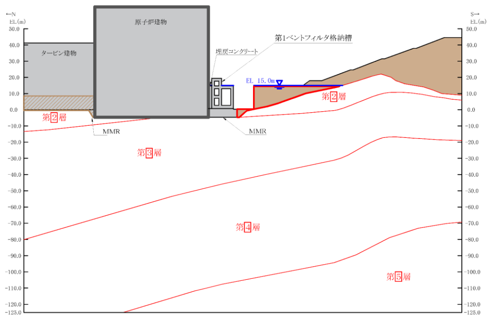
(速度層図)
