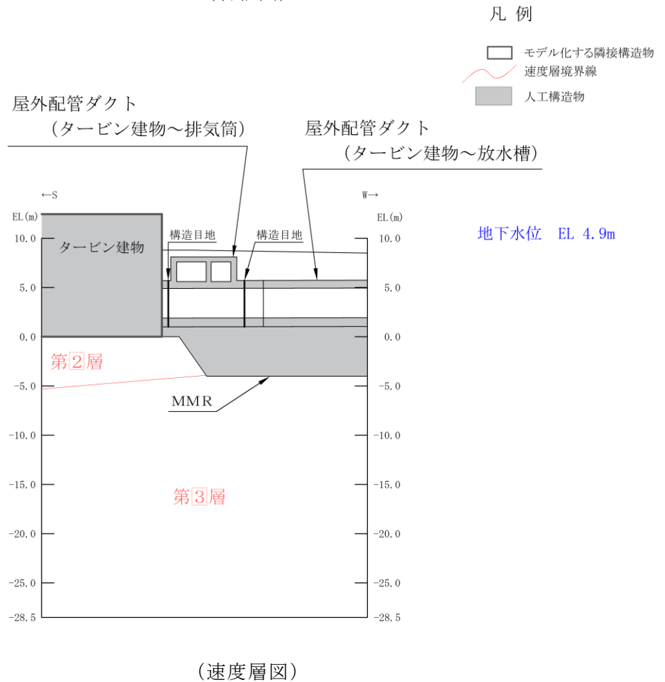
図 4.5-5(2) 屋外配管ダクト (タービン建物～排気筒) 地質断面図 (B-B断面)
