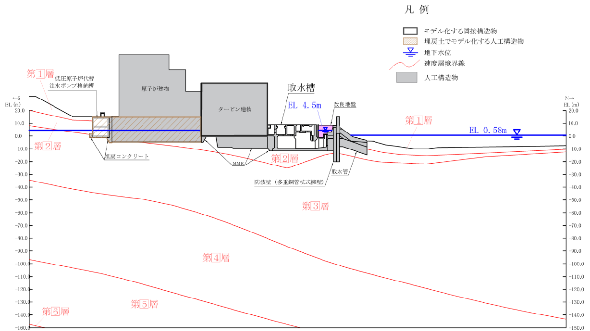
図 4.3-2(6) 取水槽 【D-D断面】 地質断面図 (②全応力解析)
