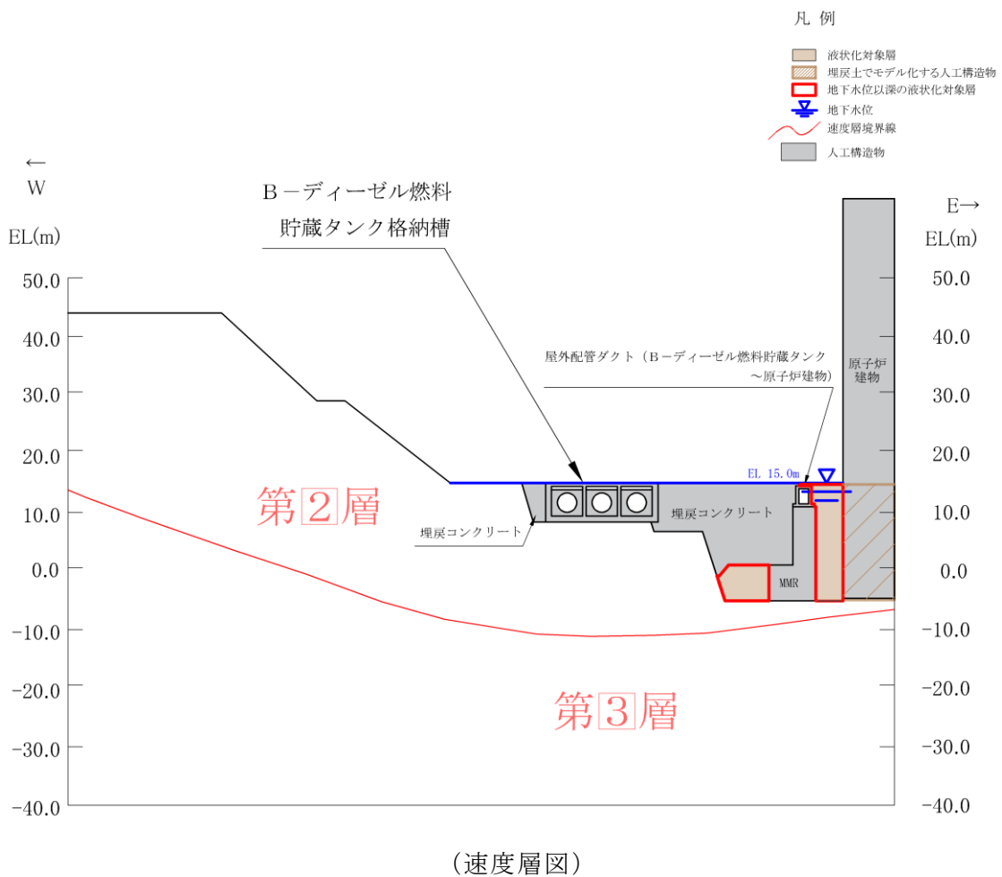
図 4.6-4 (1) B-ディーゼル燃料貯蔵タンク格納槽 地質断面図 (A-A断面)
