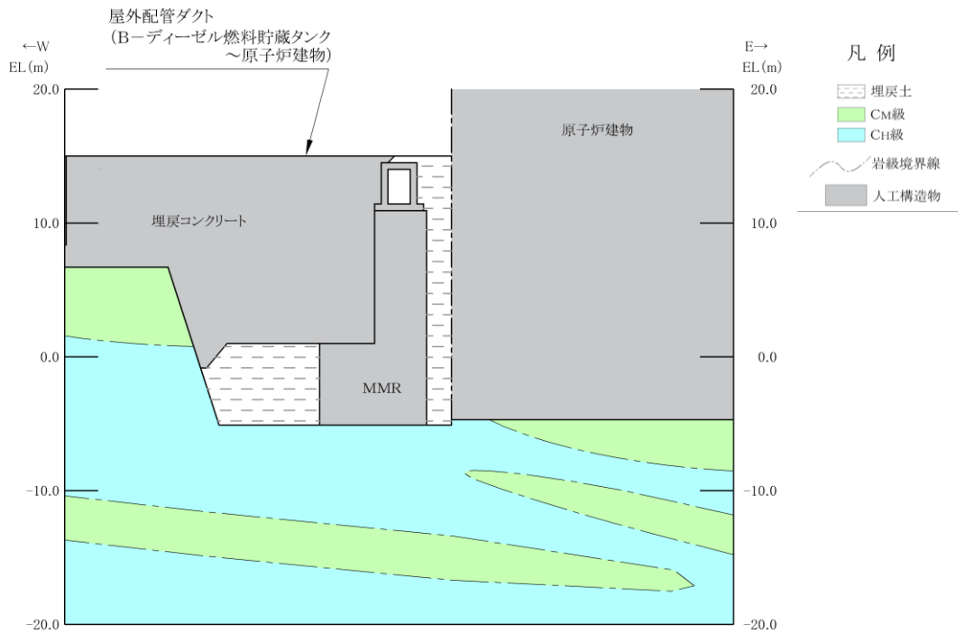
(岩級図)
