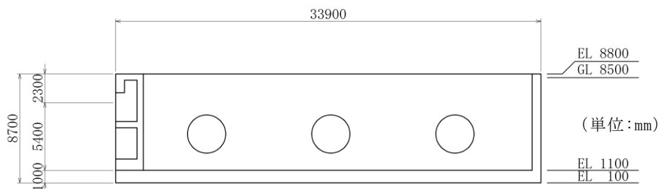
图 11.2-4 取水槽断面图(C-C断面)
