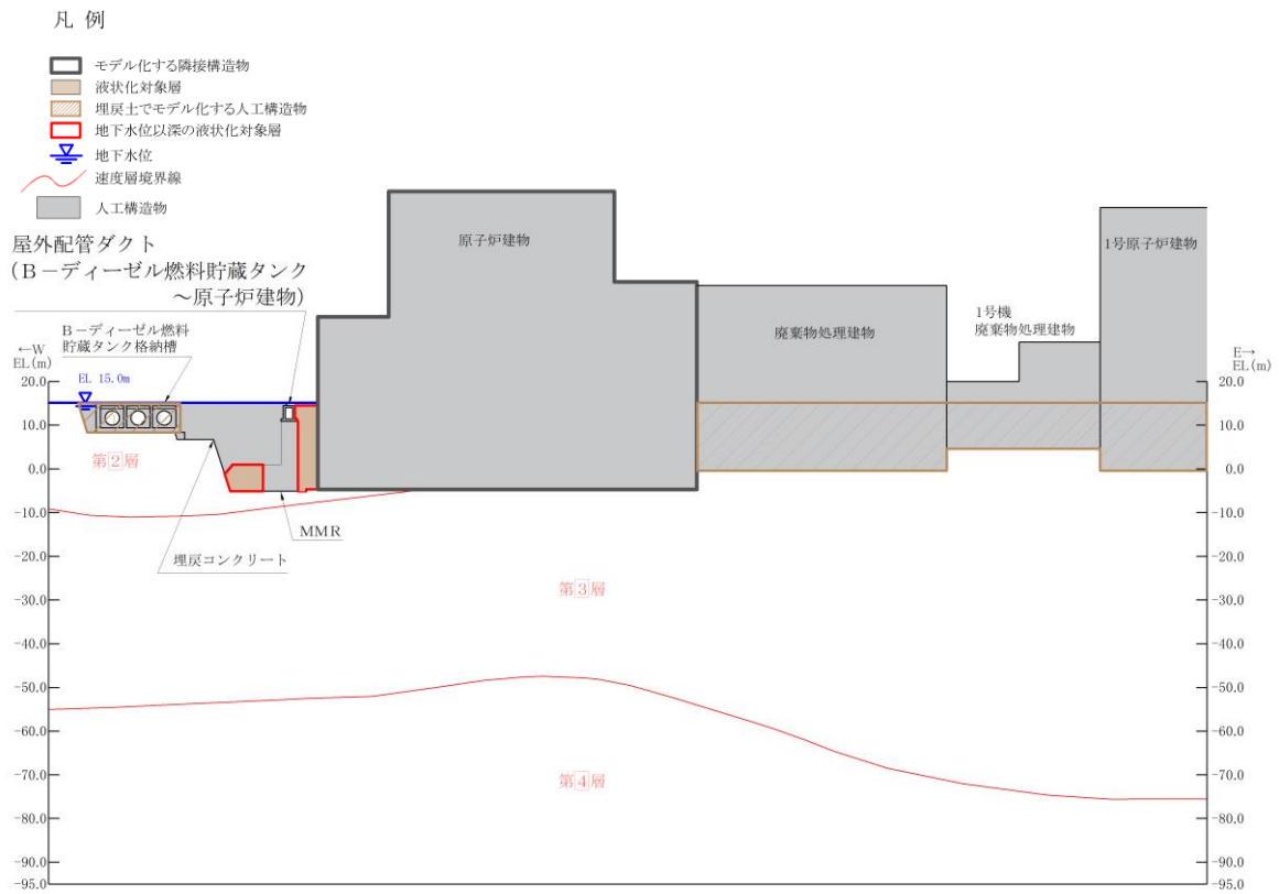
(速度層図)
