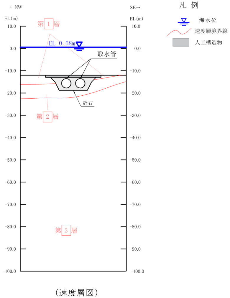
図 4.9-4 (2) 取水管 地質断面図 (E-E断面)
