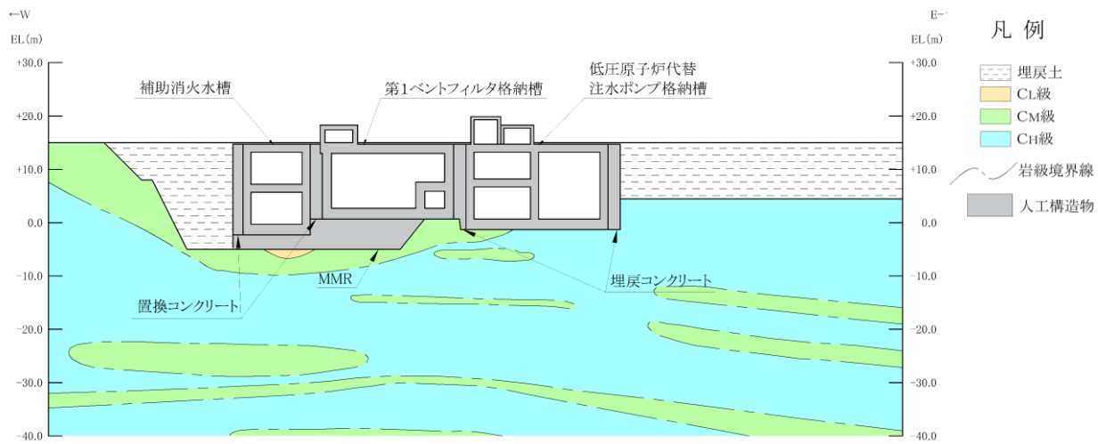
(岩級図)
