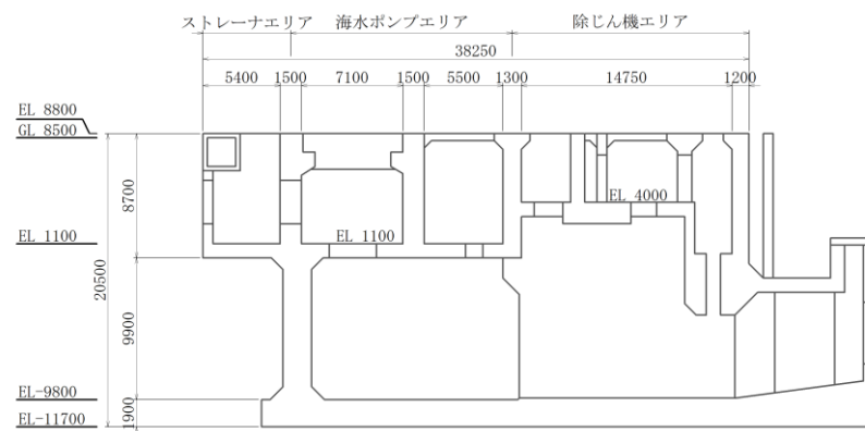
(D-D断面)
