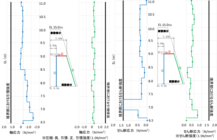
図23 境界部における引張応力図 図24 境界部におけるせん断応力図
