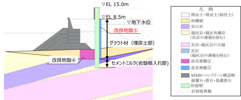
図2 断面図 (2-2断面)
