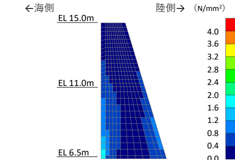
図15 コンクリートの最大せん断応力図
