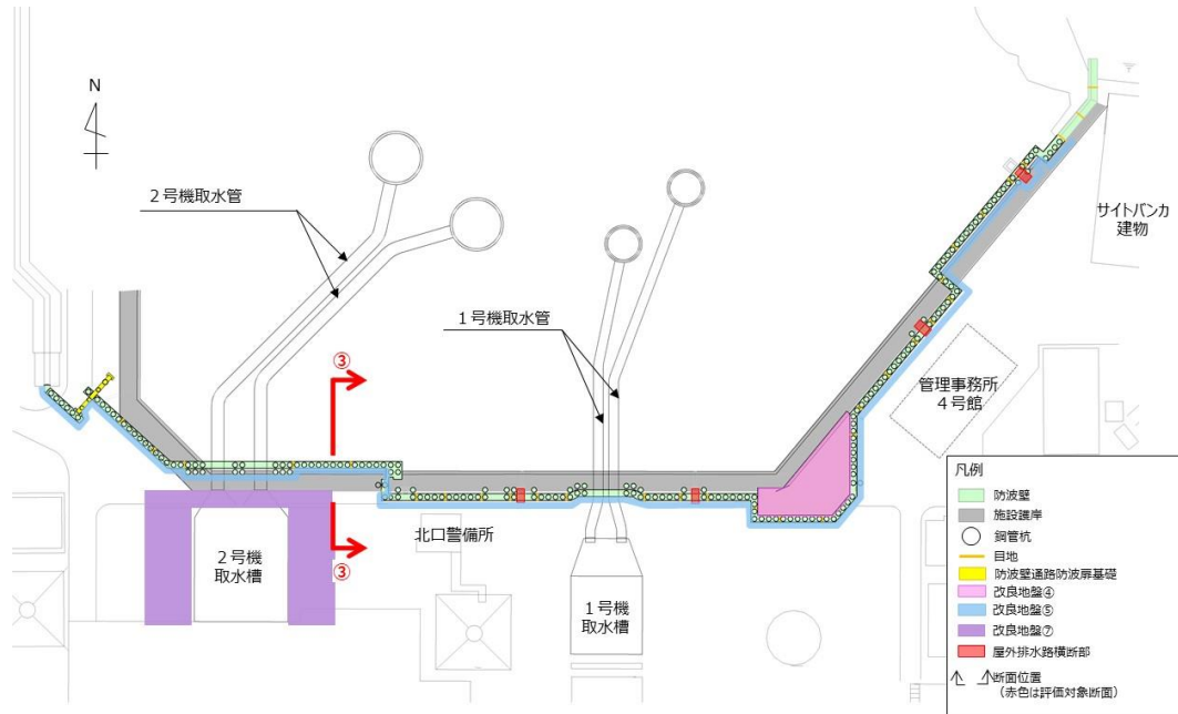
図1 平面図
