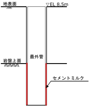
図7 セメントミルクの配置図
