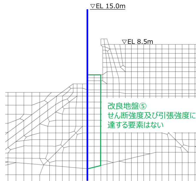
図6 改良地盤⑤の破壊履歴図 (例：③－③断面)
