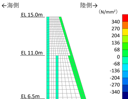
図16 鉄筋の応力図
