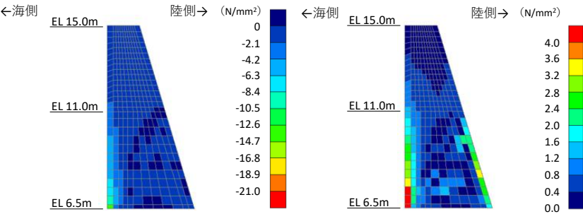
図20 コンクリートの最小主応力図 図21 コンクリートの最大せん断応力図
