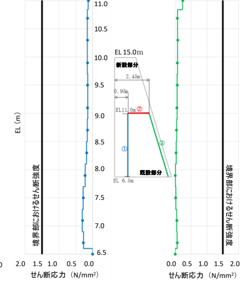
図18 境界部におけるせん断応力図
