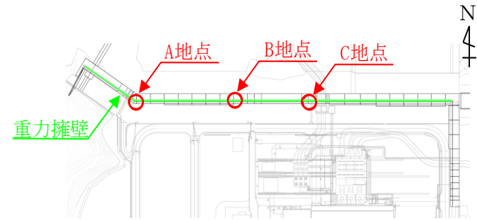
図5 付着強度試験実施位置図
