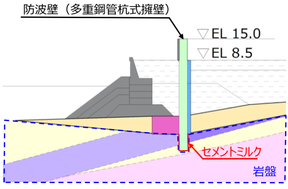
図8 解析モデル図
