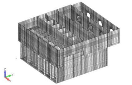
図11 3次元構造解析モデル図
