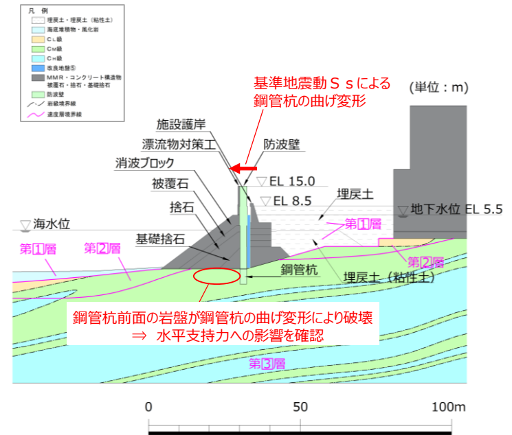
図2 断面図 (3-3断面)
