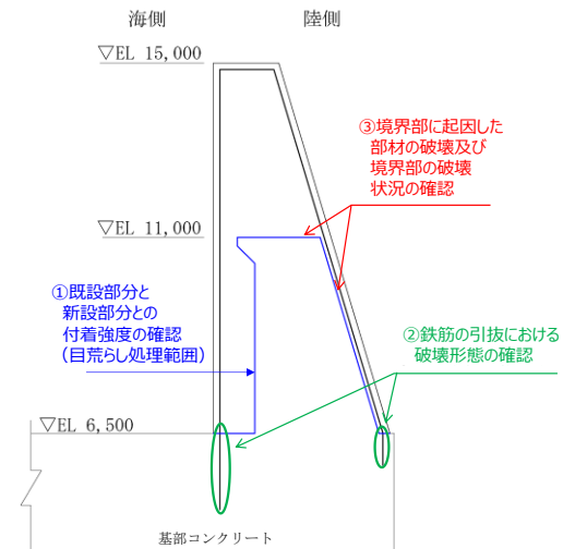
図2 一体性における確認事項
