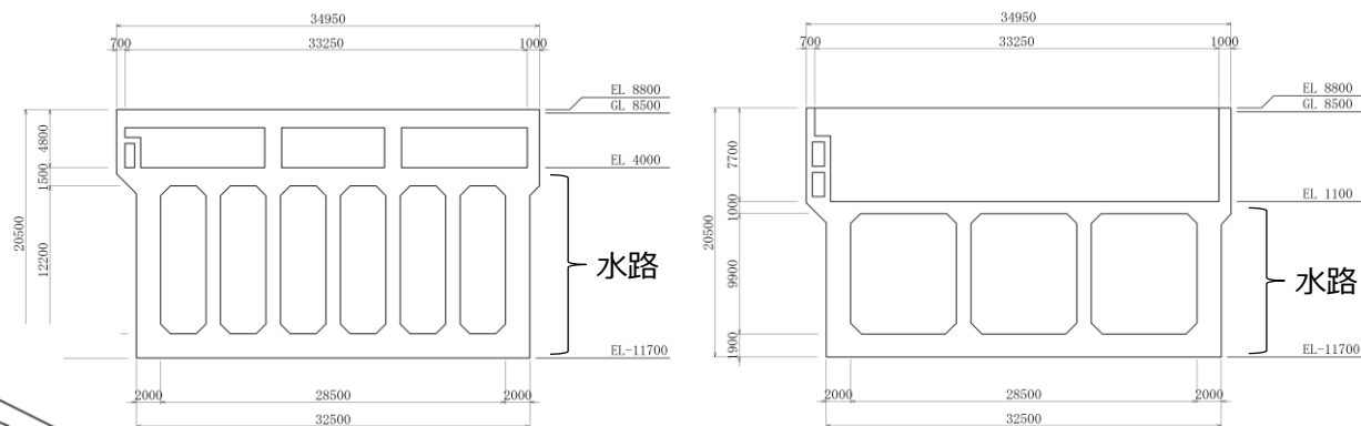
(A-A断面)
