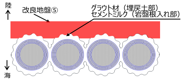
図3 地中断面図
