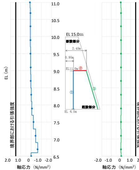
図17 境界部における引張応力図
