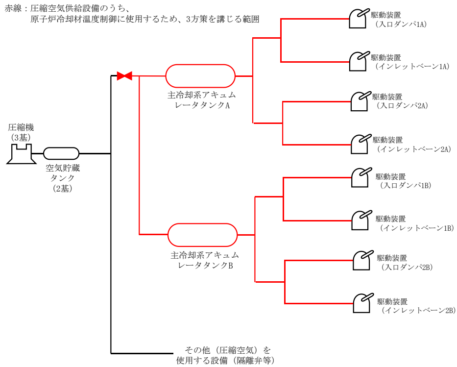
第 2.2 図 原子炉冷却材温度制御系に係る圧縮空気供給設備の概要
