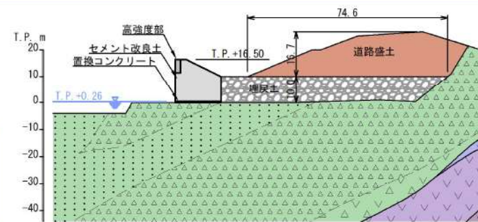
地質断面図(7-7')
