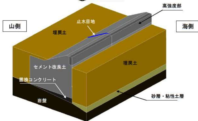
防潮堤(標準部)の構造概要
