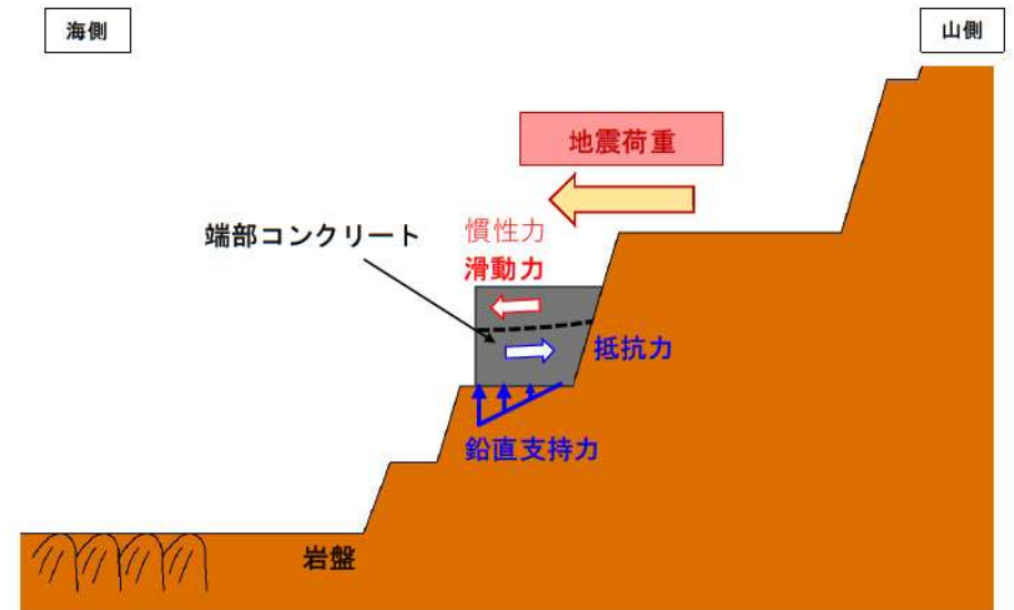
荷重図
