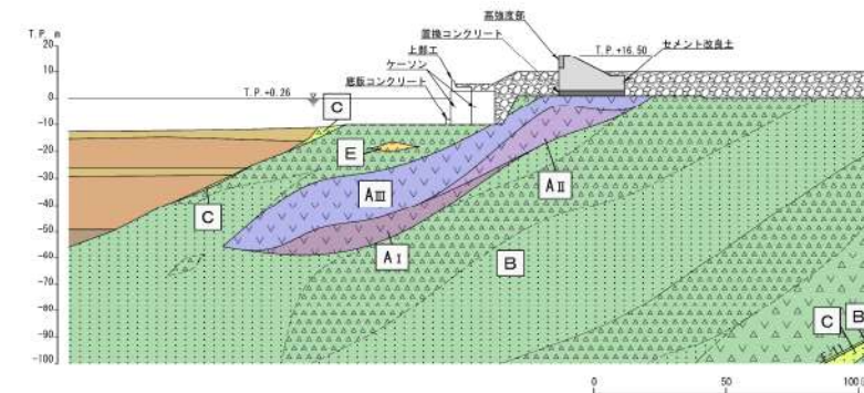
地質断面図 (4-4')
