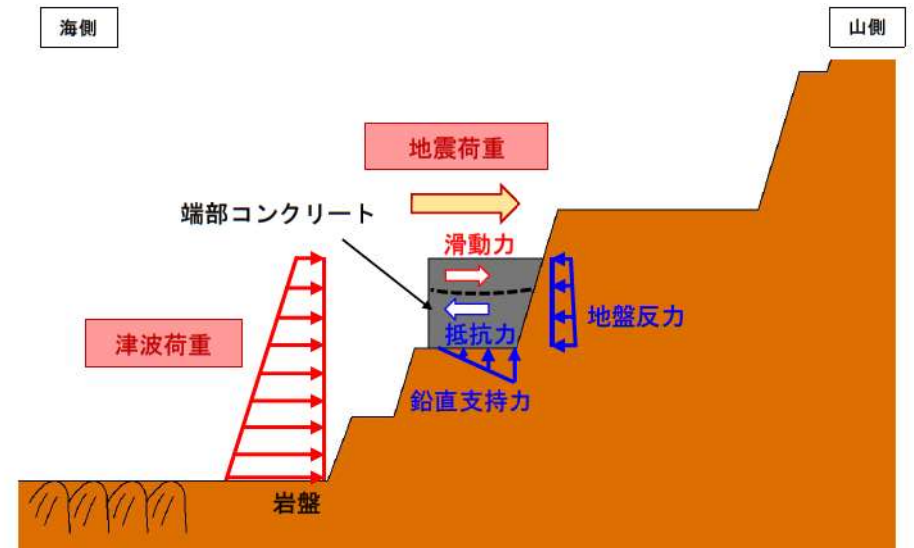
荷重図
