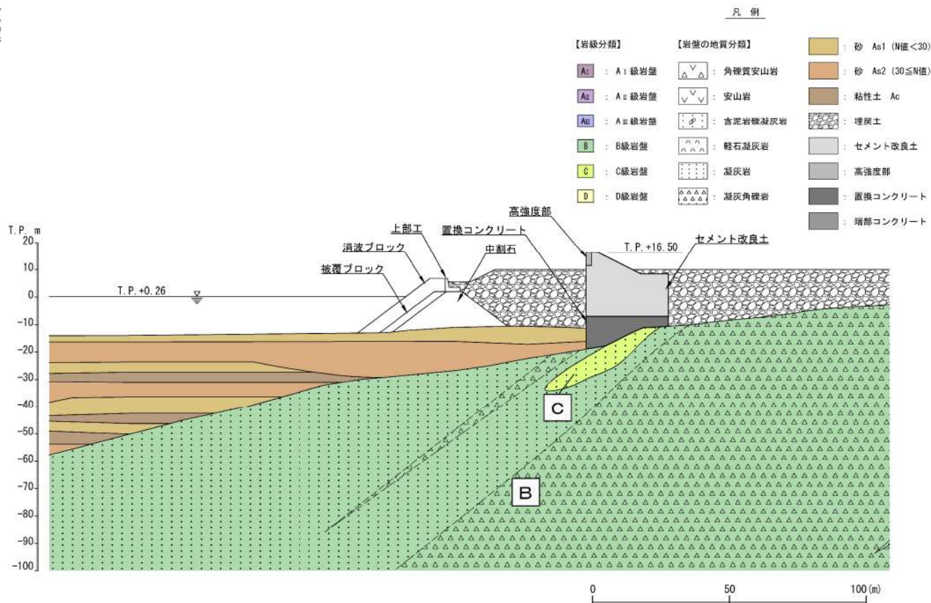
地質断面図 (2-2')
