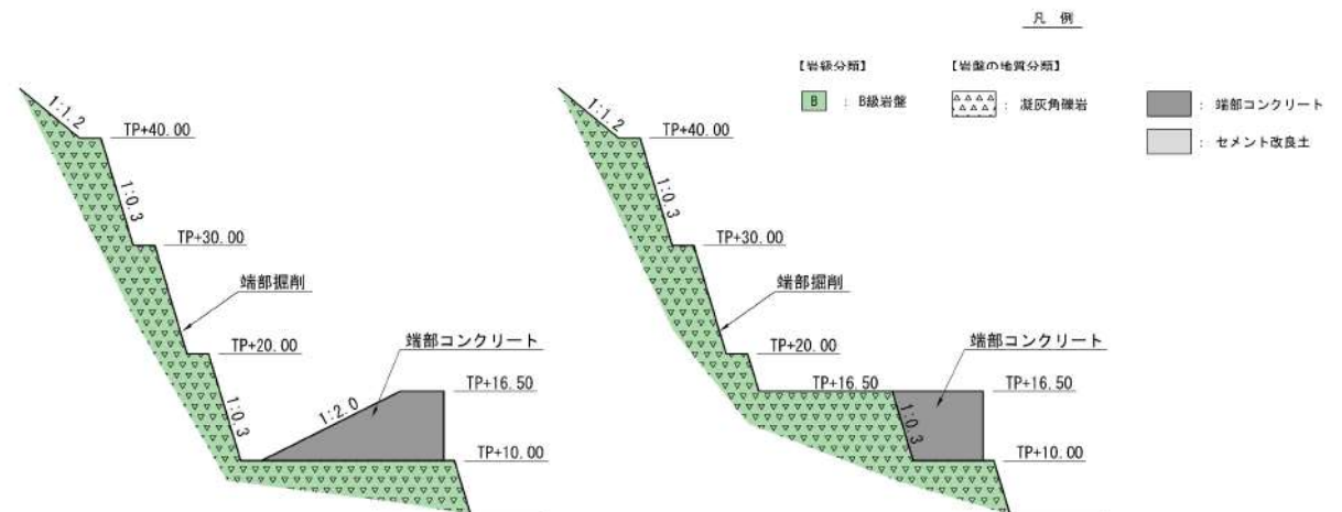
地質断面図
