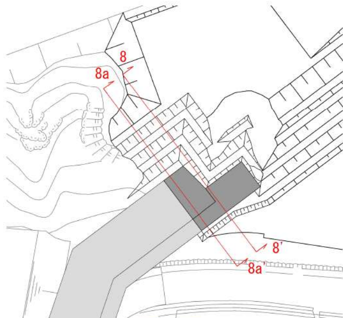
断面位置図
