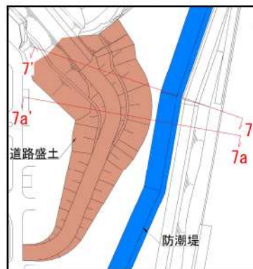
拡大図
