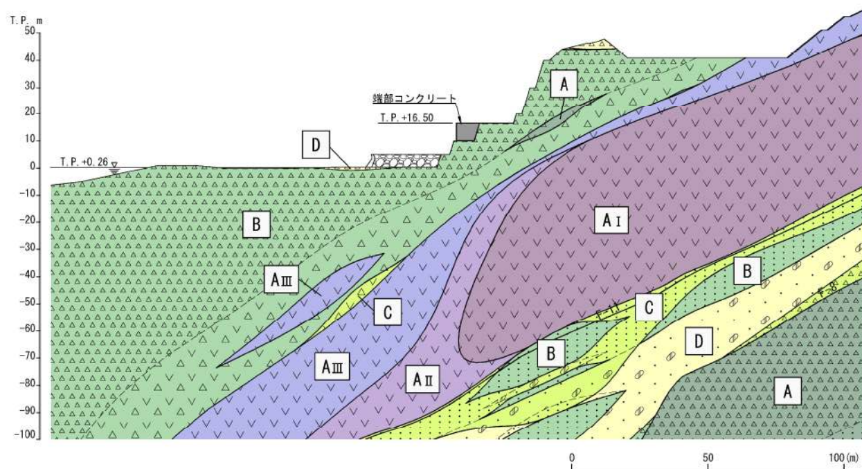
地質断面図 (8-8')
