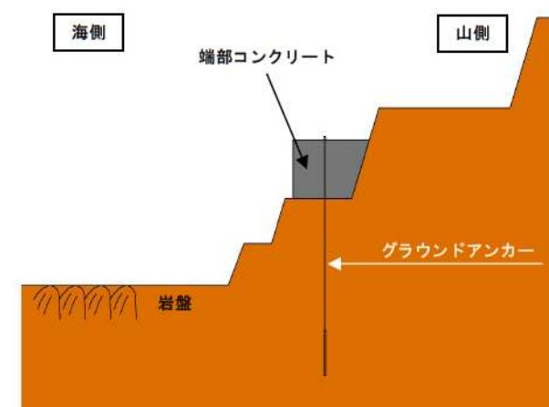
裕度向上対策後(対策イメージ図)
