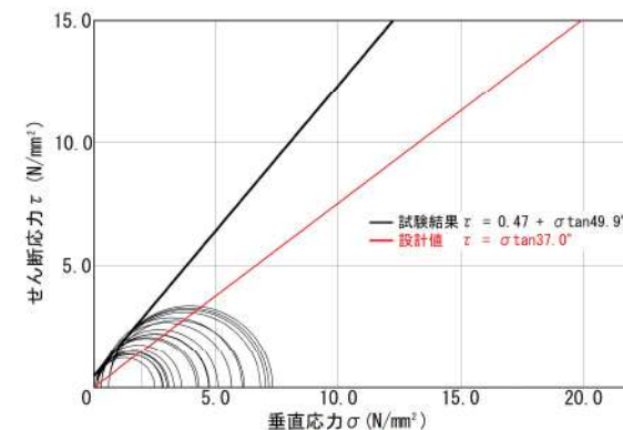
残留強度 三軸圧縮試験結果
