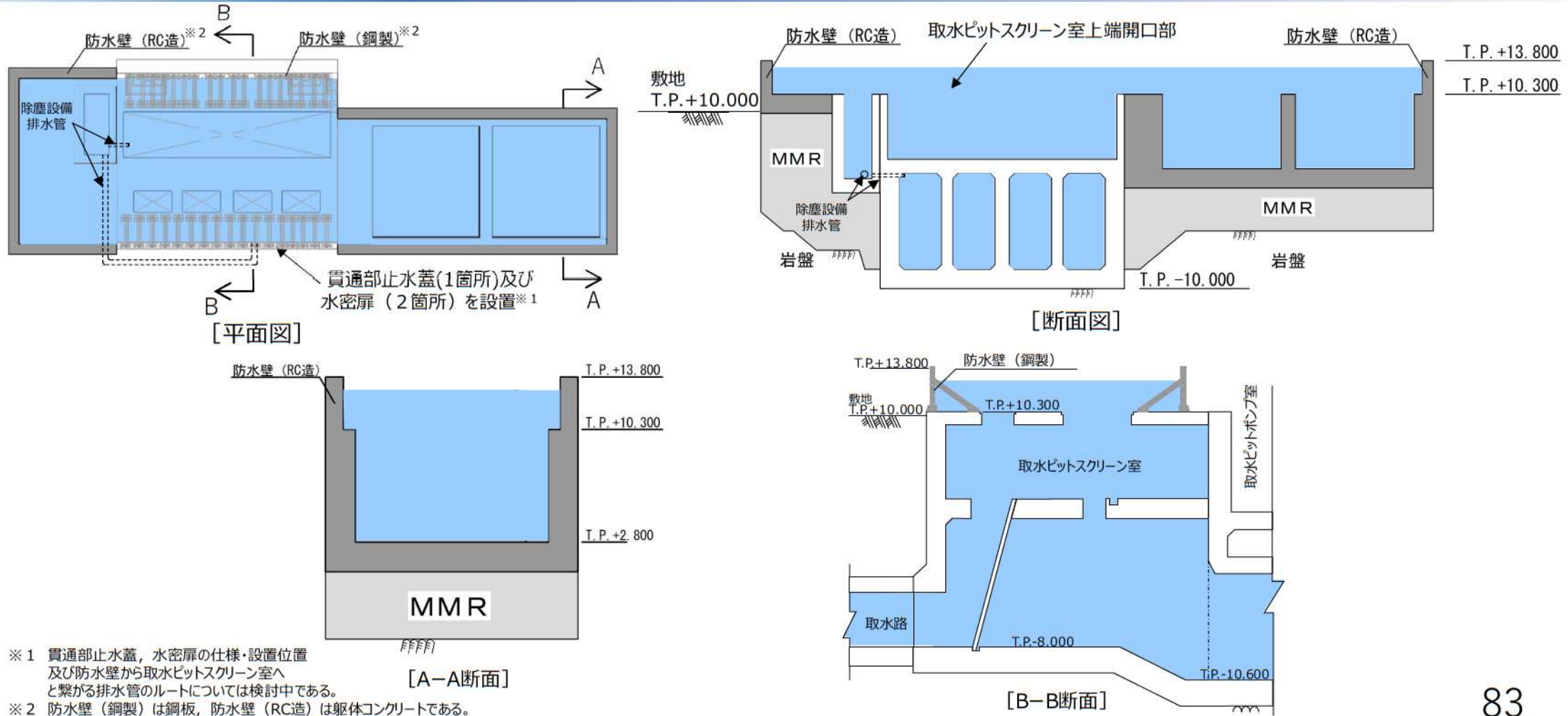
図2 3号炉取水ピットスクリーン室防水壁構造概要図
