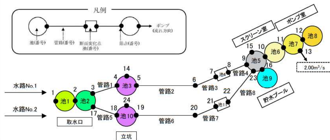
【3号炉取水路モデル図】
