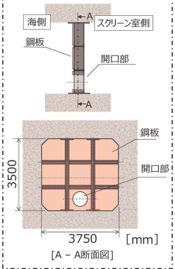
a部詳細図 (1号及び2号炉取水路流路縮小工)
