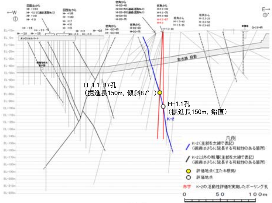
①-①' 断面図
