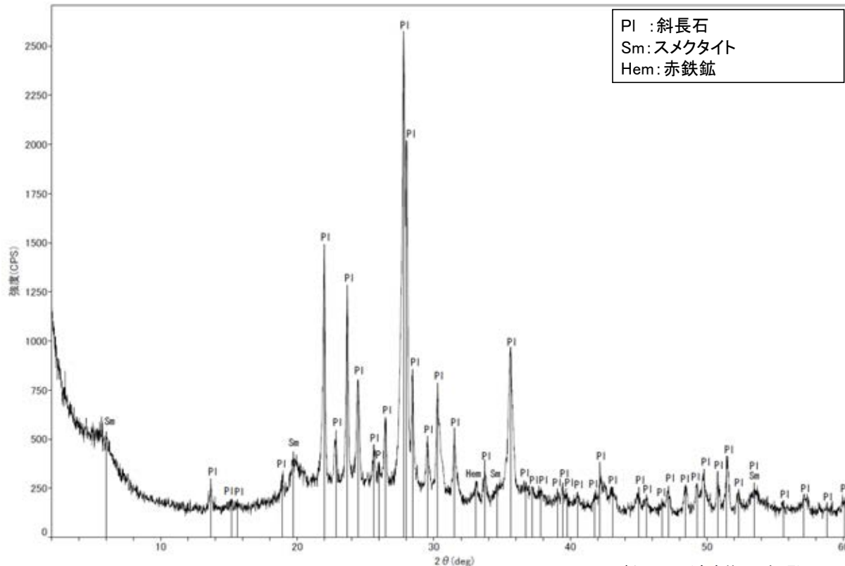
回折チャート(不定方位)_R-8.1-1-2孔 補足資料5.3-3(1) P.5.3-27
