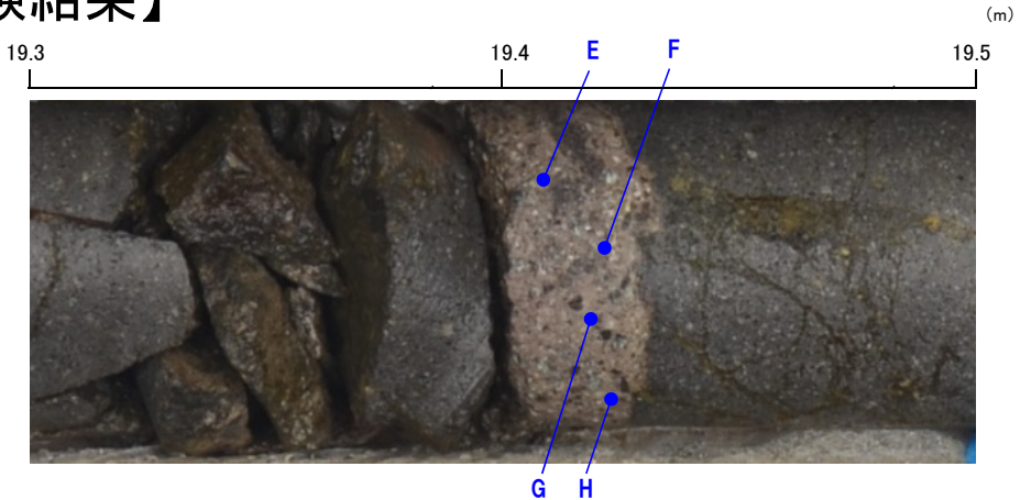
針貫入試験実施位置(M-2.2-2孔)
