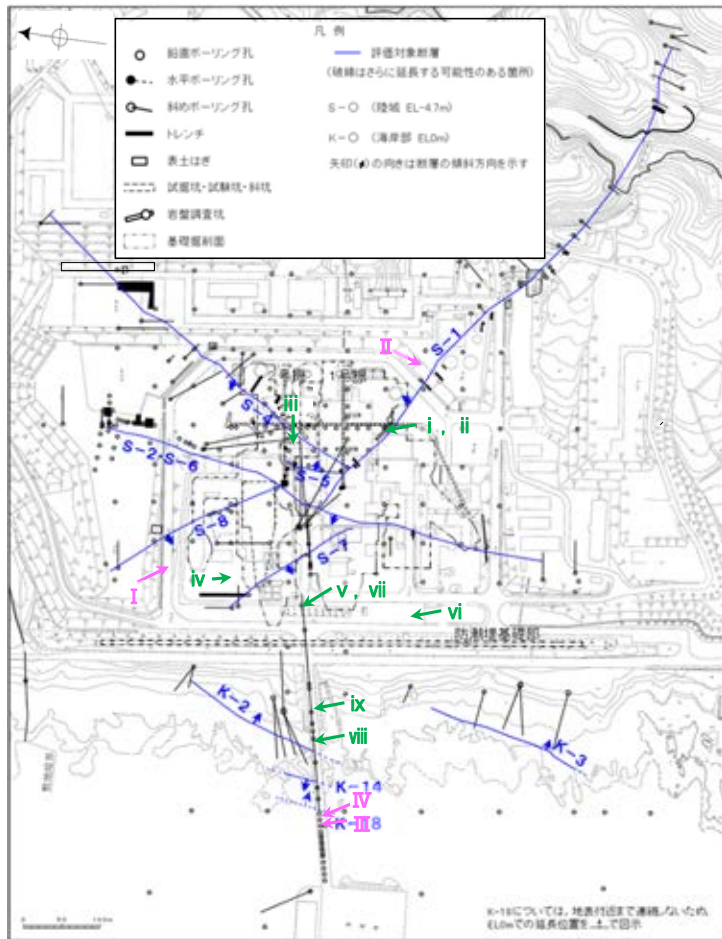
試料採取位置図 緑色矢印 白色鉱物(オパールCT)分析試料 桃色矢印 白色鉱物(フィリップサイト)分析試料
