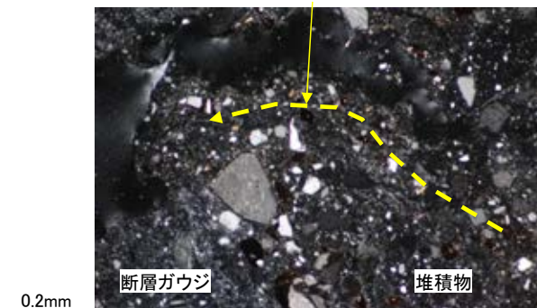
薄片写真(阿寺断層の事例)
