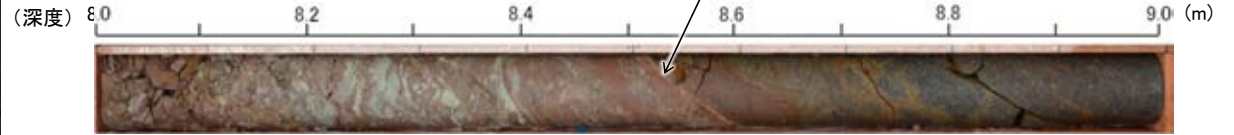
破碎部中に粘土鉱物が認められる事例 (試料D, E-8.5-2孔 深度8.55m付近)
