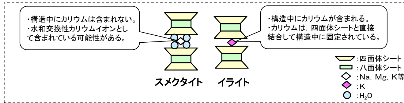
ス멕タイトとイライトの構造とその特徴 (吉村(2001)を基に作成)
