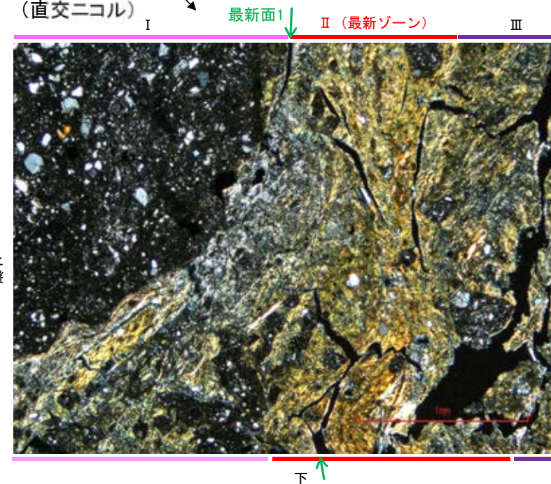
(直交ニコル)
