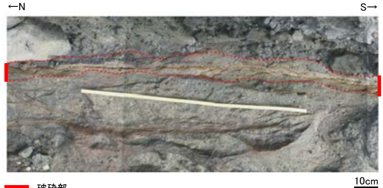
K-3 露頭a地点 破碎部の状況写真
