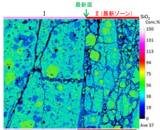
SiO 2
