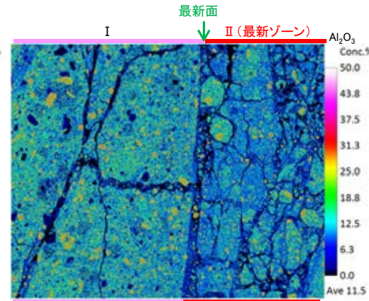
Al 2 O 3
