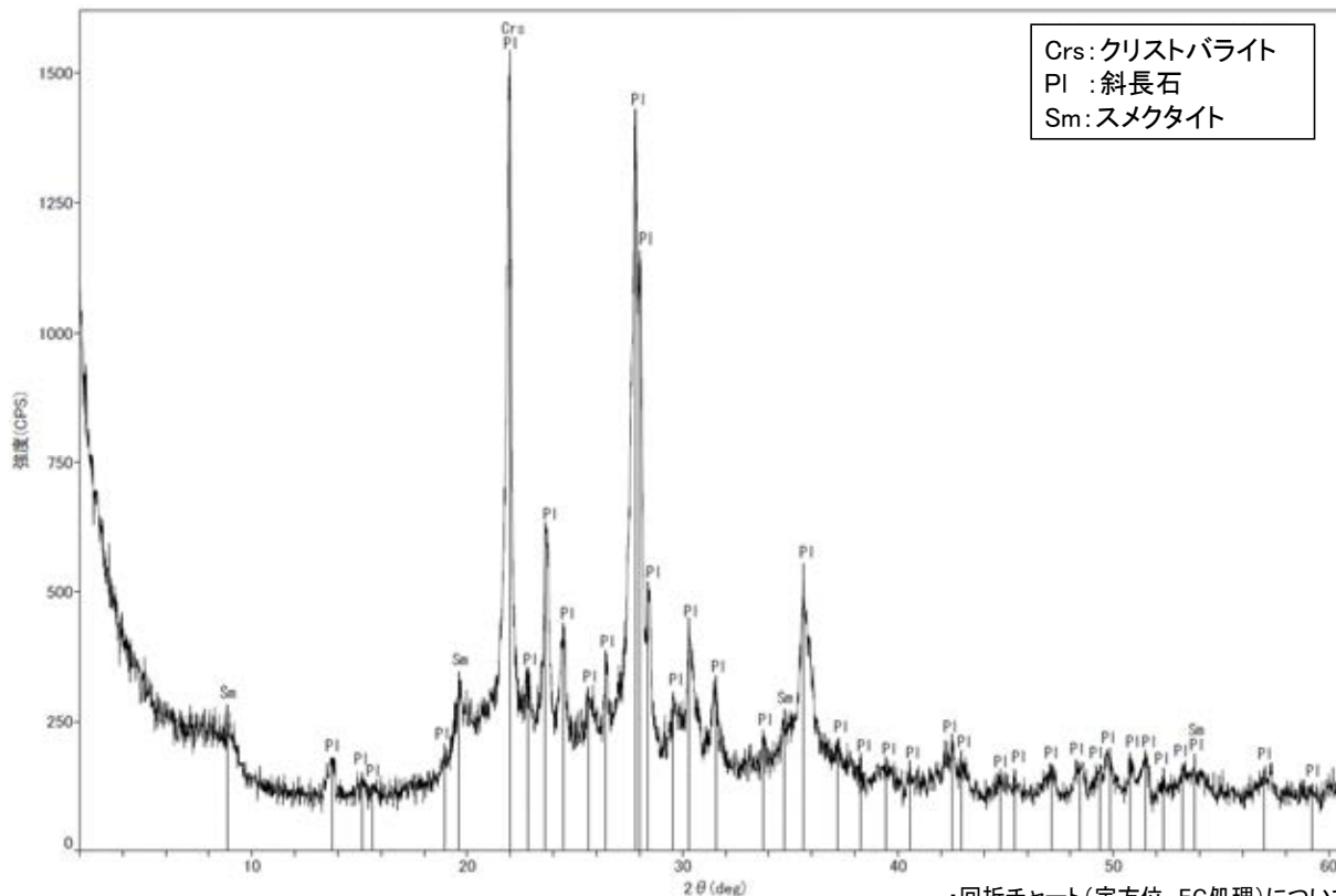
回折チャート(不定方位)_H-1.1-87孔 回折チャート(定方位, EG処理)については, 補足資料5.3-3(1) P.5.3-3-37
