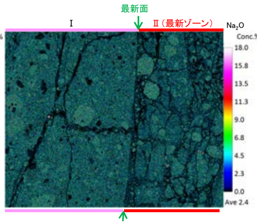
Na 2 O
