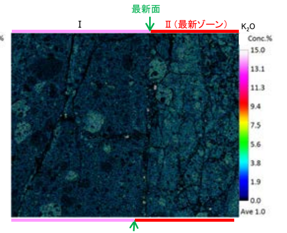
K 2 O
