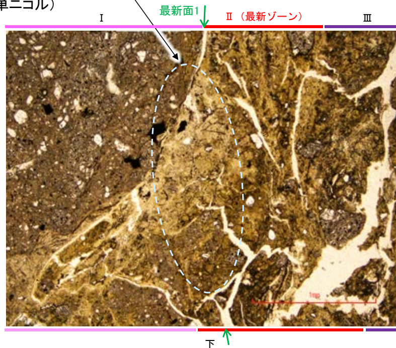
(単ニコル)
