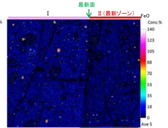
FeO
