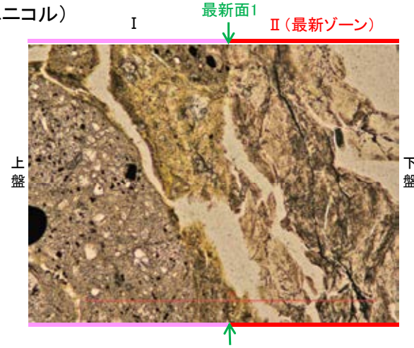
上盤 下盤
