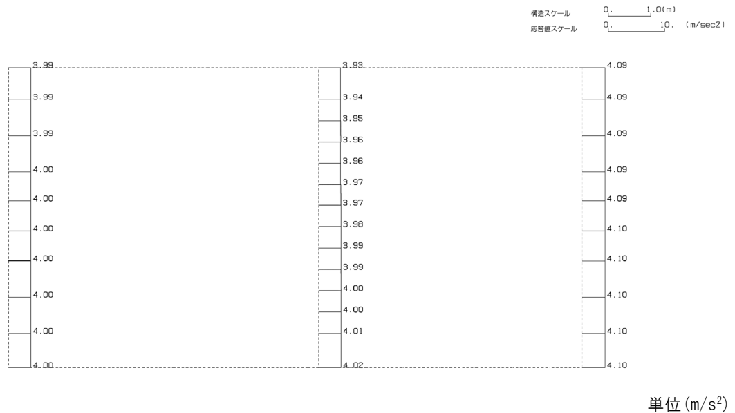
第4-4図 d-d断面の最大加速度分布図(Ss-A) (1/13)
