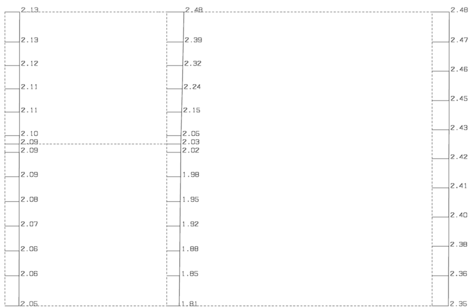
第 4-8 図 F-F 断面の最大加速度分布図 (Ss-C1) (7/13)
