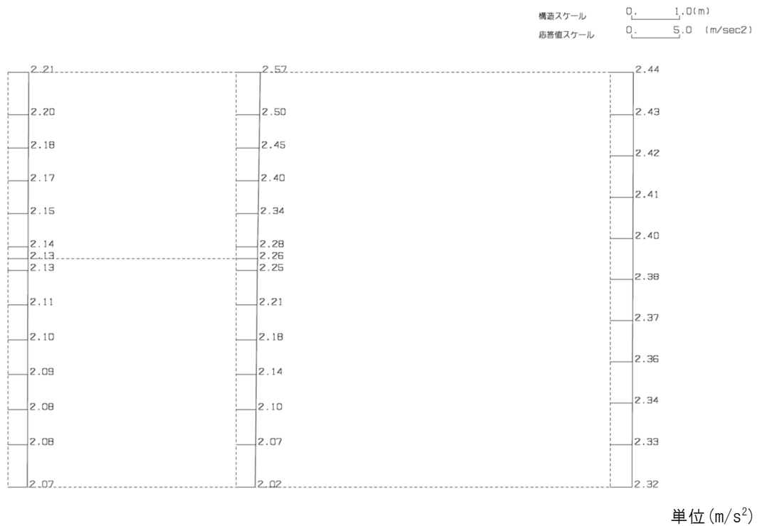
第 4-8 図 F-F 断面の最大加速度分布図 (Ss-C3 (NS)) (10/13)
