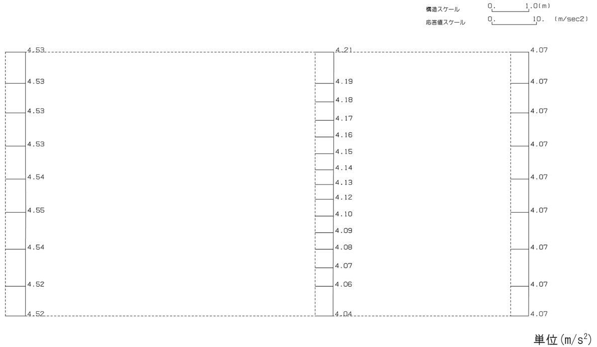
第 4-8 図 f-f 断面の最大加速度分布図(Ss-B3) (4/13)
