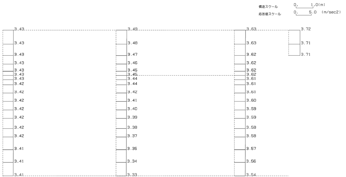
第 4-2 図 c-c 断面の最大加速度分布図 (Ss-B1) (2/13)
