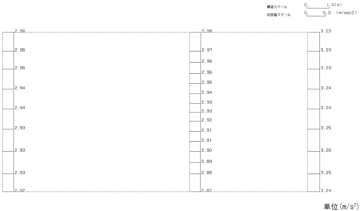
第 4-8 図 f-f 断面の最大加速度分布図 (Ss-B4) (5/13)
