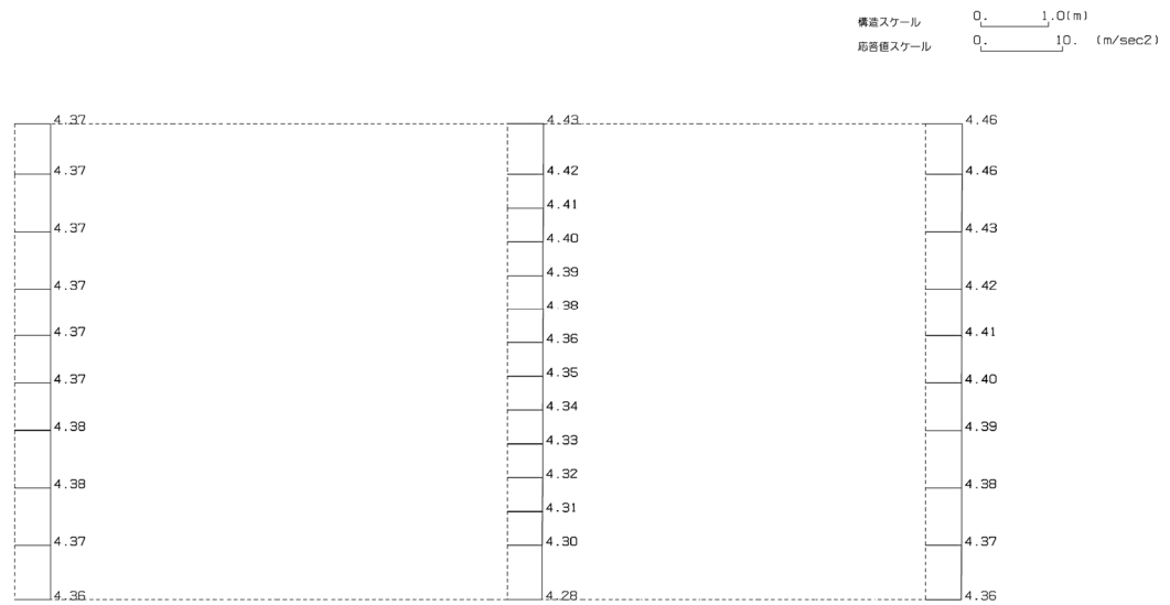
第 4-4 図 d-d 断面の最大加速度分布図 (Ss-B3) (4/13)
