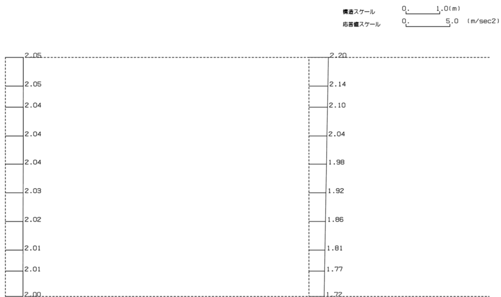
第 4-2 図 C-C 断面の最大加速度分布図 (Ss-C1) (7/13)
