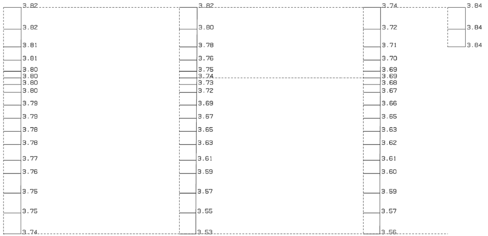
第 4-2 図 c-c 断面の最大加速度分布図 (Ss-B5) (6/13)
