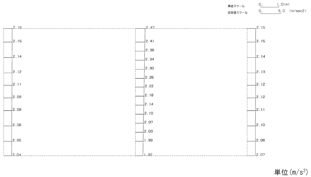
第 4-4 図 d-d 断面の最大加速度分布図 (Ss-C1) (7/13)
