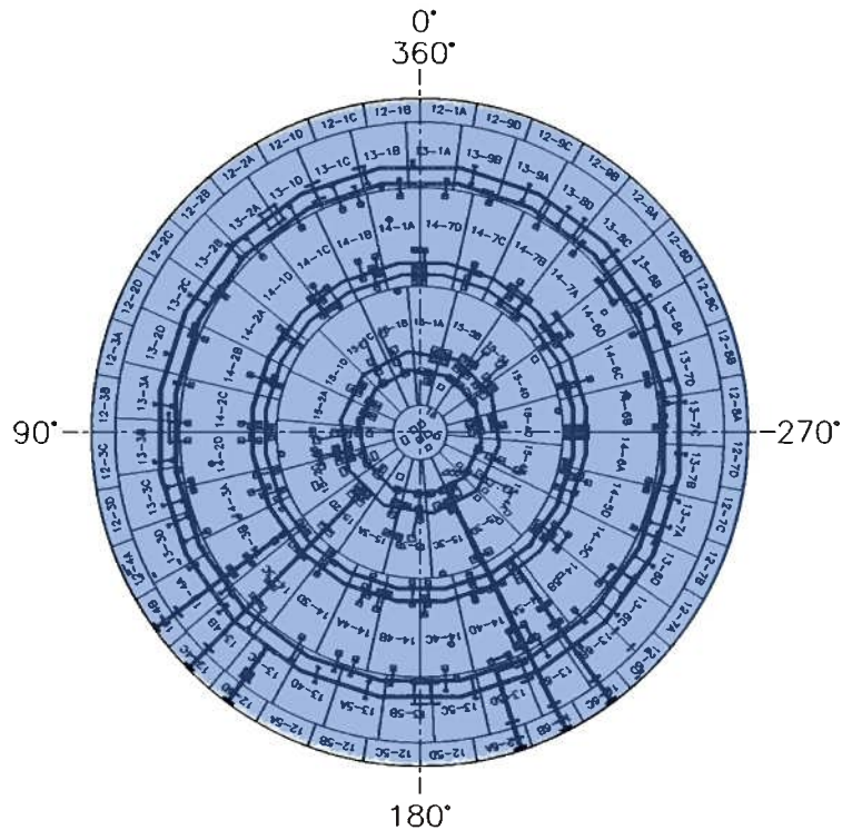
図3.5.1 半球部内面
