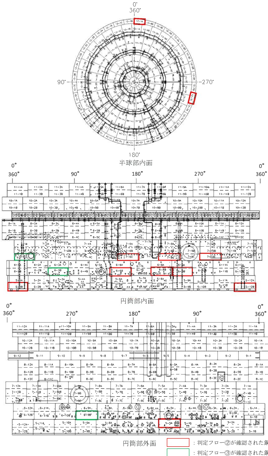
図5. 3. 1 軽微な劣化が確認された鋼板
