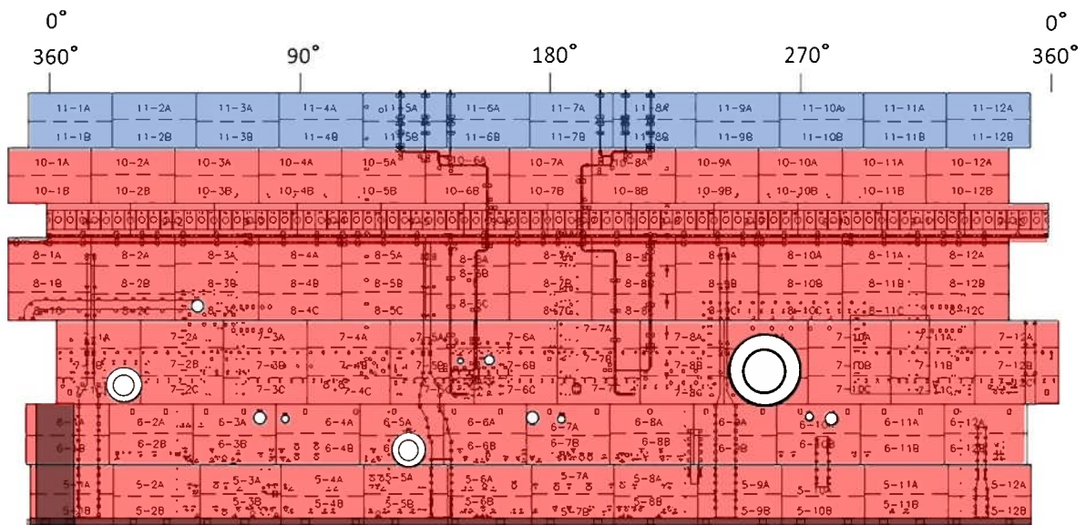
図3.5.3 円筒部内面
