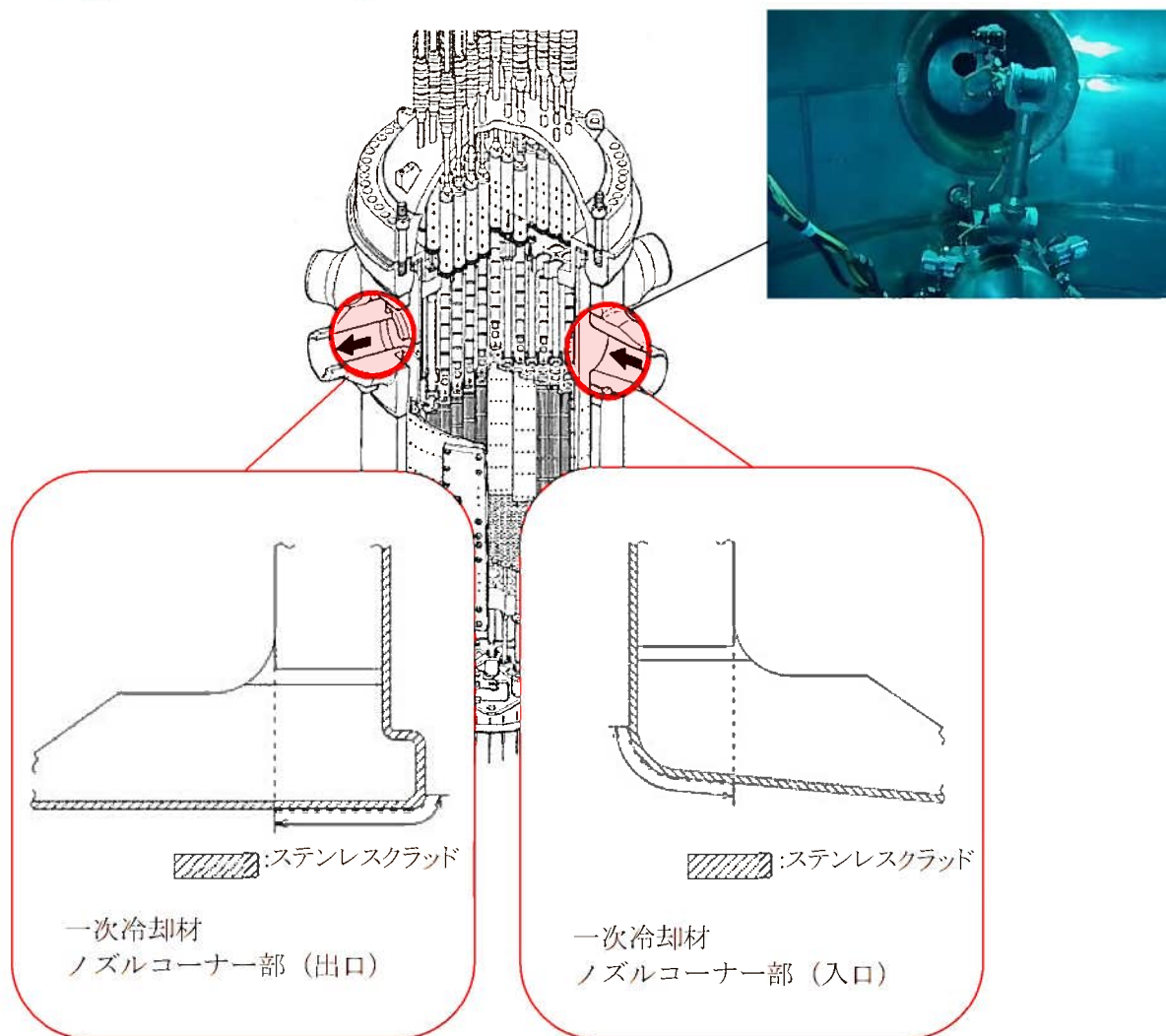
図3.2.2.1 試験対象(一次冷却材ノズルコーナー部)及び探傷画像(イメージ)
