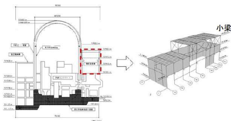
図 5.2.1 燃料取扱棟の解析モデル
