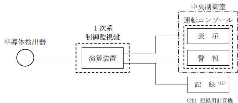
図 1.2.5 使用済燃料ピットエリアモニタの概略構成図
