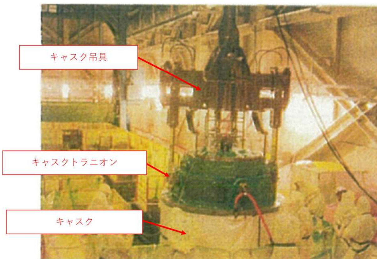
図1 キャスク吊具の現場での使用状況
