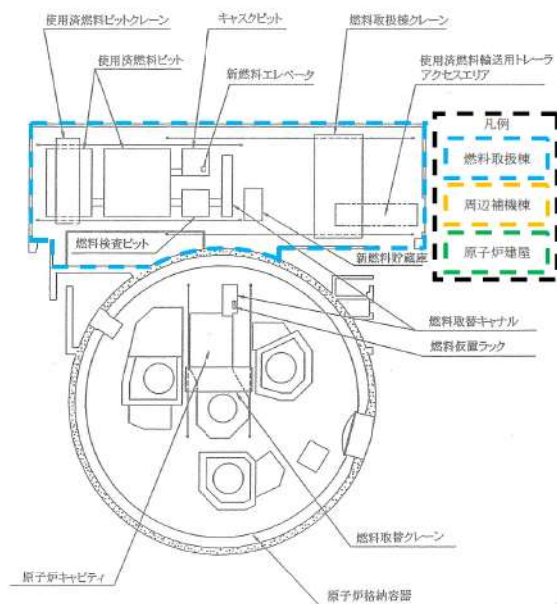
図 1 泊 3 号炉の建屋名称 (横断面図)
