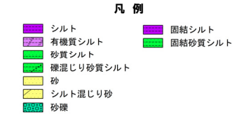
ボーリング柱状図 (深度40~45m)
