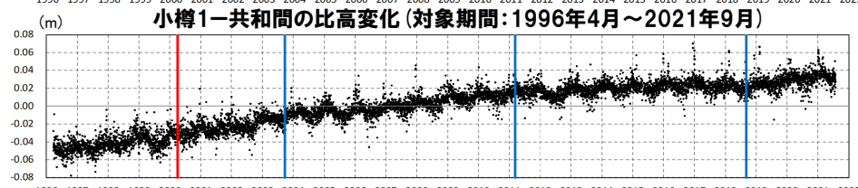
小樽1-共和間の比高変化(対象期間:1996年4月~2021年9月)
