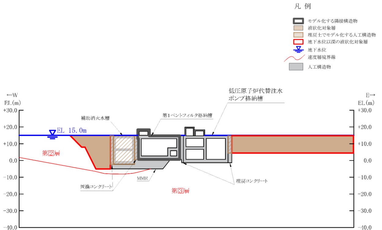
図 2-3 低圧原子炉代替注水ポンプ格納槽 評価対象断面図 (C-C断面)
