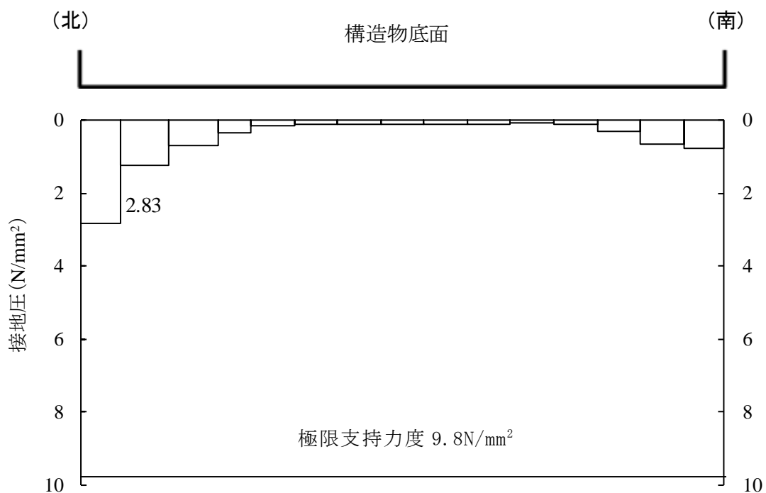
図 5-12 基礎地盤の最大接地圧分布図 (A-A断面, 解析ケース①, S s -D (+-))
