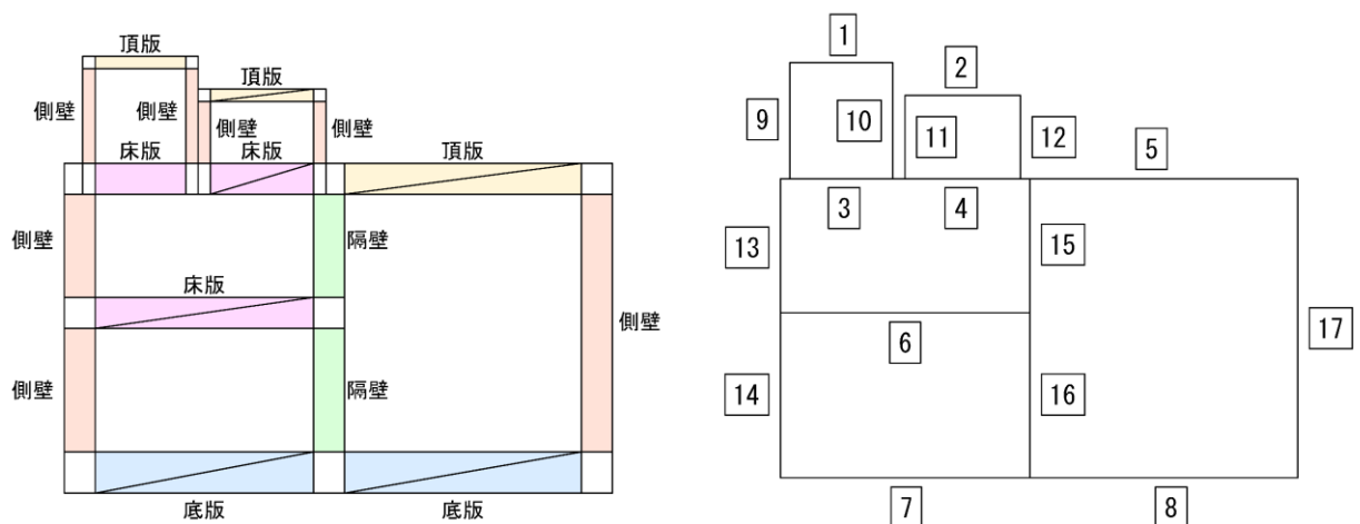
図 2-19 評価部位位置図
