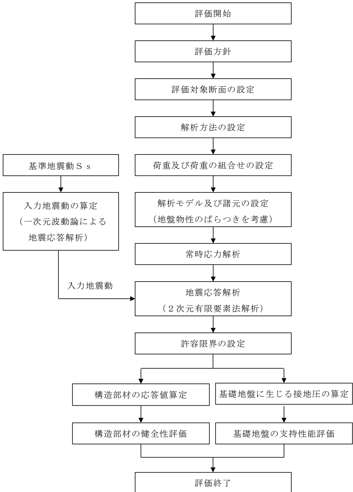
図 2-20 低圧原子炉代替注水ポンプ格納槽の耐震評価フロー
