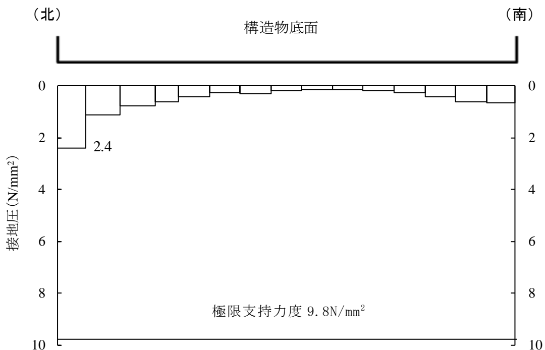
図 5-13 基礎地盤の最大接地圧分布図 (B-B断面, 解析ケース③, S s -D (+-))
