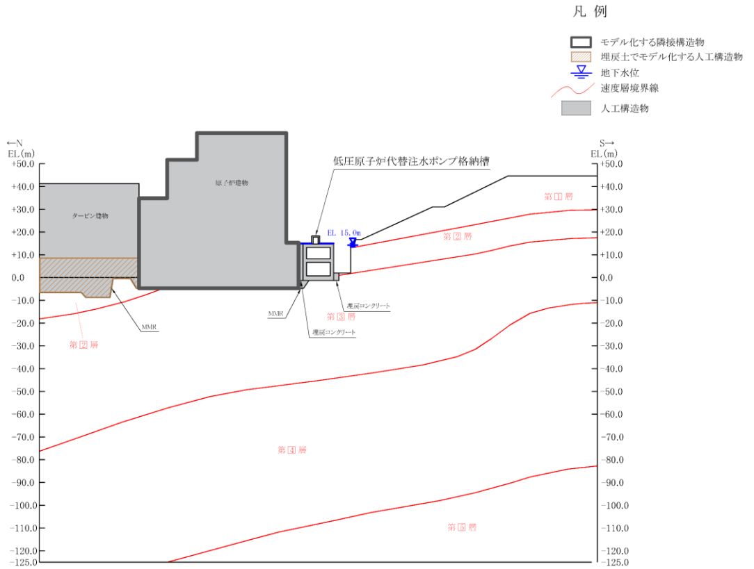
図 3-10 評価対象地質断面図 (A-A 断面)
