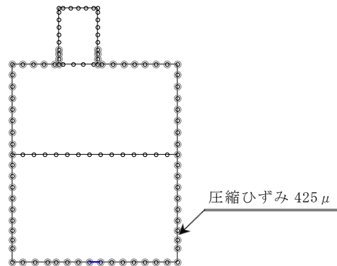
図 5-1 曲げ・軸力系の破壊に対する照査が最も厳しくなるケースの時刻歴波形 (全応力解析) (A-A断面, 解析ケース①, S s -D (+ -))
