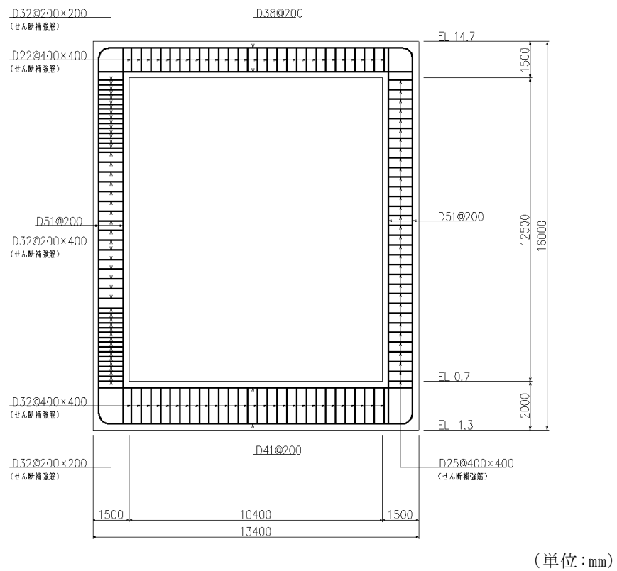
図 2-9 低圧原子炉代替注水ポンプ格納槽 概略配筋図 (B-B 断面)
