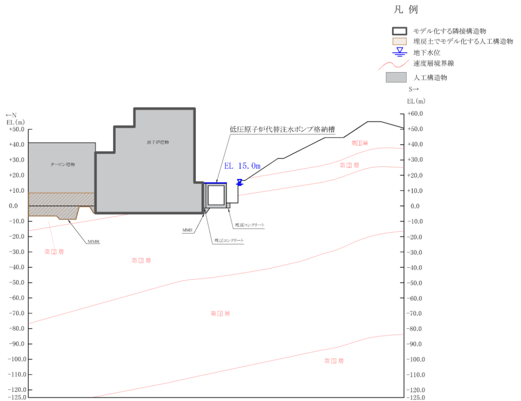
図 3-11 評価対象地質断面図 (B-B 断面)
