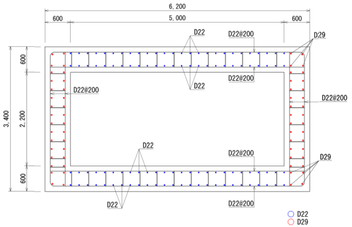
図 1-6 ケミカルアンカー設置位置図
