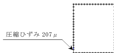
図 5-10 最大圧縮ひずみ発生位置（ケース①，S s - D（+-））
