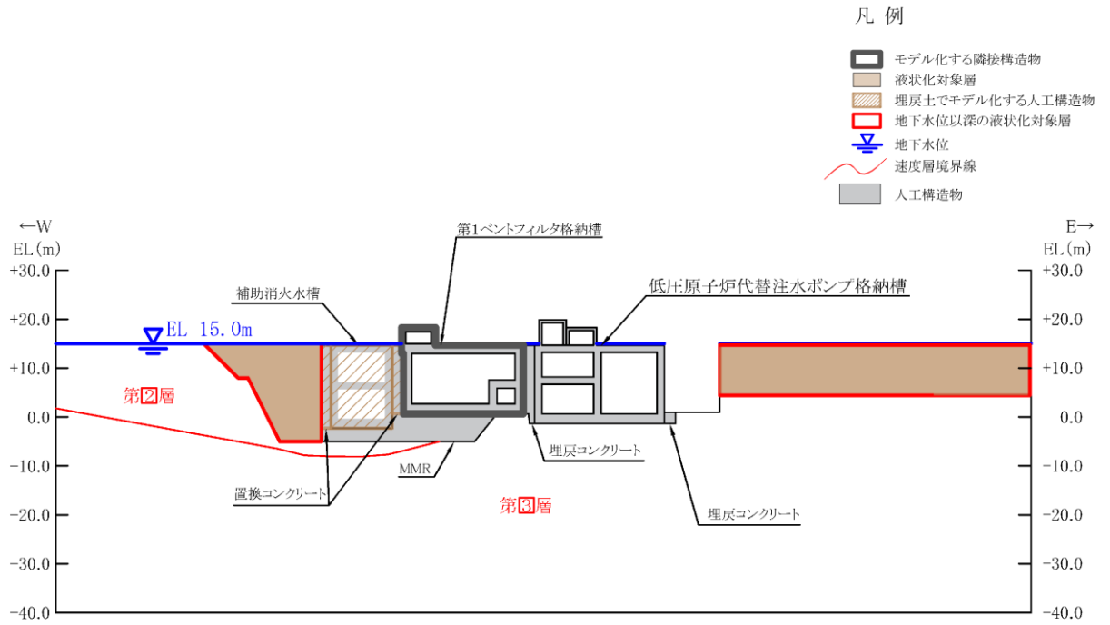
図 3-12 評価対象地質断面図 (C-C 断面)
