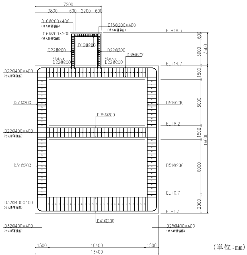
図 2-6 低圧原子炉代替注水ポンプ格納槽 概略配筋図 (A-A 断面)
