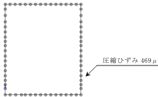
図 3-6 曲げ・軸力系の破壊に対する照査におけるひずみ（コンクリート）の時刻歴波形（B-B断面，解析ケース③，S s - N 1（++））
