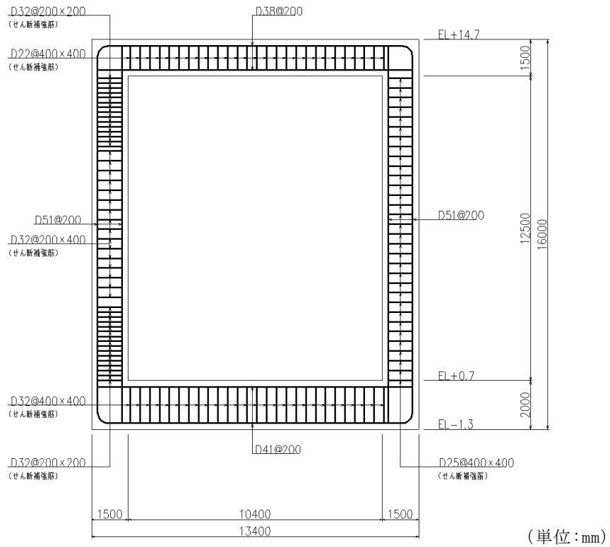
図 2-7 低圧原子炉代替注水ポンプ格納槽 概略配筋図 (B-B 断面)
