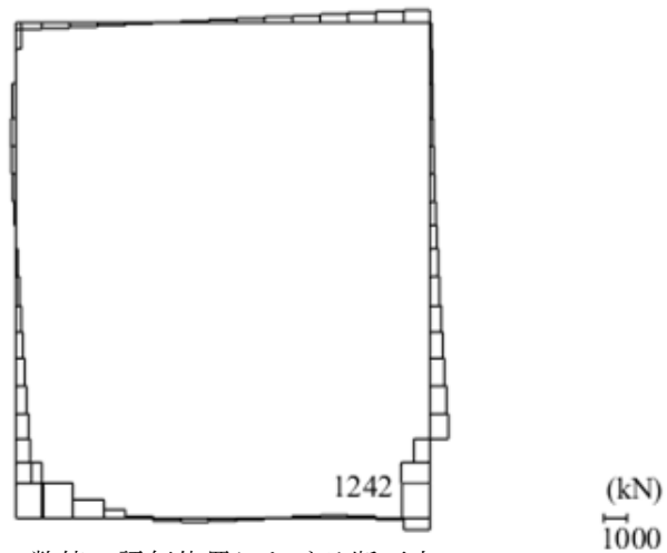
図 3-11 せん断破壊に対する照査値最大時の断面力図 (B-B断面, 解析ケース③, S s -D (+-), t=14.59s)
