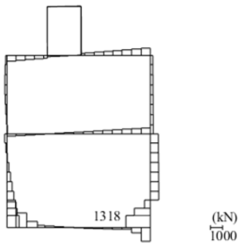
図 3-10 せん断破壊に対する照査値最大時の断面力図 (A-A断面, 解析ケース①, S s -D (---), t=8.79s)
