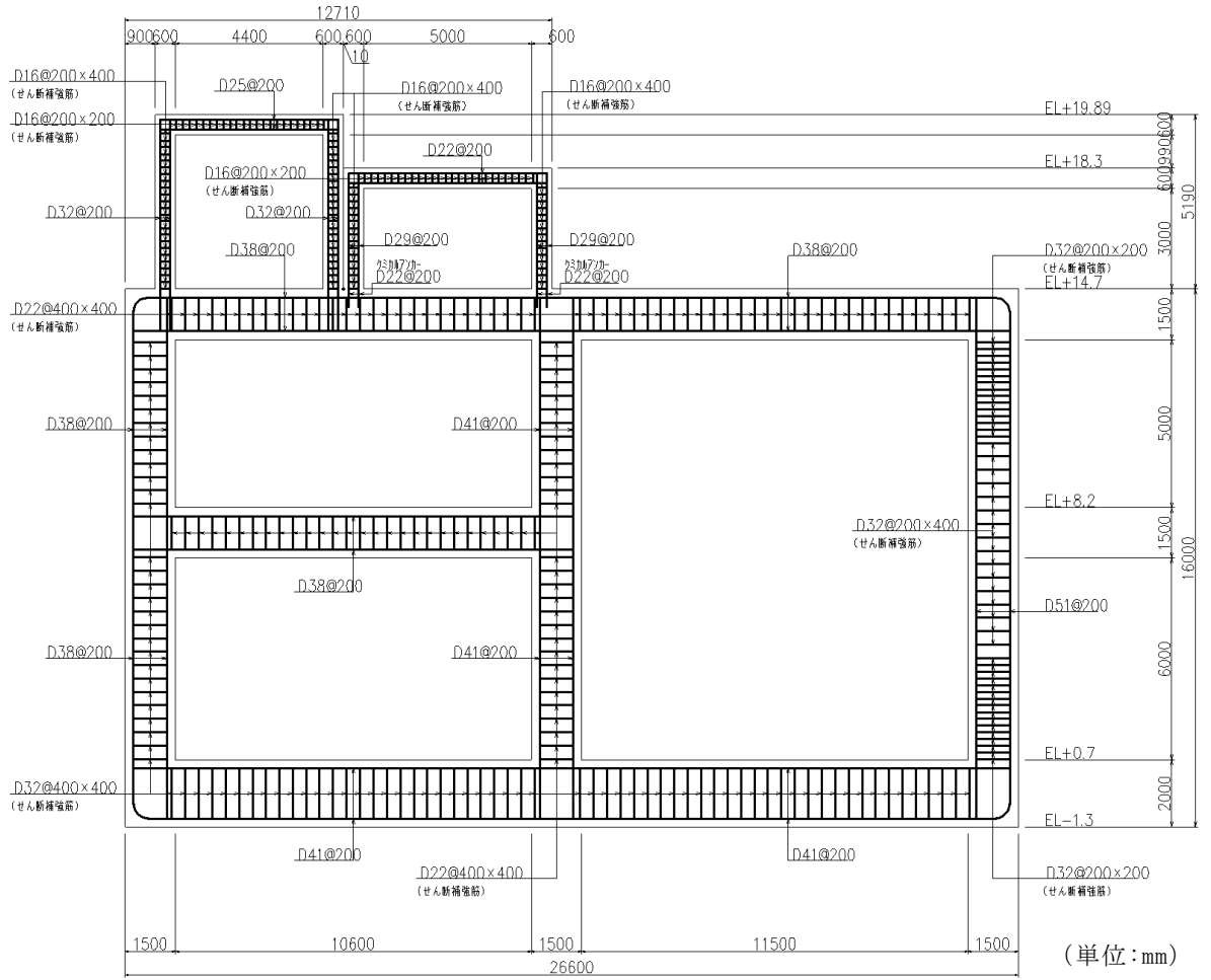
図 2-8 低圧原子炉代替注水ポンプ格納槽 概略配筋図 (C-C 断面)
