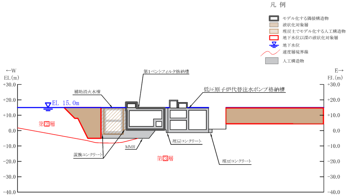
図 3-4 低圧原子炉代替注水ポンプ格納槽 評価対象断面図 (C-C 断面)
