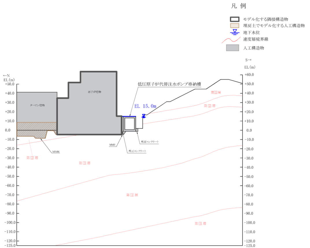
図 3-3 低圧原子炉代替注水ポンプ格納槽 評価対象断面図 (B-B断面)
