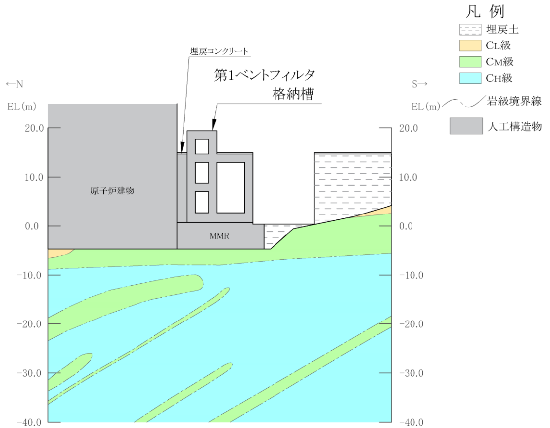
図 3-2 第 1 ベントフィルタ格納槽 評価対象断面図 (A-A断面)
