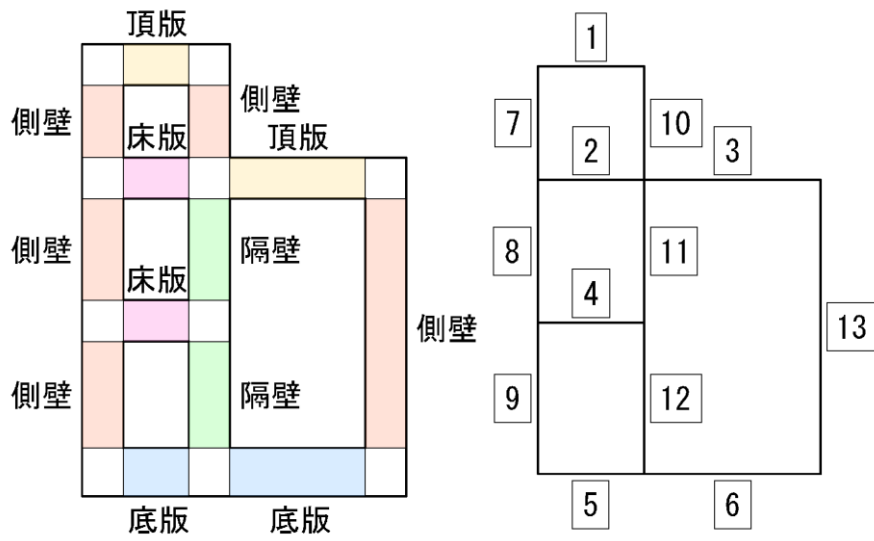
(A-A断面)
