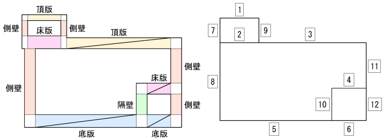
(B-B断面)
