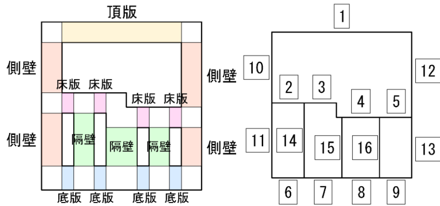
(B-B断面)
