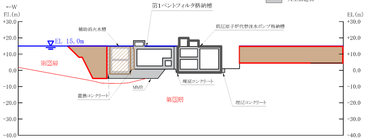
図 3-4 第 1 ベントフィルタ格納槽 評価対象断面図 (C-C 断面)
