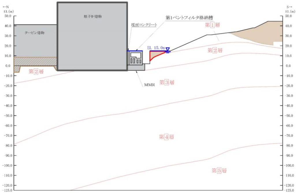
図 3-3 第 1 ベントフィルタ格納槽 評価対象断面図 (B-B 断面)
