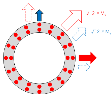
図5-13 曲げモーメントの算定概念図
