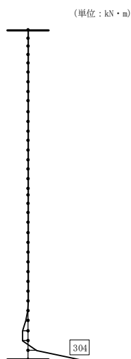
図 5-12 (2) 底版からの廻り込みを考慮した側壁の曲げモーメント図 鉄筋の曲げ軸力に対する評価 (A-A断面, S_s - D (+, -)) (検討ケース③)
