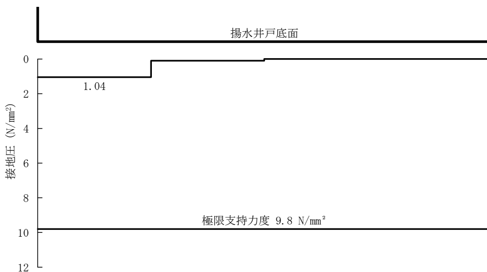
図 5-14 (9) A-A 断面の接地圧分布図 (S s -N 2 (NS)(++)) (検討ケース①)
