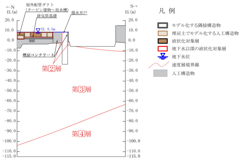
(速度層図)
