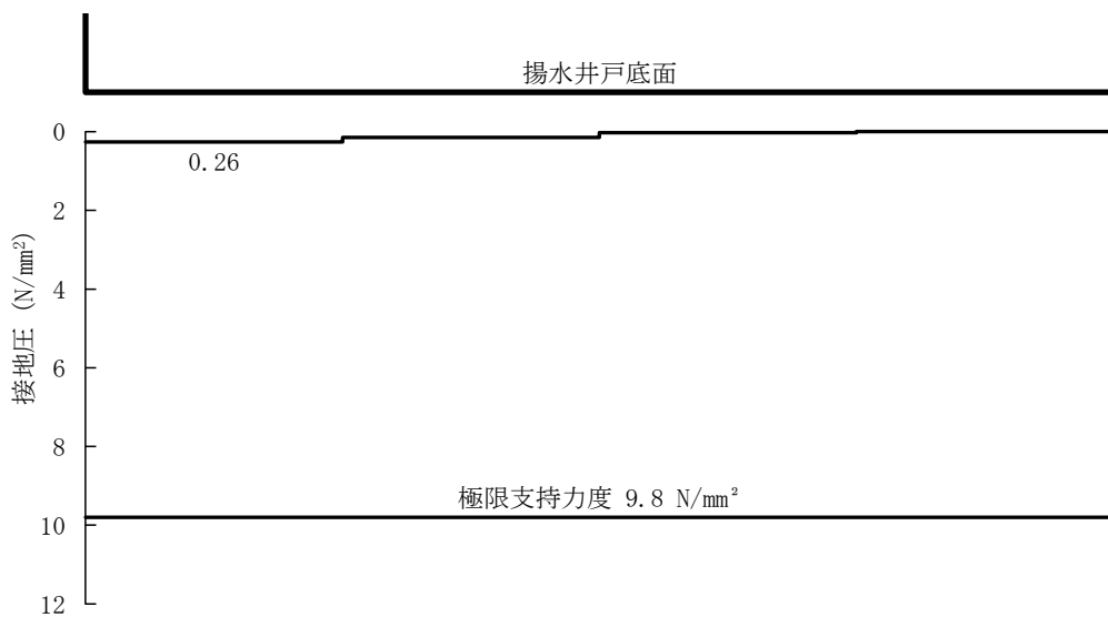
図 5-14 (25) B - B 断面の接地圧分布図 ( S s - N 2 ( E W ) ( + + ) ) ( 検 討 ケ ー ス ① )
