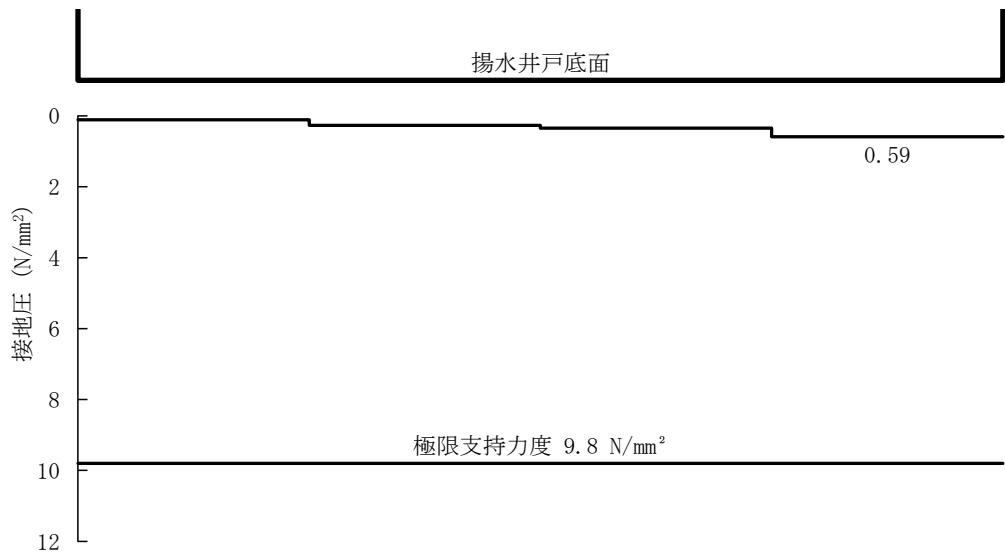
図 5-14 (18) B - B 断面の接地圧分布図 (S s - D (-)) (検討ケース①)
