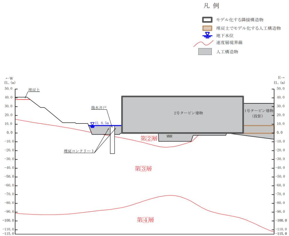
図 3-10 (1) 評価対象地質断面図 (A-A 断面 (東西方向))
