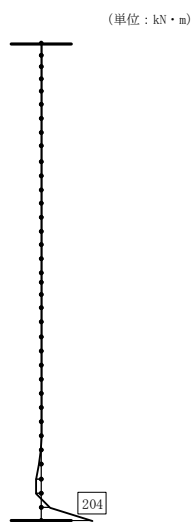
図 5-12 (4) 底版からの廻り込みを考慮した側壁の曲げモーメント図 鉄筋の曲げ軸力に対する評価 (B-B断面, S s - D (+, -)) (検討ケース①)
