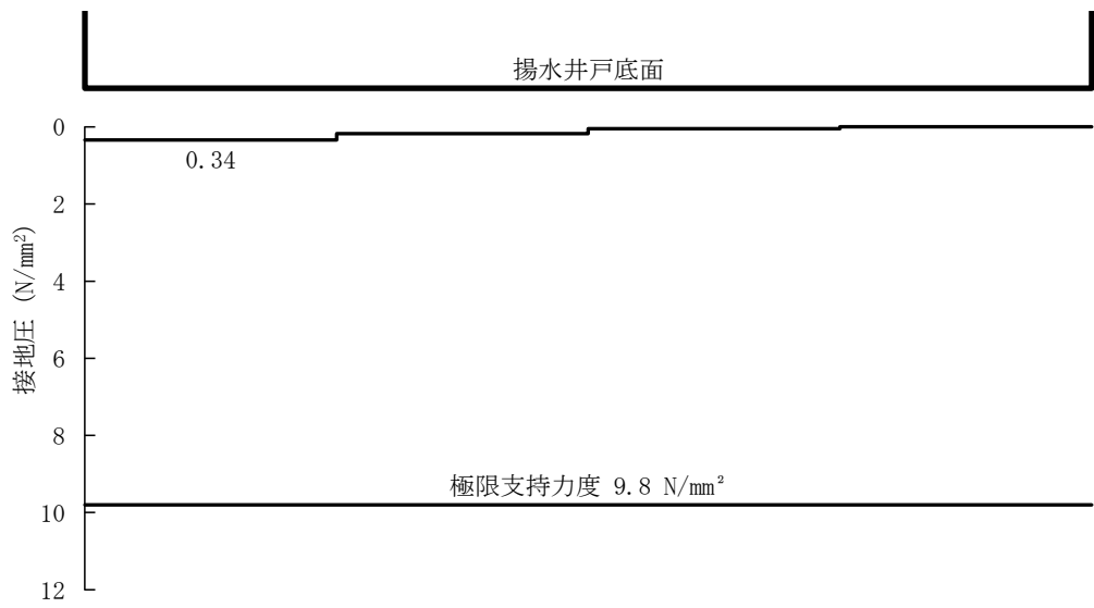
図 5-14 (17) B - B 断面の接地圧分布図 (S s - D (+)) (検討ケース①)
