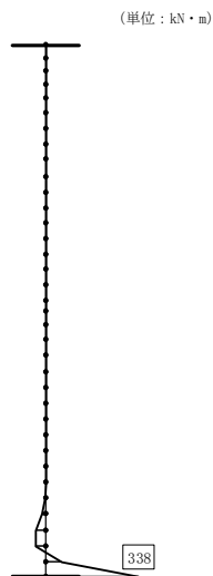
図 5-12 (1) 底版からの廻り込みを考慮した側壁の曲げモーメント図 コンクリートの曲げ軸力に対する評価 (A-A断面, S_s - N1 (-, +)) (検討ケース②)
