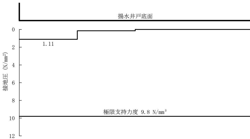
図 5-14 (2) A-A 断面の接地圧分布図 (S s - D (-+ ) ) (検討ケース①)
