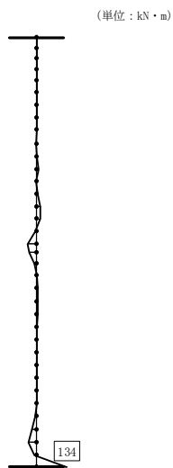
図 5-11 (4) 側壁両端固定はりモデルにおける曲げモーメント図 鉄筋の曲げ軸力に対する評価 (B-B断面, S s - D (+, -)) (検討ケース①)
