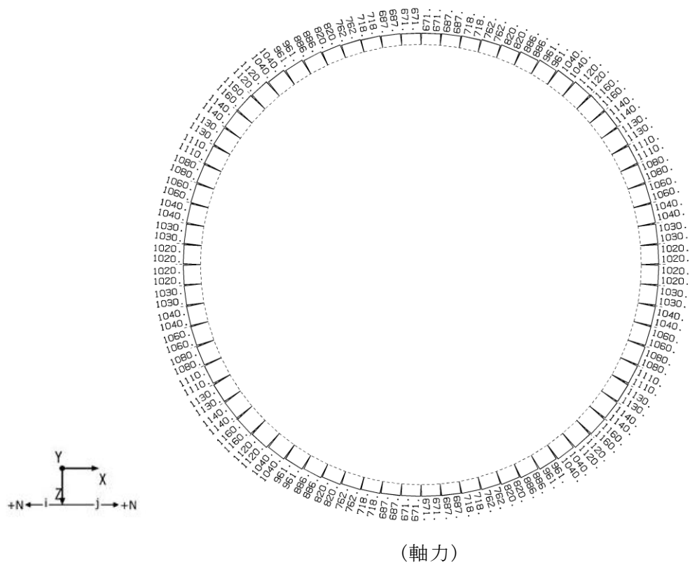
図 5-6 (6) コンクリート及び鉄筋の曲げ軸力が最も厳しい時刻の断面力 (B-B断面, 下部, S s - D (-, +), t = 8.55 s) (検討ケース③)
