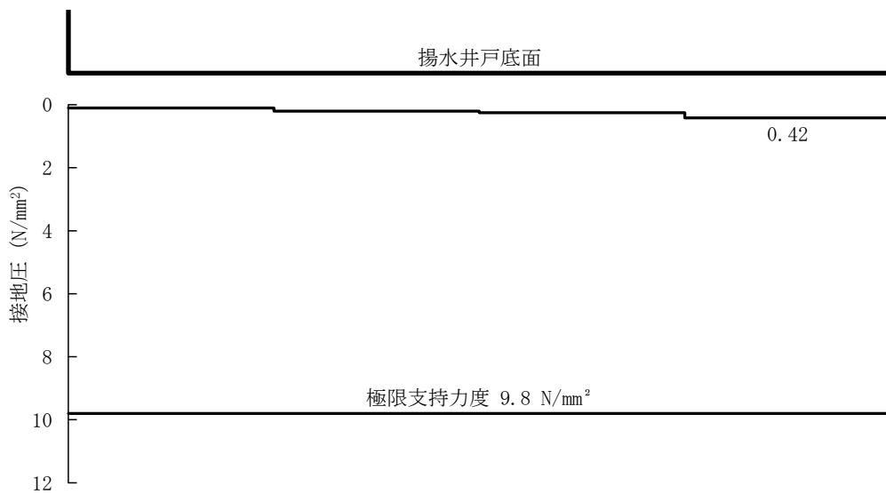
図 5-14 (26) B - B 断面の接地圧分布図 ( S s - N 2 ( E W ) ( - + ) ) ( 検 討 ケ ー ス ① )
