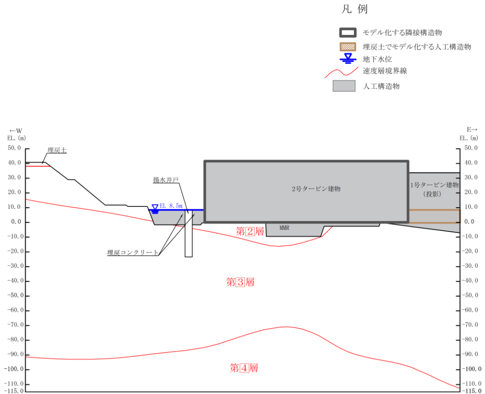
(速度層図)
