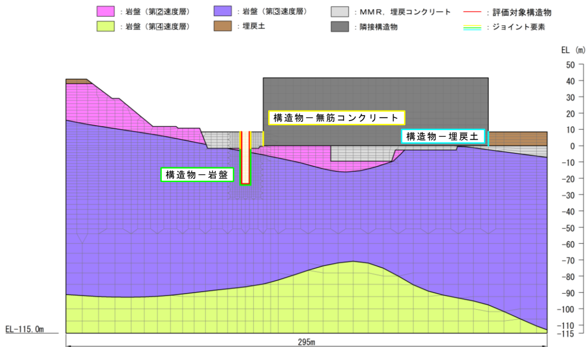
(A-A断面 (東西方向))
