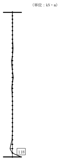
図 5-11 (3) 側壁両端固定はりモデルにおける曲げモーメント図 コンクリートの曲げ軸力に対する評価 (B-B断面, S s - D (+, +)) (検討ケース①)
