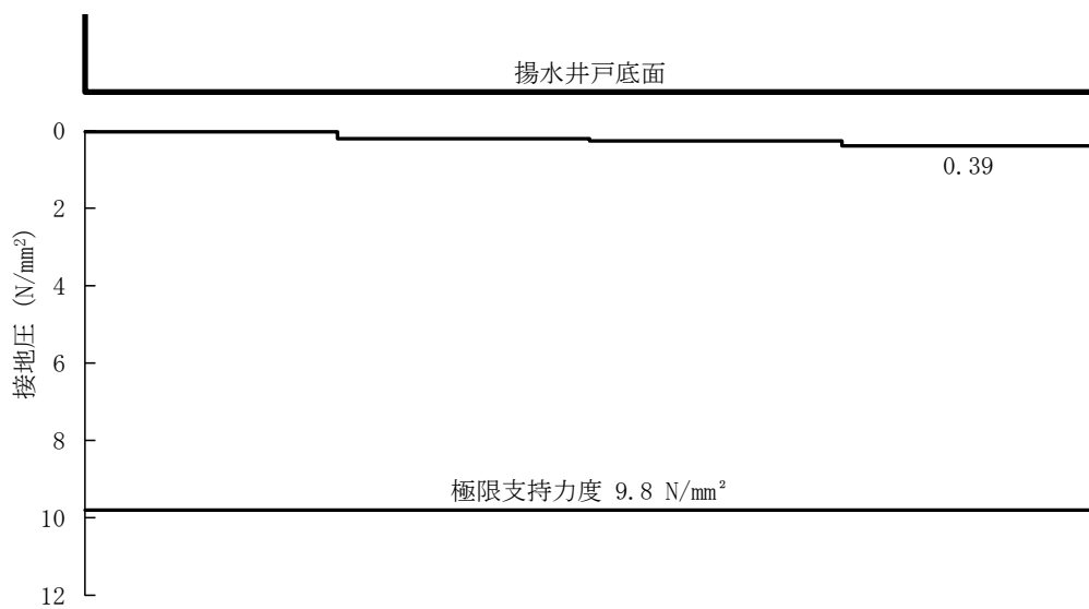
図 5-14 (16) B-B断面の接地圧分布図 (S s -D(-+))(検討ケース①)
