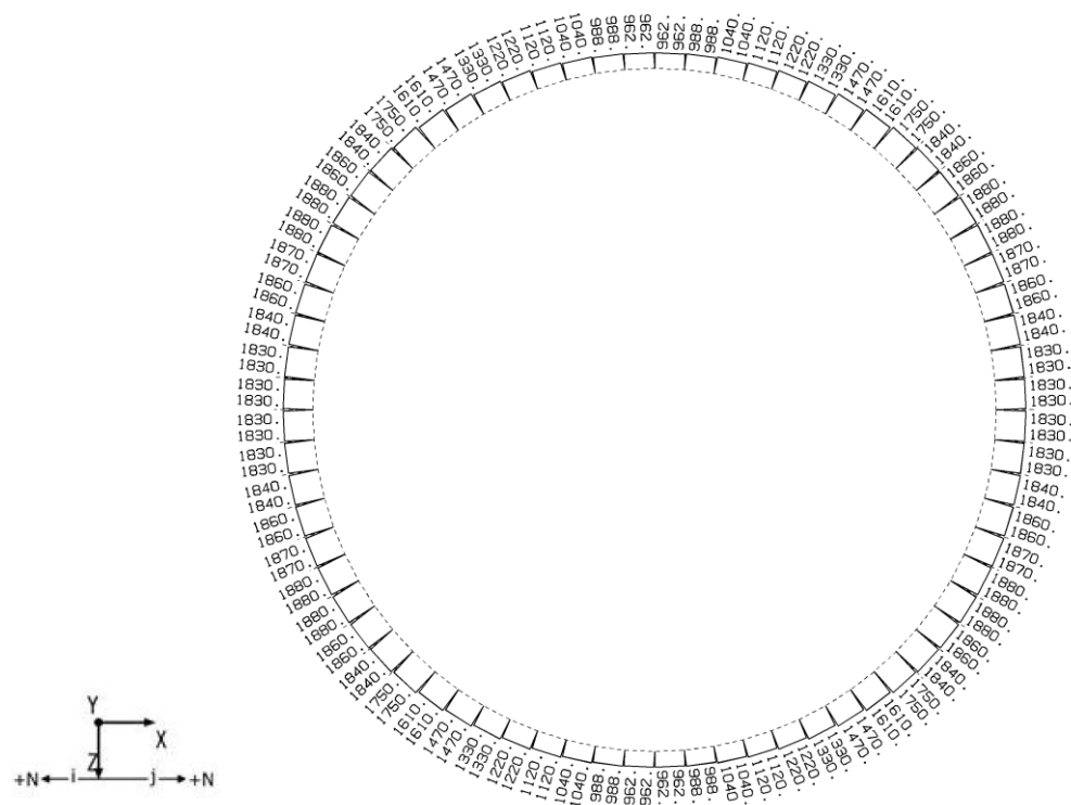
(軸力)
