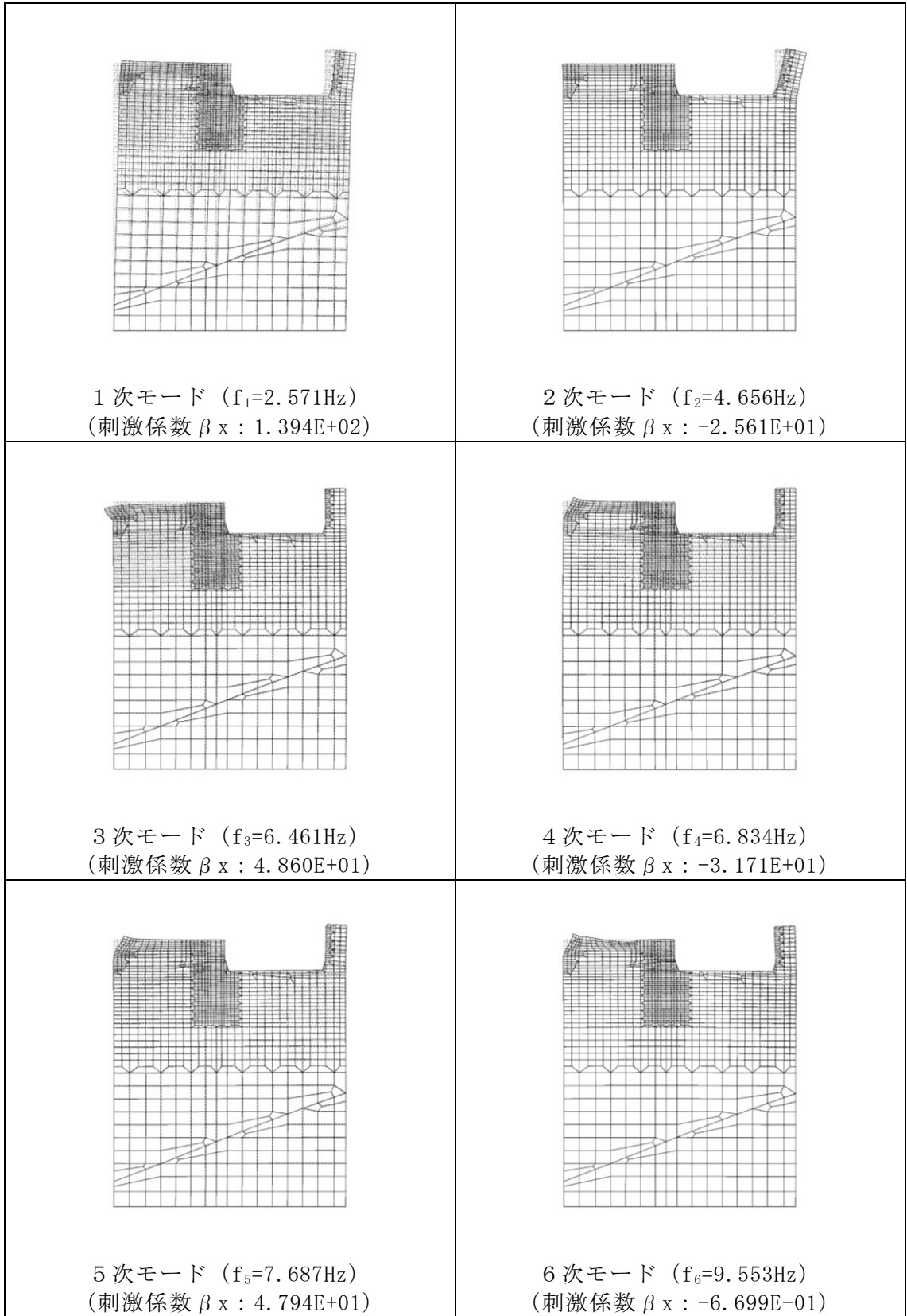
図 3-15 (3) 固有値解析結果 (モード図) (B-B断面 (南北方向))
