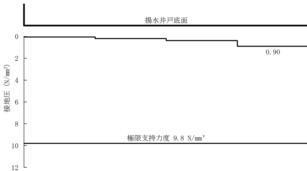
図 5-14 (11) A-A 断面の接地圧分布図 (S s - N 2 (EW) (++) (検討ケース①))
