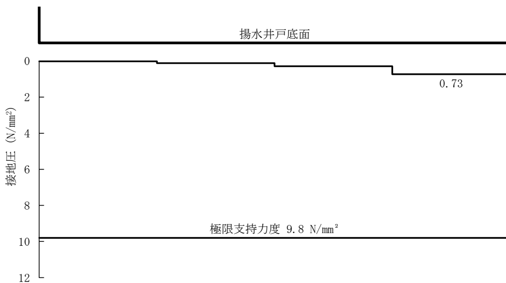
図 5-14 (10) A-A 断面の接地圧分布図 (S s -N 2 (NS)(-+)) (検討ケース①)
