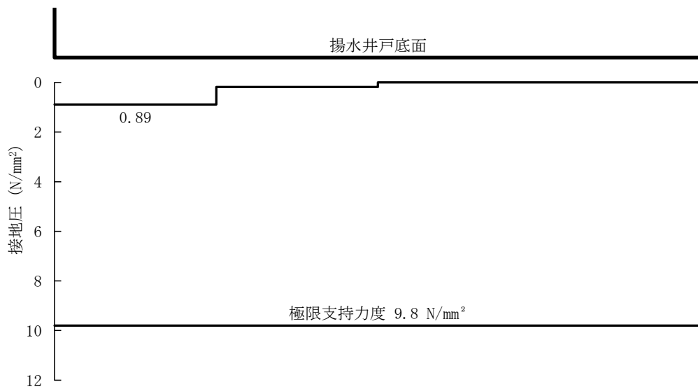
図 5-14 (12) A-A 断面の接地圧分布図 (S s - N 2 (EW) (-+) (検討ケース①))
