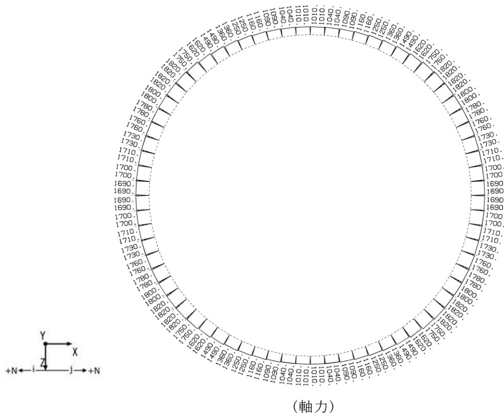
図 5-6 (3) コンクリート及び鉄筋の曲げ軸力が最も厳しい時刻の断面力 (A-A断面, 下部, S s - N 1 (+, +), t = 7.61 s) (検討ケース③)
