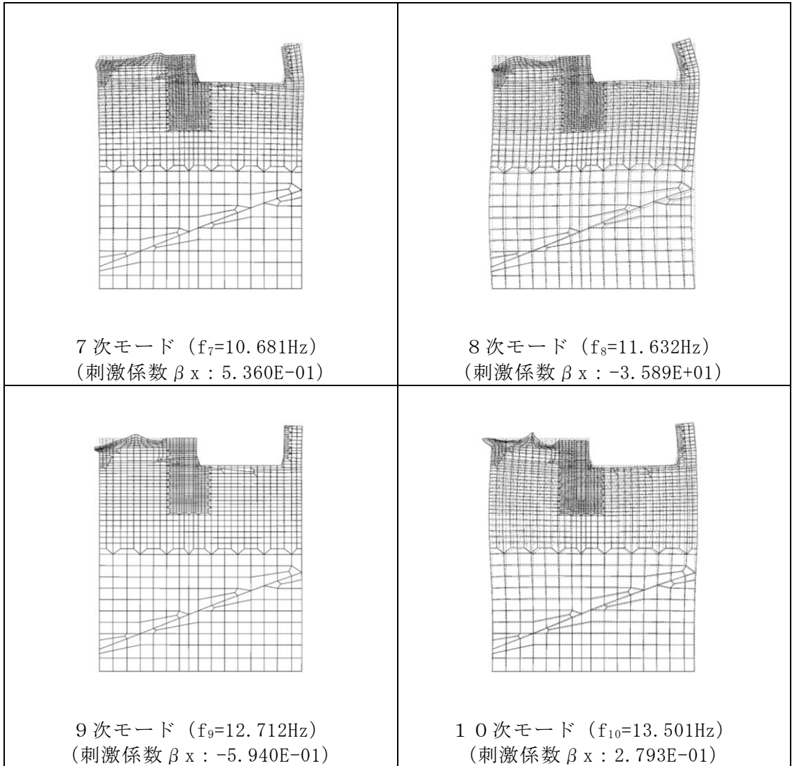
図 3-15 (4) 固有値解析結果 (モード図) (B-B 断面 (南北断面))
