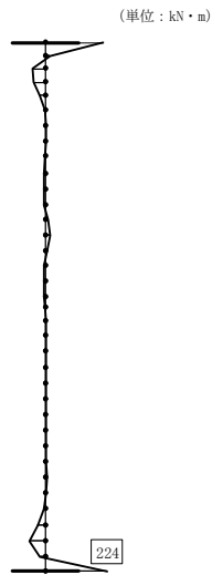
図 5-11 (1) 側壁両端固定はりモデルにおける曲げモーメント図 コンクリートの曲げ軸力に対する評価 (A-A断面, S_s - N1 (-, +)) (検討ケース②)
