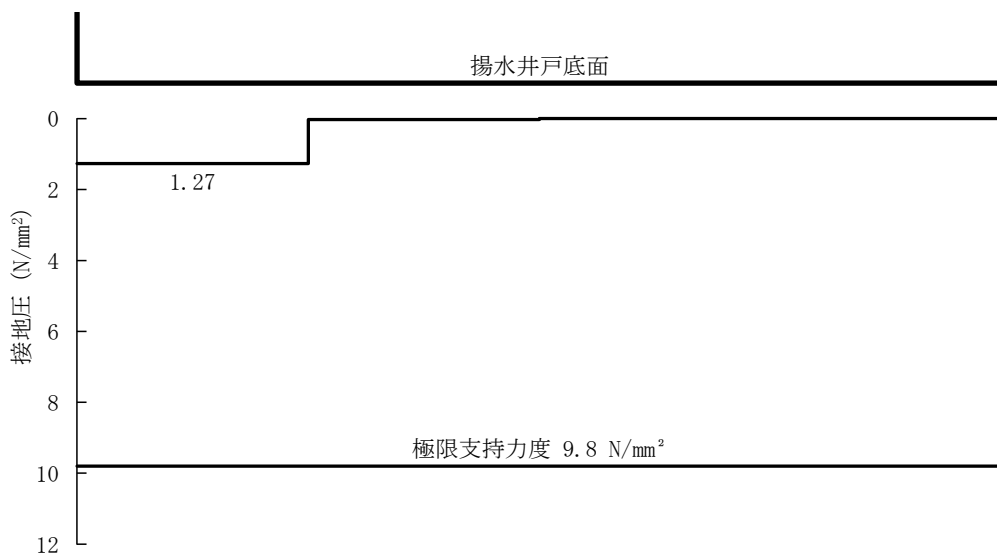
図 5-14 (1) A-A 断面の接地圧分布図 (S s - D (++) ) (検討ケース①)
