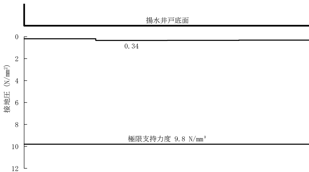
図 5-14 (15) B-B断面の接地圧分布図 (S s -D(++))(検討ケース①)
