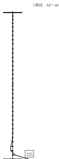
図 5-12 (3) 底版からの廻り込みを考慮した側壁の曲げモーメント図 コンクリートの曲げ軸力に対する評価 (B-B断面, S s - D (+, +)) (検討ケース①)
