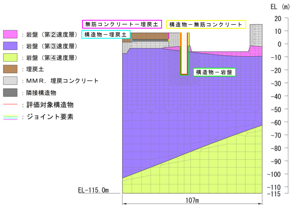
(B-B断面 (南北方向))
