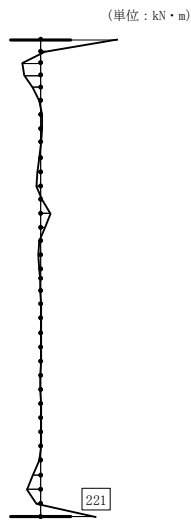
図 5-11 (2) 側壁両端固定はりモデルにおける曲げモーメント図 鉄筋の曲げ軸力に対する評価 (A-A断面, S_s - D (+, -)) (検討ケース③)
