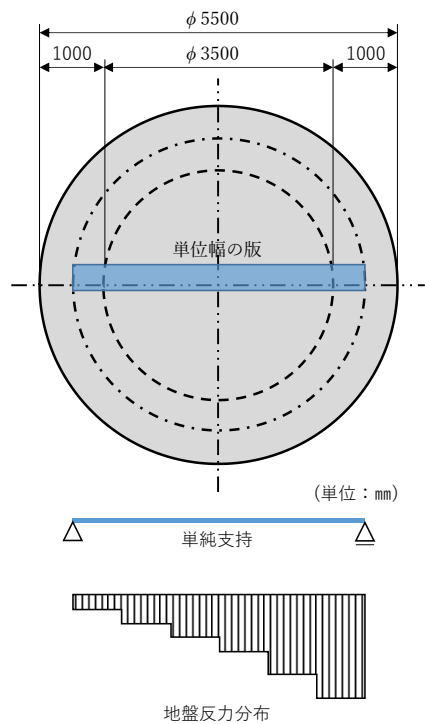
図4-18 底版の応答解析概念図
