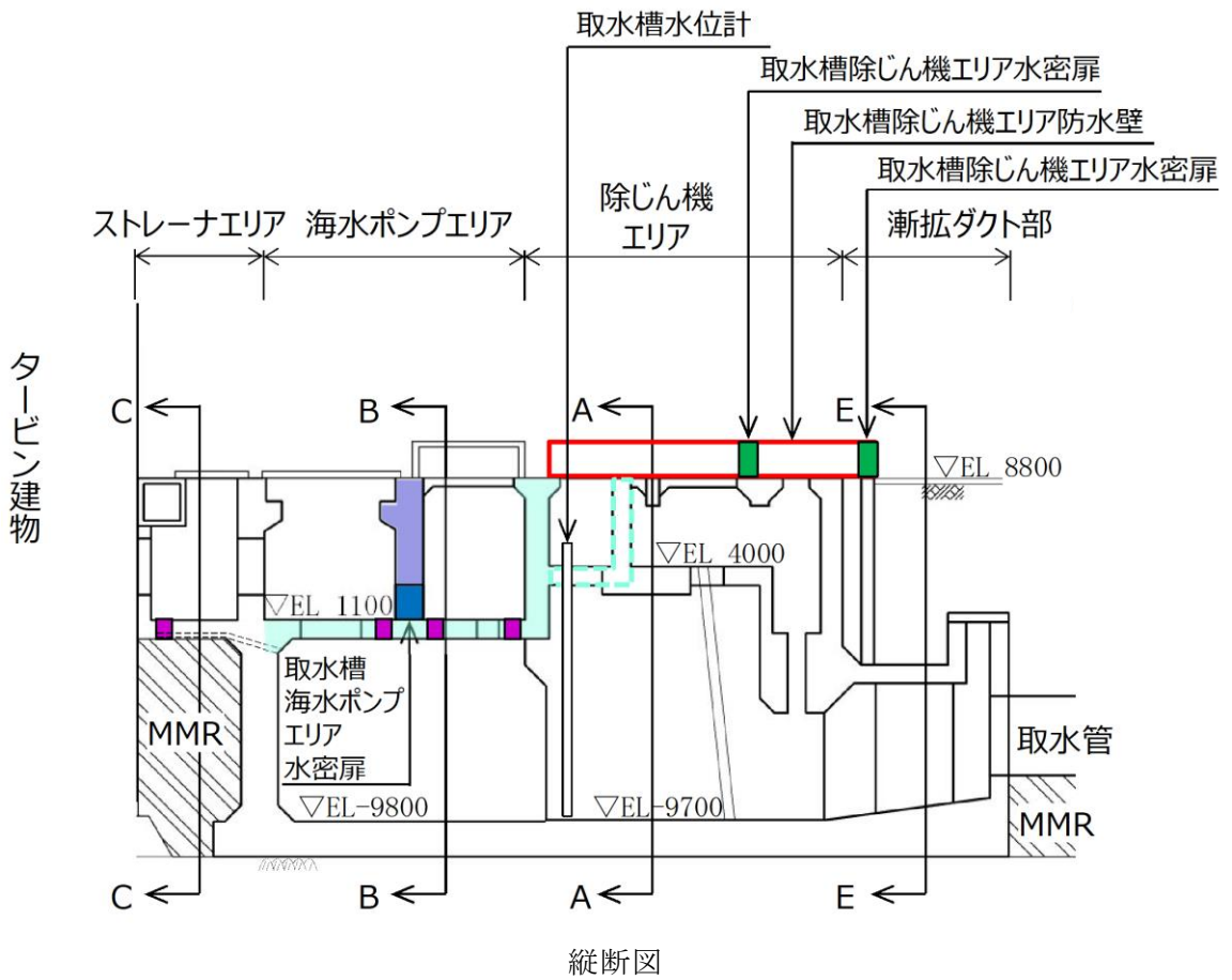
図 4.4-7 取水槽のうち止水機能が要求される範囲
