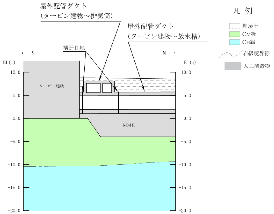
(岩級図)
