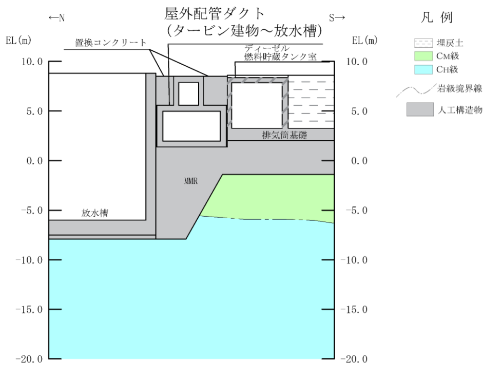
(岩級図)
