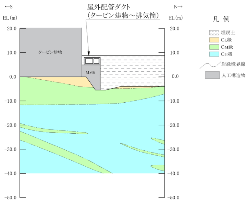
(岩級図)
