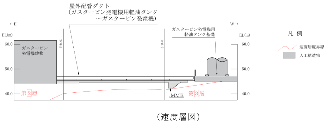
図 4.15-4 (2) 屋外配管ダクト (ガスタービン発電機用軽油タンク～ガスタービン発電機) 地質断面図 (B-B断面)
