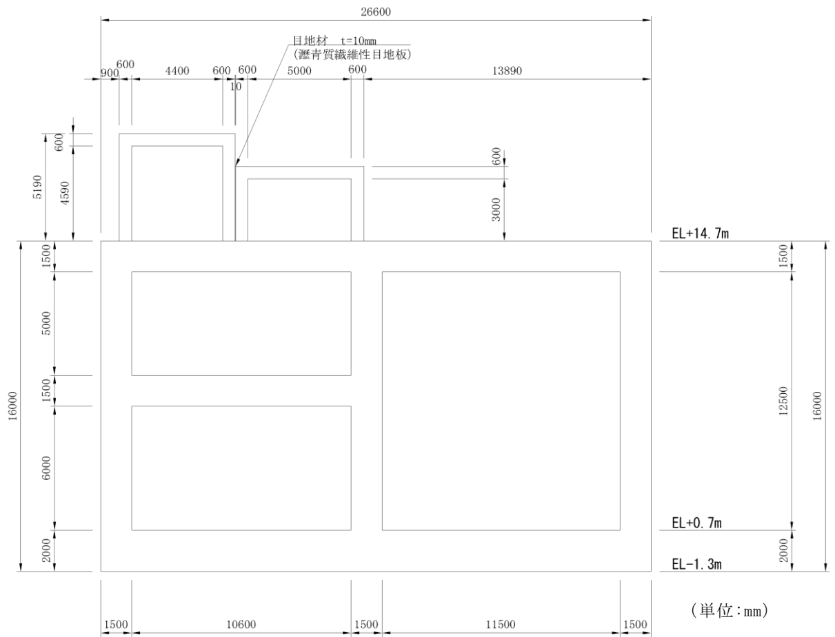
図 4.12-3 (3) 低圧原子炉代替注水ポンプ格納槽 断面図 (C-C 断面)
