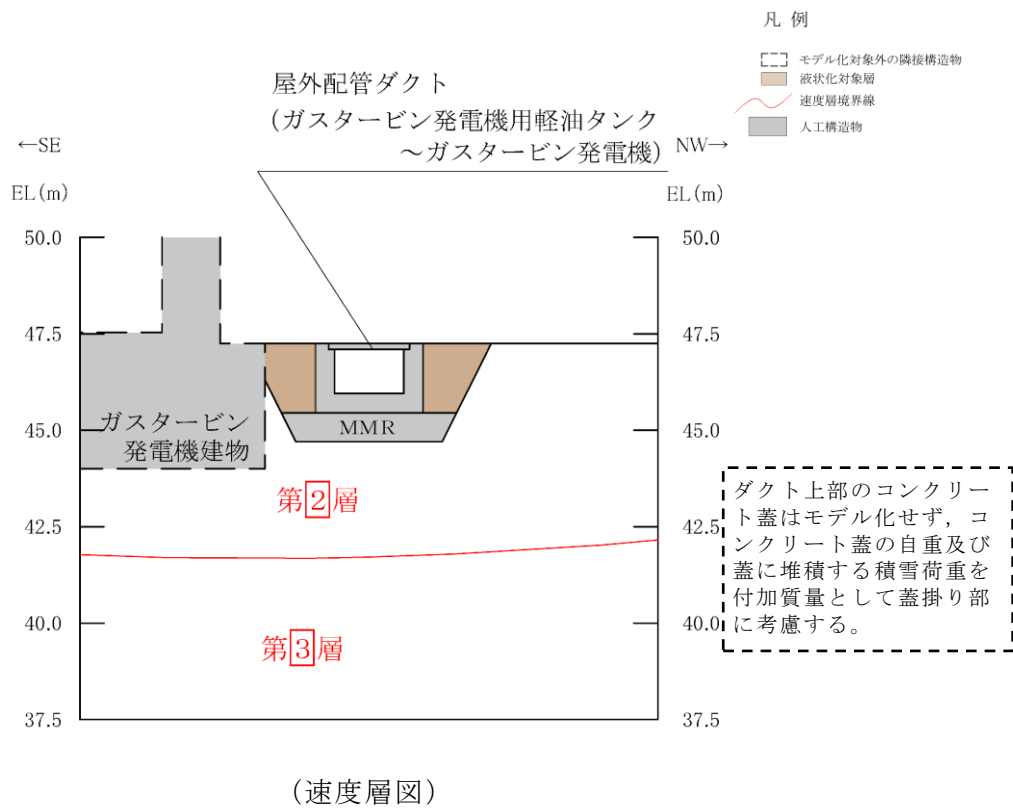
図 4.15-4 (1) 屋外配管ダクト
