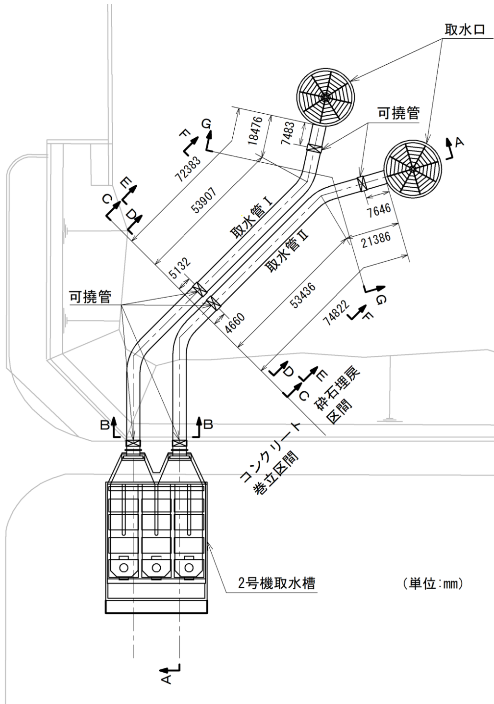
图4.9-2 取水管 平面图
