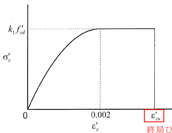
図6.2-4 コンクリートの応力-ひずみ関係と評価式
