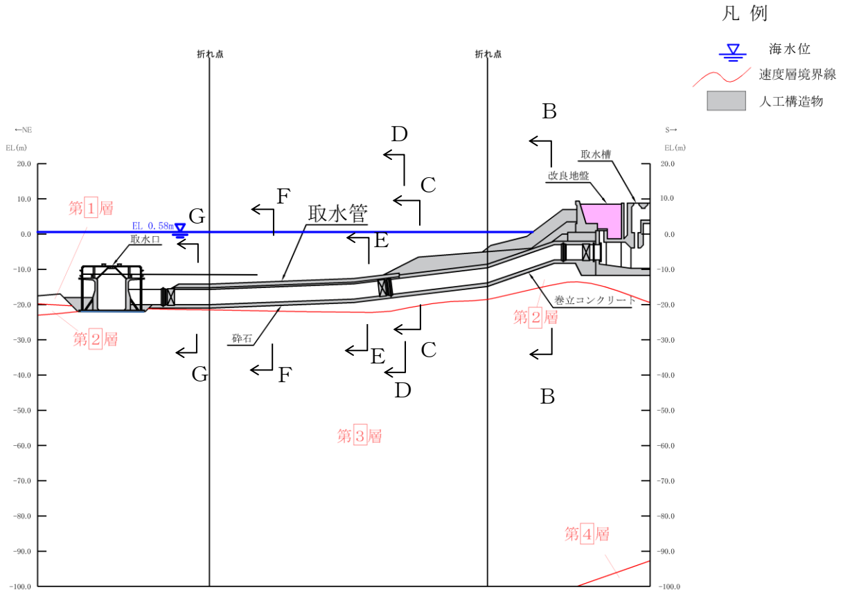
(速度層図)
