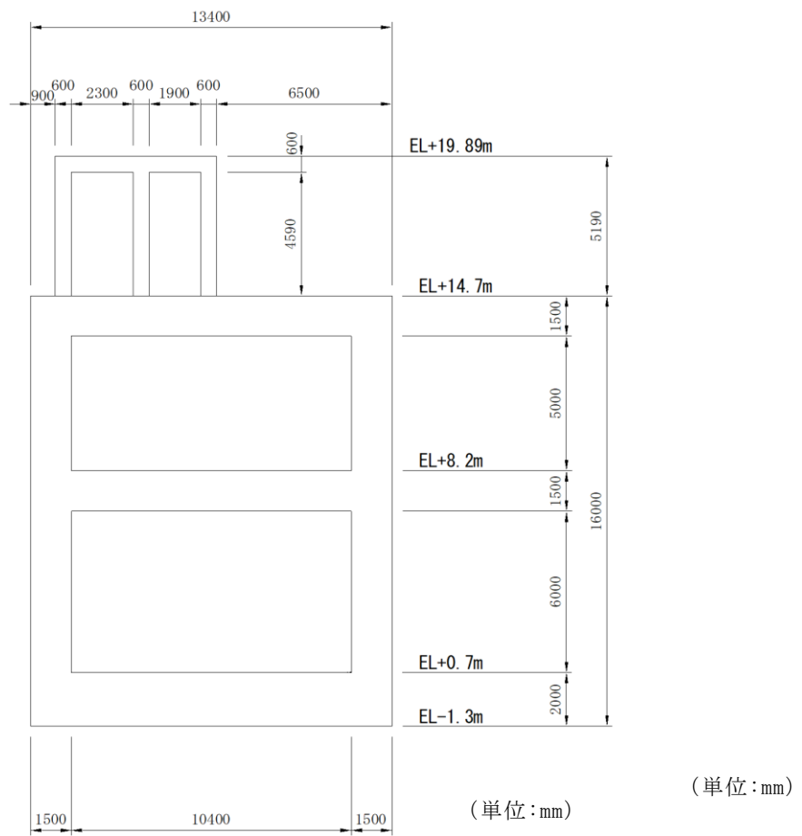
図 4.12-3 (5) 低圧原子炉代替注水ポンプ格納槽 断面図 (E-E断面)
