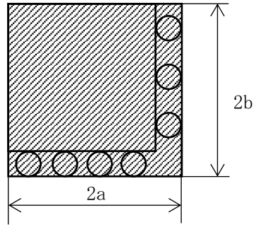
図 5.2-2 計算モデル図 ( 架構 )
