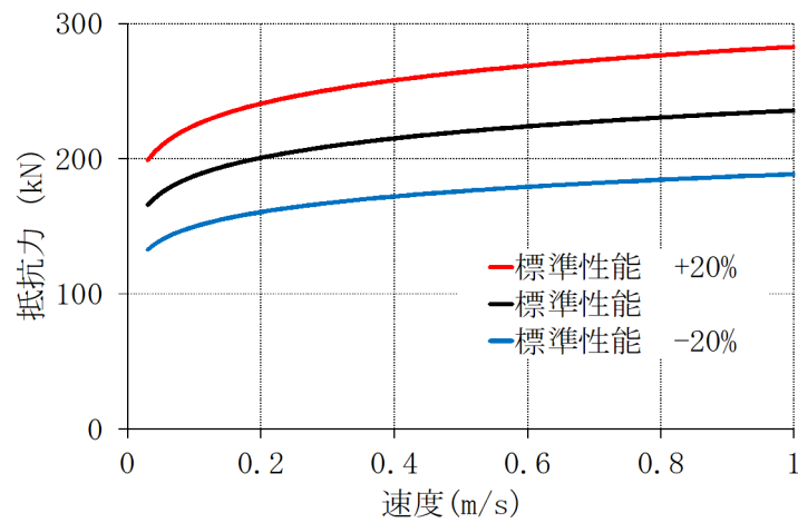
図 3-10 地震応答解析モデルにおける段階的な減衰性能の設定
