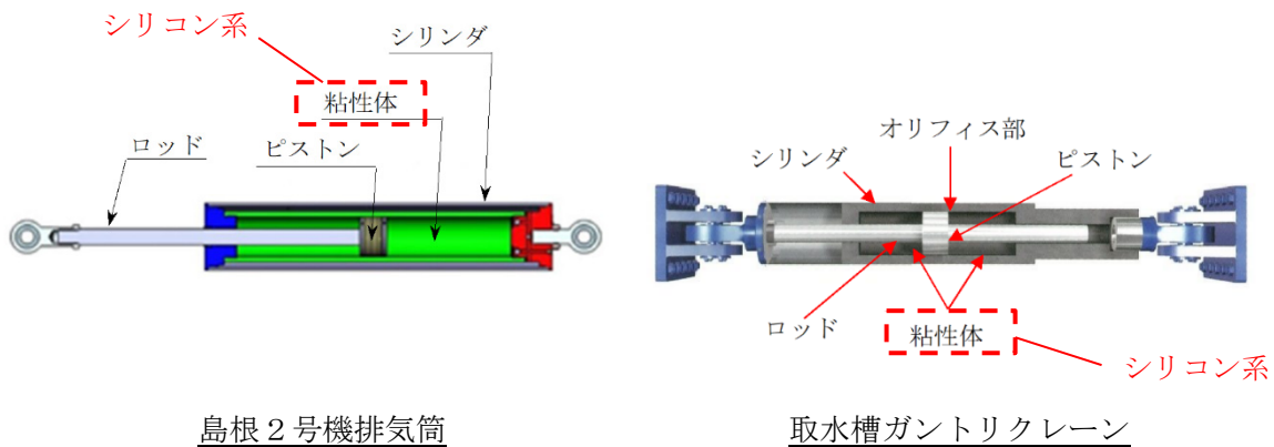
図 2-2 単軸粘性ダンパの構造比較
