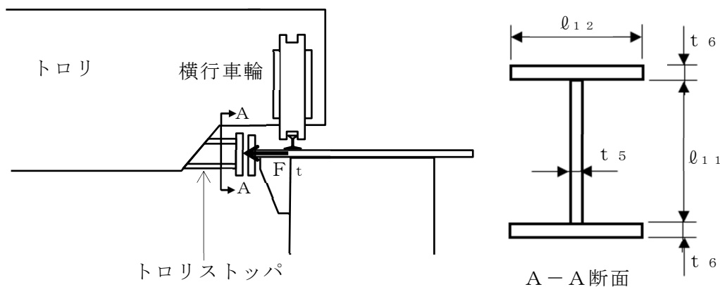
図 4-15 トロリストッパの概要図
