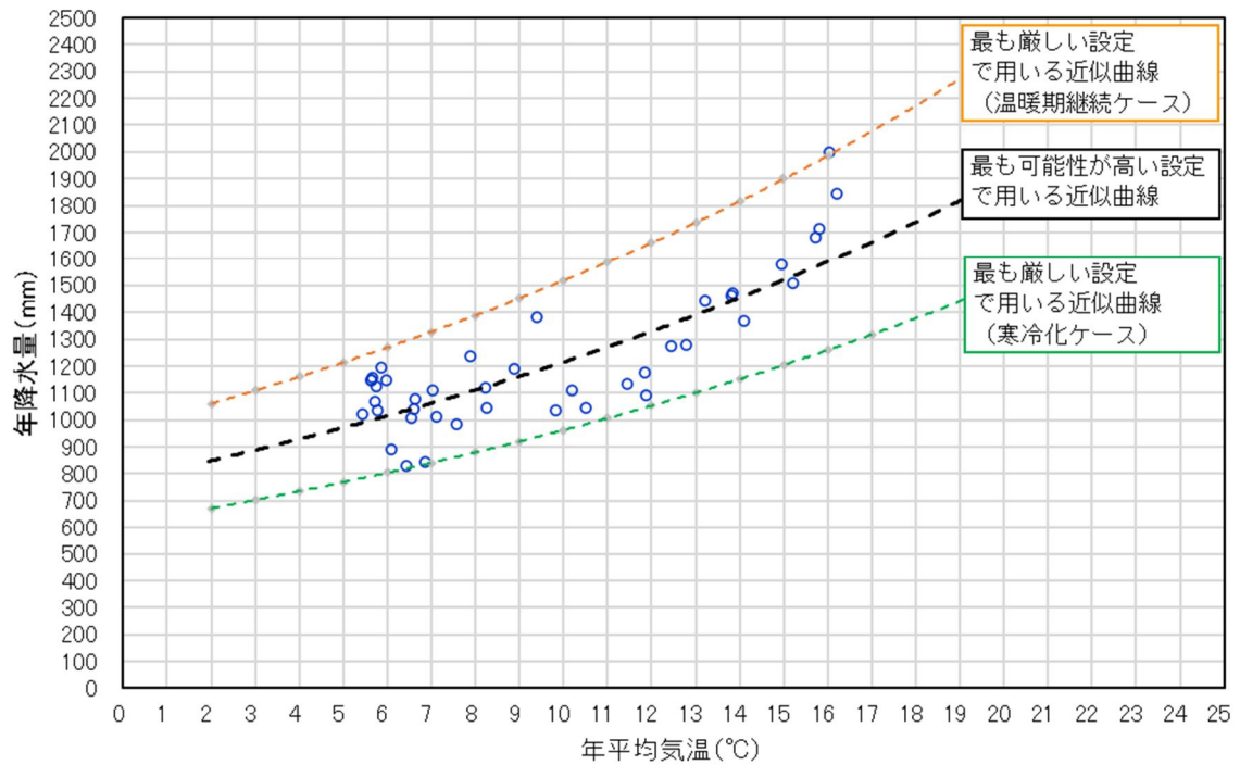
第 11 図 敷地周辺と類似する気候因子を持つ地点の気温と年降水量の相関
