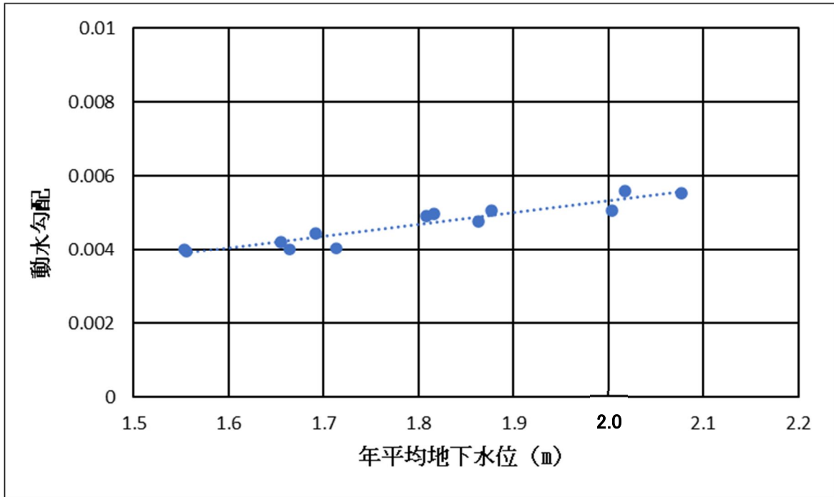
第 14 図 年平均地下水位と年間の動水勾配の相関
