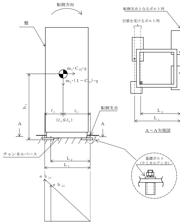
図5-1(7) 計算モデル
