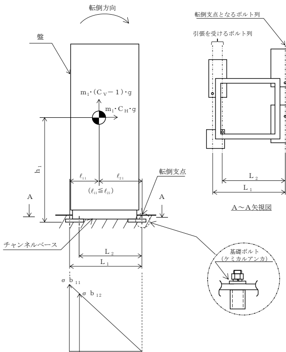
図5-1(8) 計算モデル
