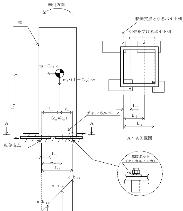
図5-1(3) 計算モデル
