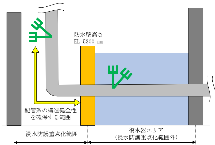
図 3-1 構造健全性を確保する範囲（高さによる範囲）
