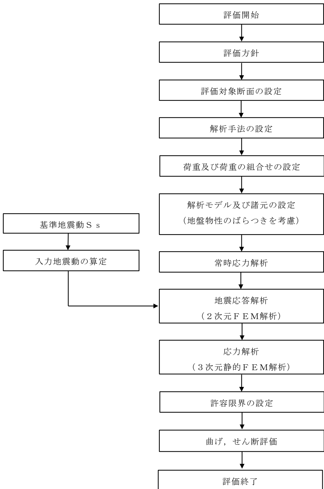
図 2-6 復水貯蔵タンク遮蔽壁の波及的影響の評価フロー
