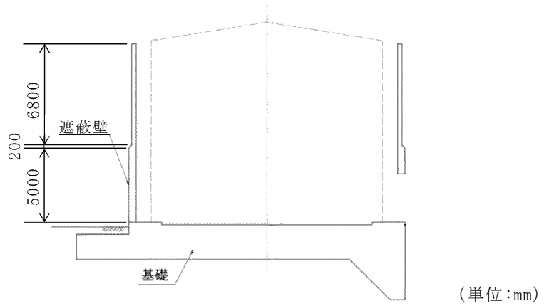
図 2-3 復水貯蔵タンク遮蔽壁 断面図 (A-A 断面, 南北)
