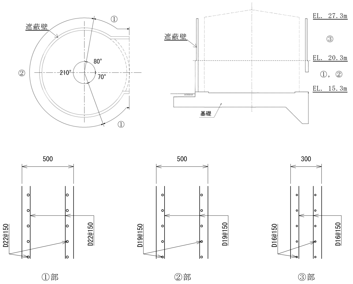
図 2-5 概略配筋図
