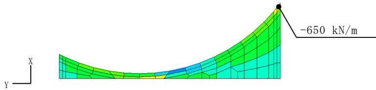
遮蔽壁（開口部頂版）
