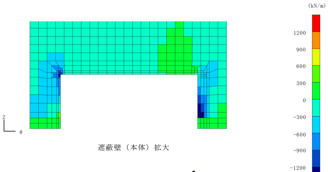
遮蔽壁（本体）
