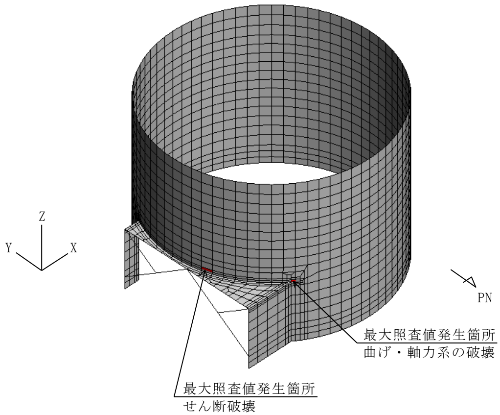
図 6-7 最大照査値発生箇所位置図（鳥瞰図，北東側から望む）
