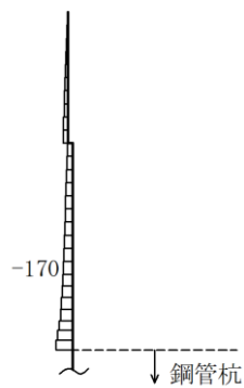
数値：評価位置における断面力 (c) せん断力 (kN)
