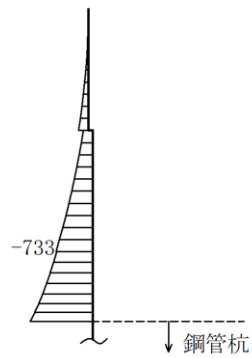
数値：評価位置における断面力 (a) 曲げモーメント (kN・m)
