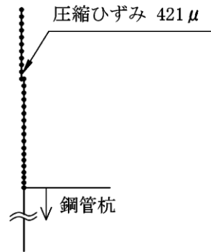
図 4-1 曲げ・軸力系の破壊に対する照査が最も厳しくなるケースの圧縮縁コンクリートひずみの時刻歴波形及び発生位置 (解析ケース①, S s -D (++) )
