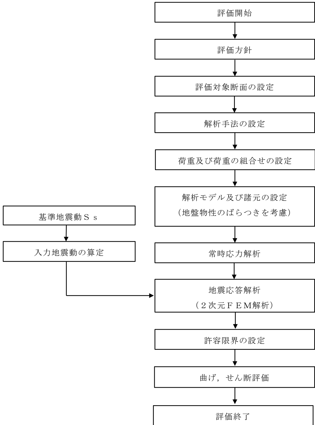
図 2-6 免震重要棟遮蔽壁の耐震評価フロー
