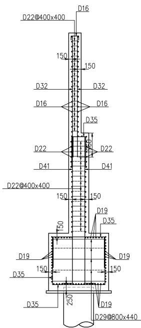
図 2-5 免震重要棟遮蔽壁の概略配筋図
