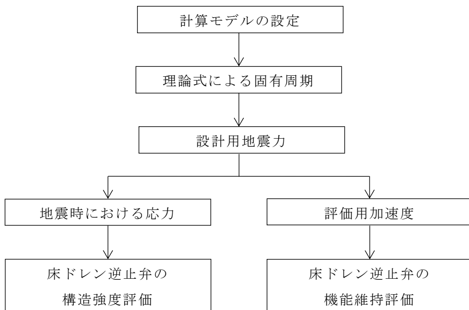
図 2-1 床ドレン逆止弁の耐震評価フロー
