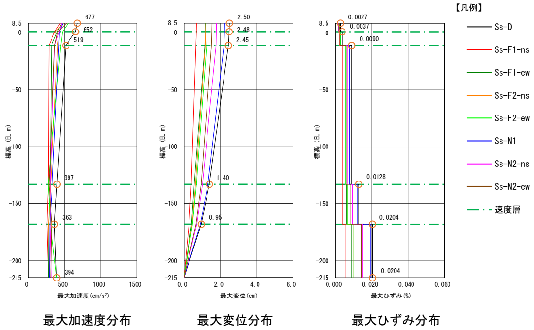
図 7(1) 第 4 保管エリア南側（水平方向）
