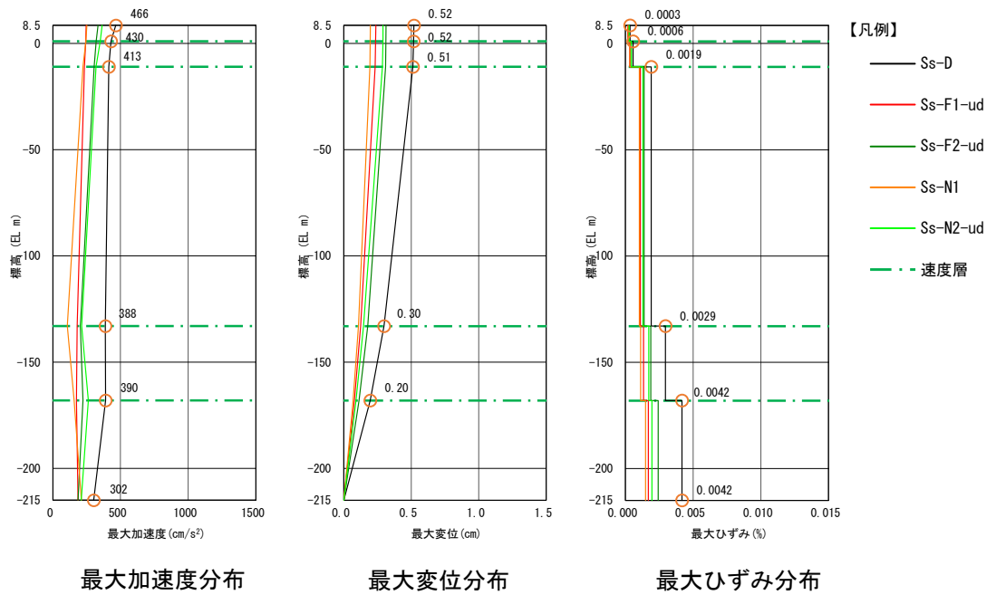
図 7(2) 第 4 保管エリア南側（鉛直方向）
