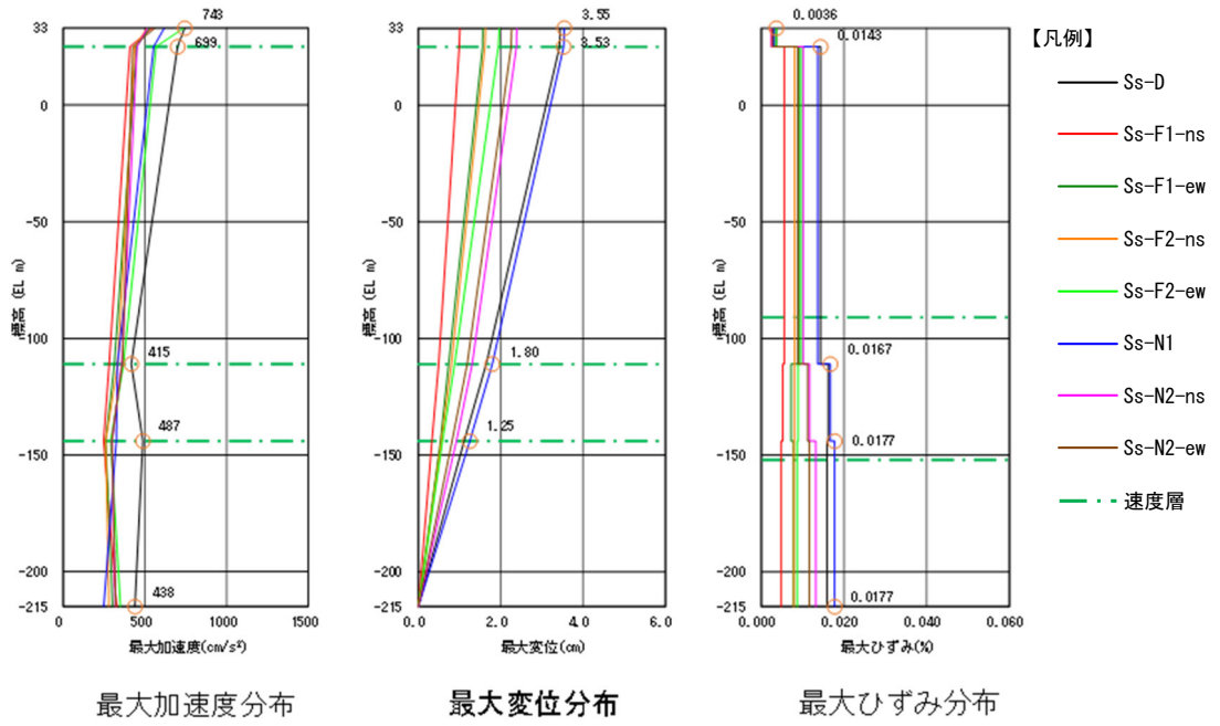
図 5(1) 第 3 保管エリア東側（水平方向）
