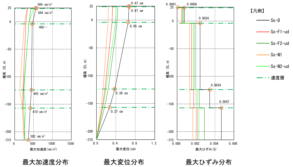
図4(2) 第3保管エリア西側（鉛直方向）
