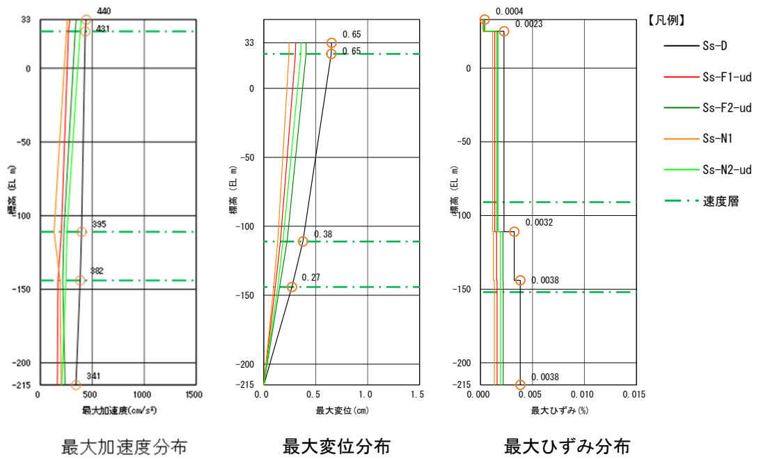
図 5(2) 第 3 保管エリア東側（鉛直方向）
