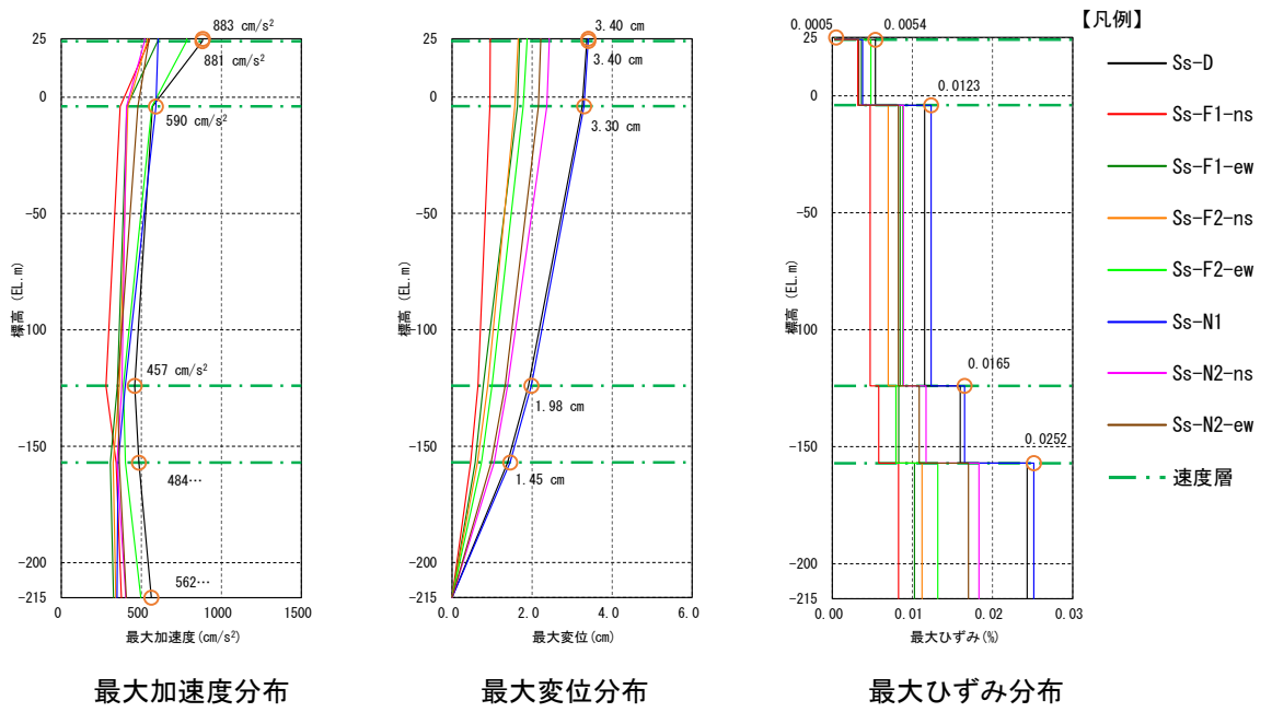
図4(1) 第3保管エリア西側（水平方向）
