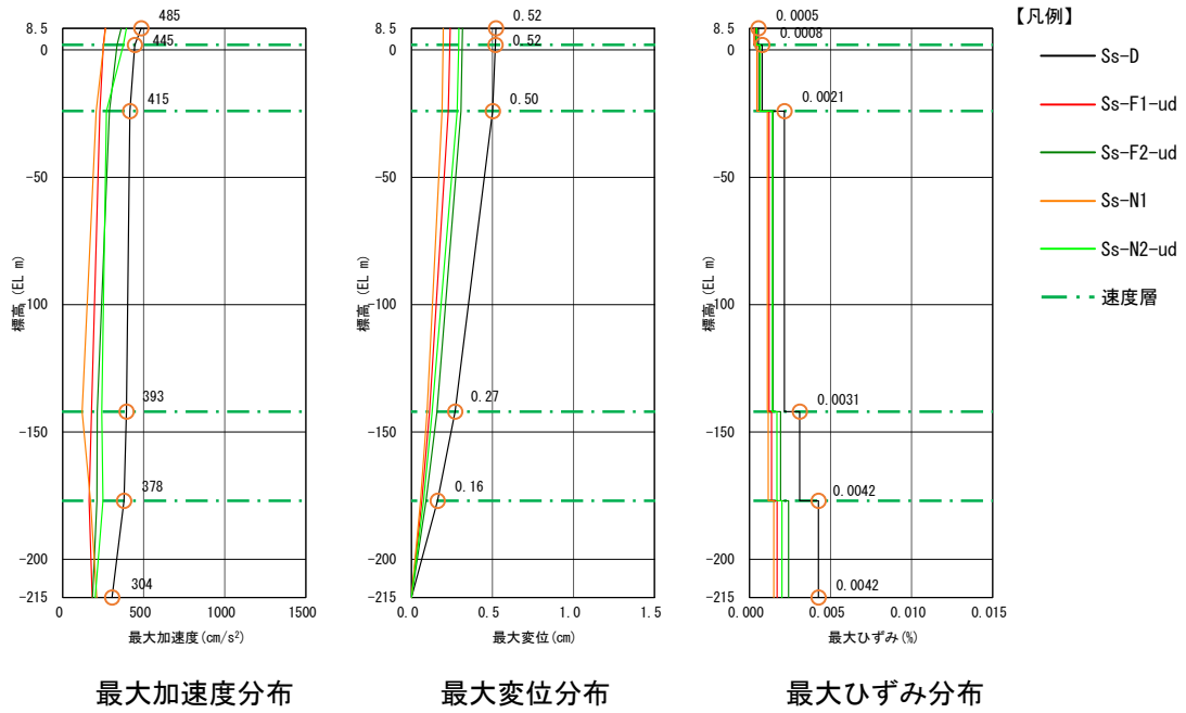
図 6(2) 第 4 保管エリア北側 (鉛直方向)
