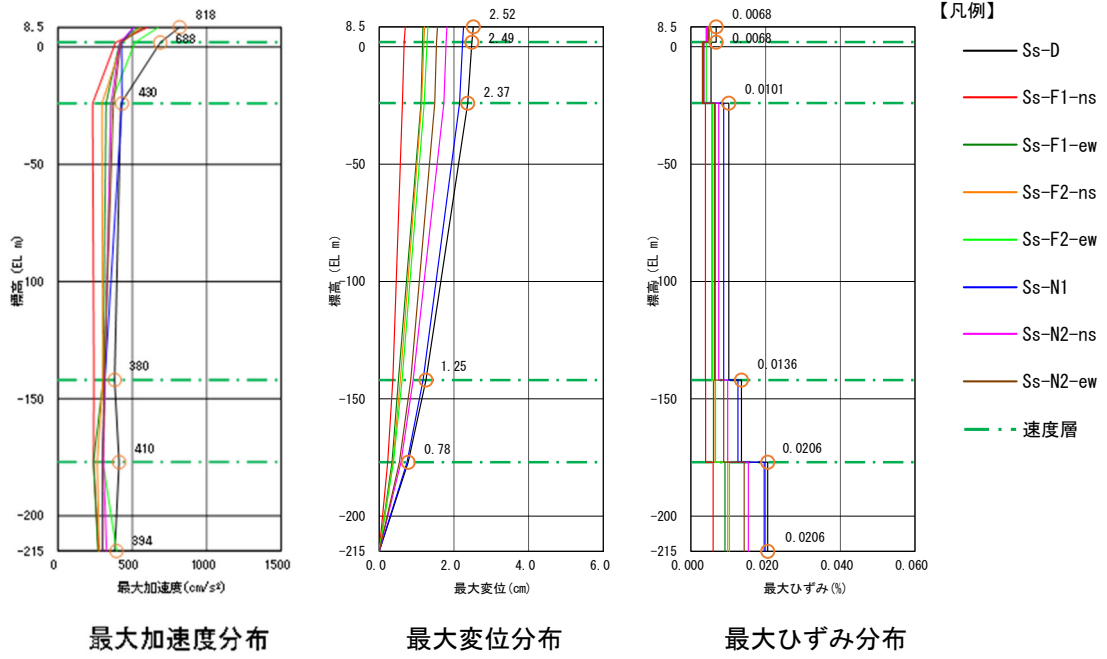
図 6(1) 第 4 保管エリア北側 (水平方向)
