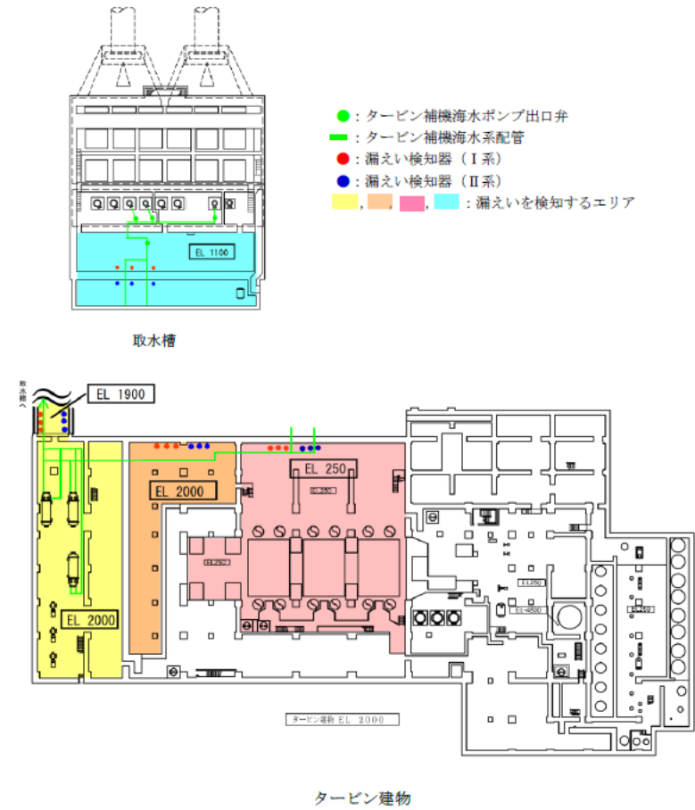
図 4-3 漏えい検知器及びタービン補機海水ポンプ出口弁配置図
