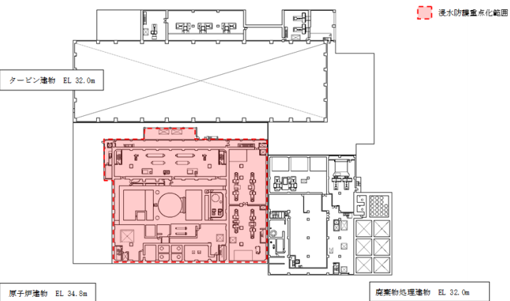
図 3-29(3) 浸水防護重点化範囲 (平面図) (3/4)
