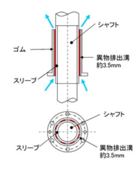
図 3-38 海水ポンプ軸受構造図
