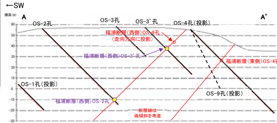
断面図(H:V=1:1)
