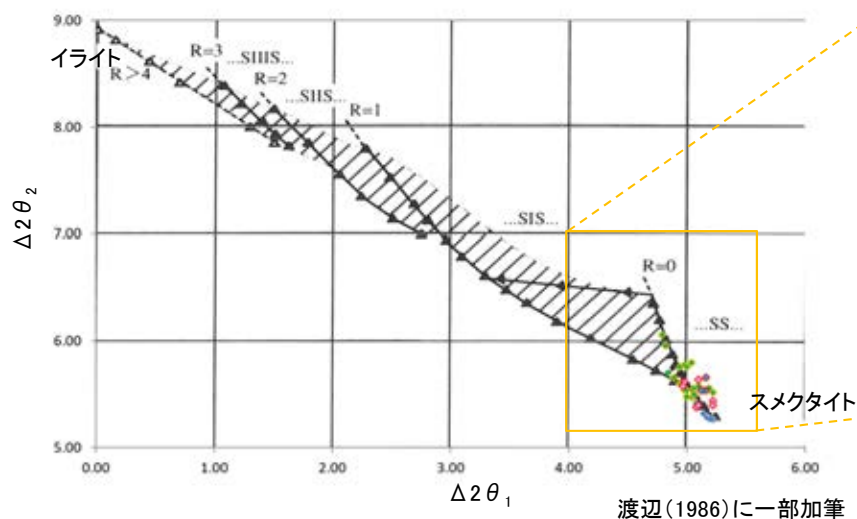
渡辺(1986)に一部加筆
