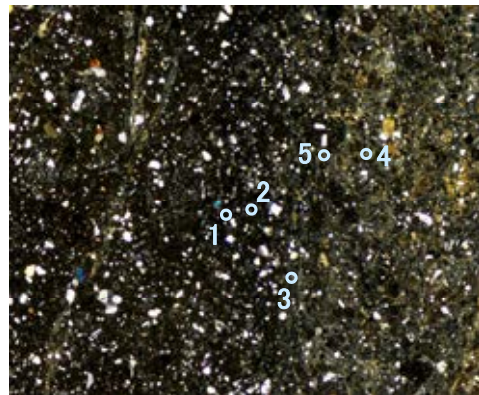
直交ニコル
