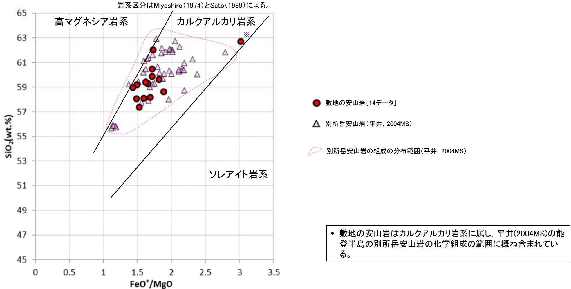
能登半島と敷地における火山岩の主要成分(FeO*/MgO図)※ ※I-9-1のプロット位置を適正化。 分析値は、100%ノーマライズしたものを使用して作図した。
