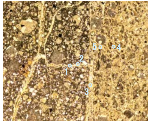
単ニコル
