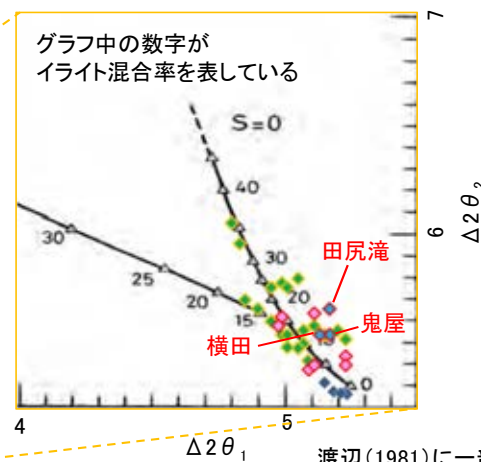
渡辺(1981)に一部加筆
