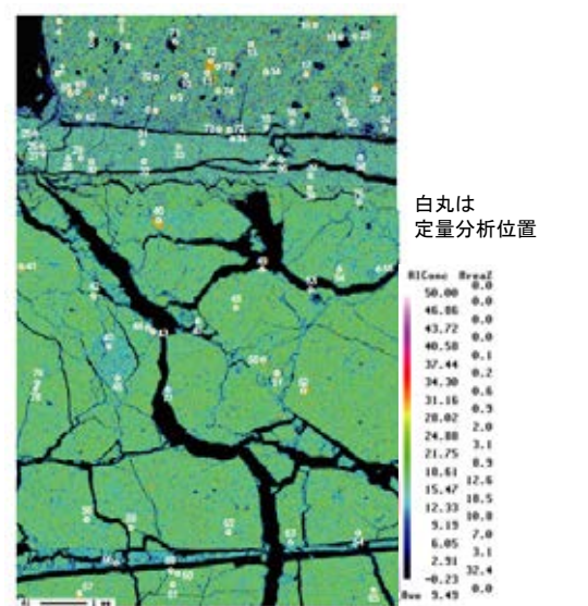
EPMAマッピング(AI)
