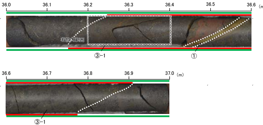
K-2写真(H-0.9-75孔)
