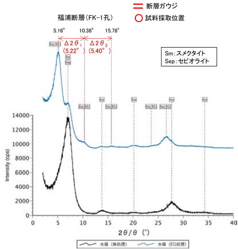
X線回折チャート(定方位)
