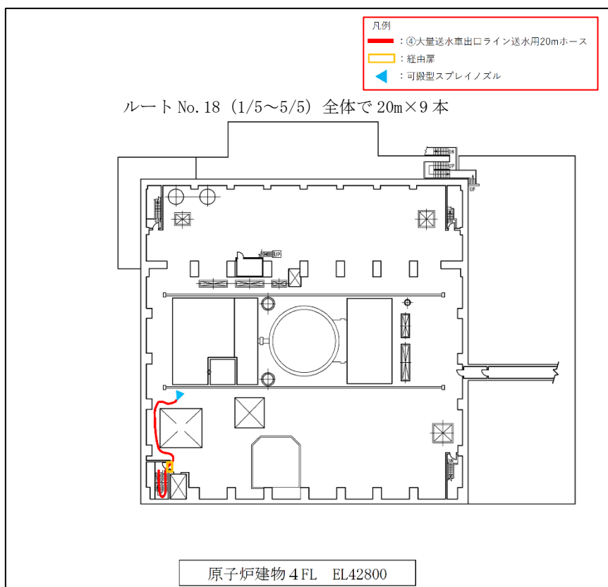
図 1-18 ホース敷設ルート No. 18(5/5)
