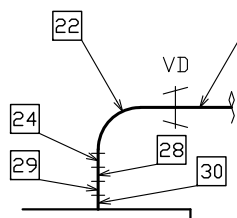
A~A矢視図
