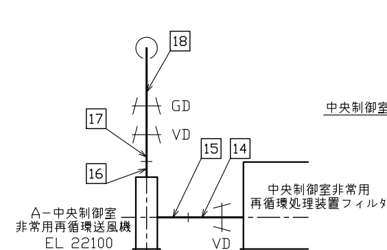
J~J矢視図
