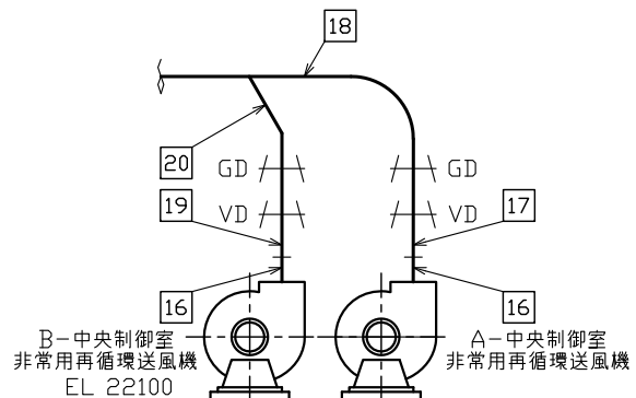
I~I矢視図
