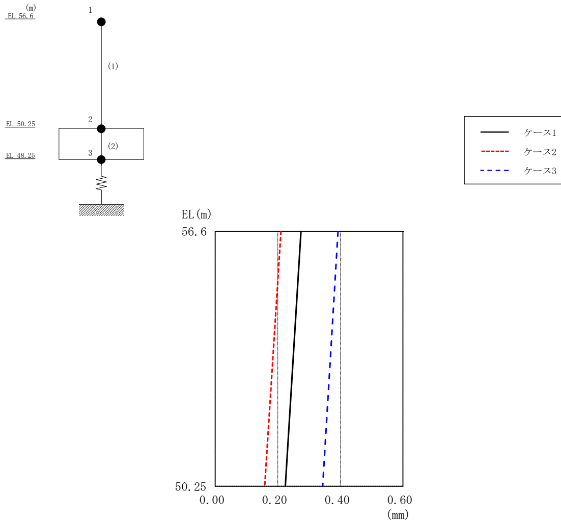
図 2-10 最大応答変位 (基準地震動 S s -D, 鉛直方向)
