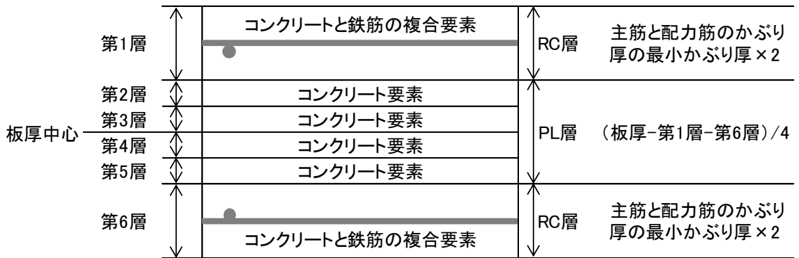
図 3-9 非線形シェル要素の概念図
