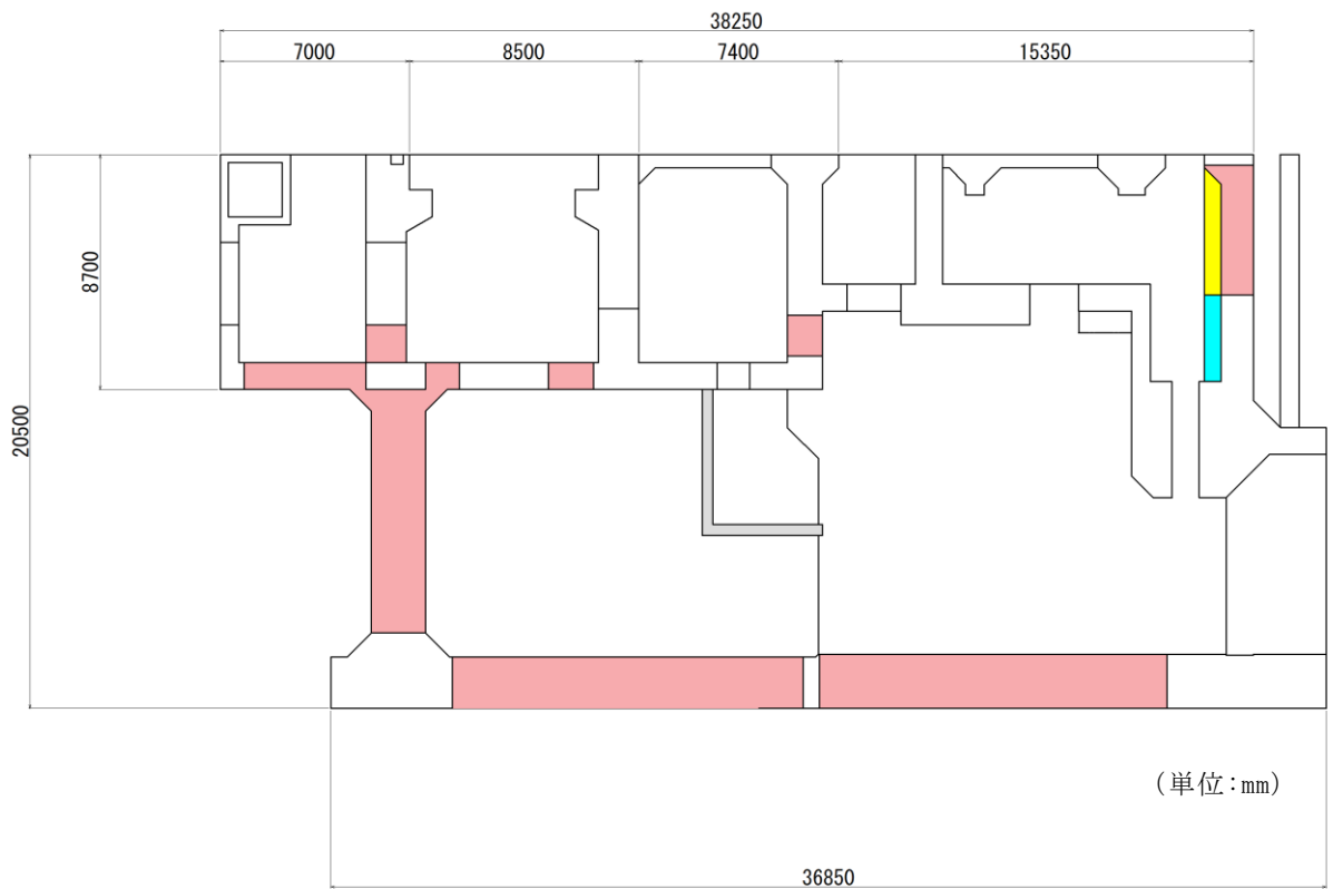
図 2-16 せん断補強計画図 (D-D断面)
