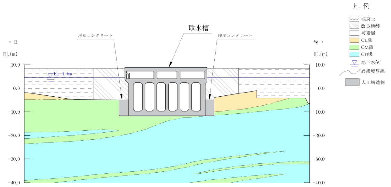
図 3-2 取水槽 地震時荷重算出用地質断面図 (A-A 断面)
