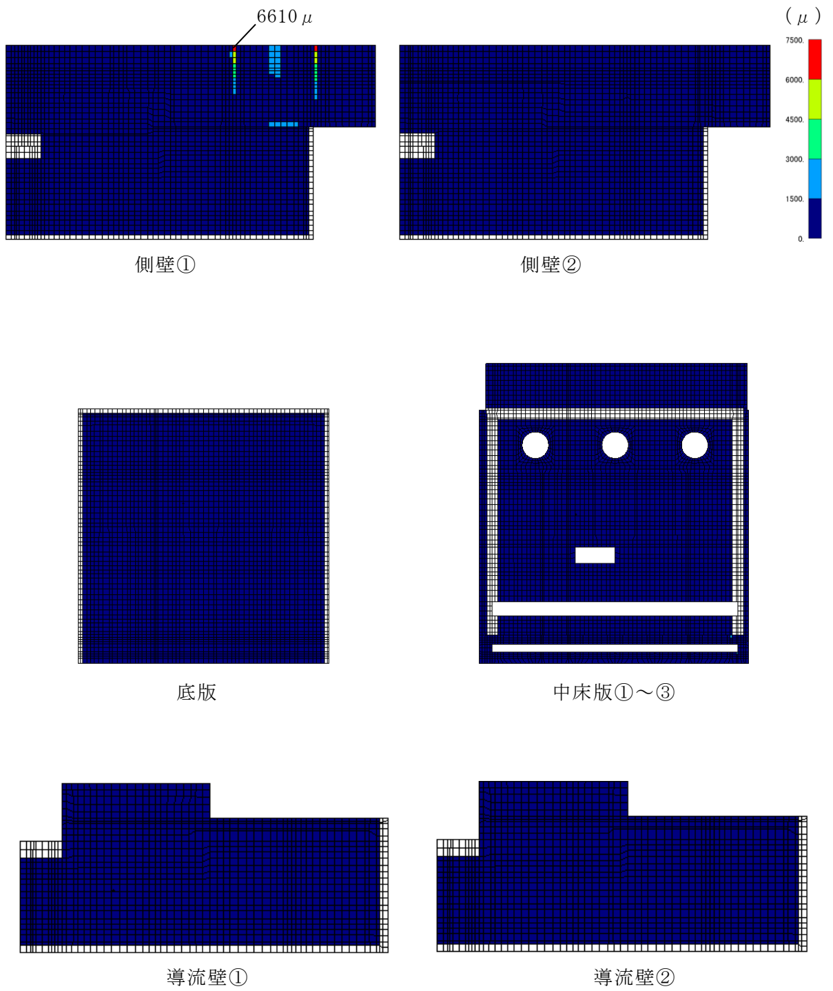
図 4-4 (1) 曲げ・軸力系の破壊に対する照査値最大時のひずみ分布図 (コンクリートの圧縮縁ひずみ) (側壁, 解析ケース④, S_s - D (-+) )
