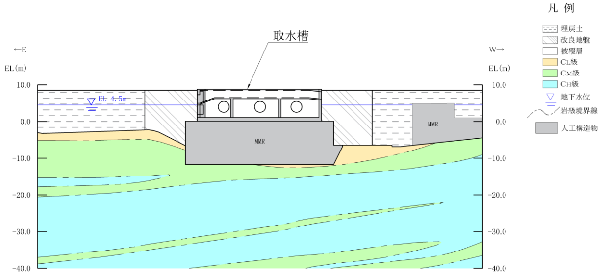
図 3-4 取水槽 地震時荷重算出用地質断面図 (C-C断面)
