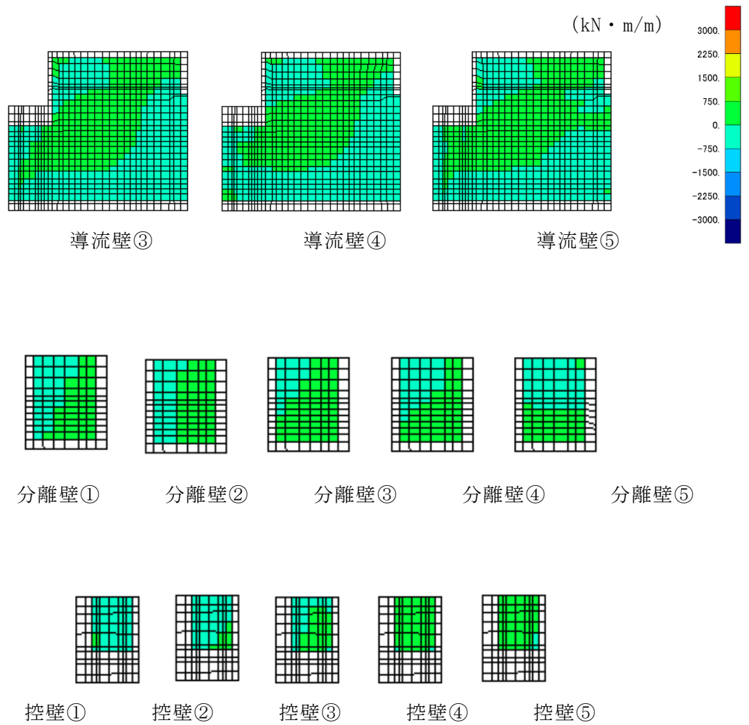
図 4-12 (2) せん断破壊に対する照査値最大時の断面力分布図
