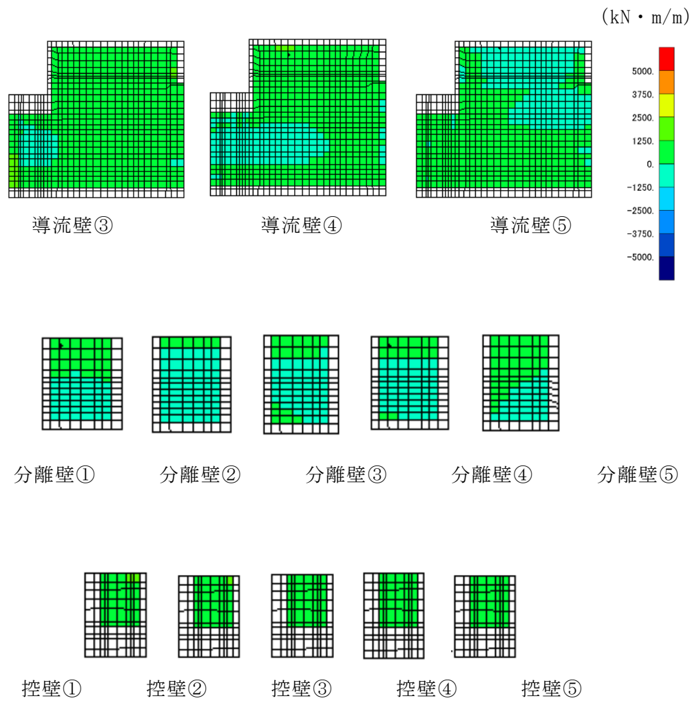
図 4-10 (2) せん断破壊に対する照査値最大時の断面力分布図
