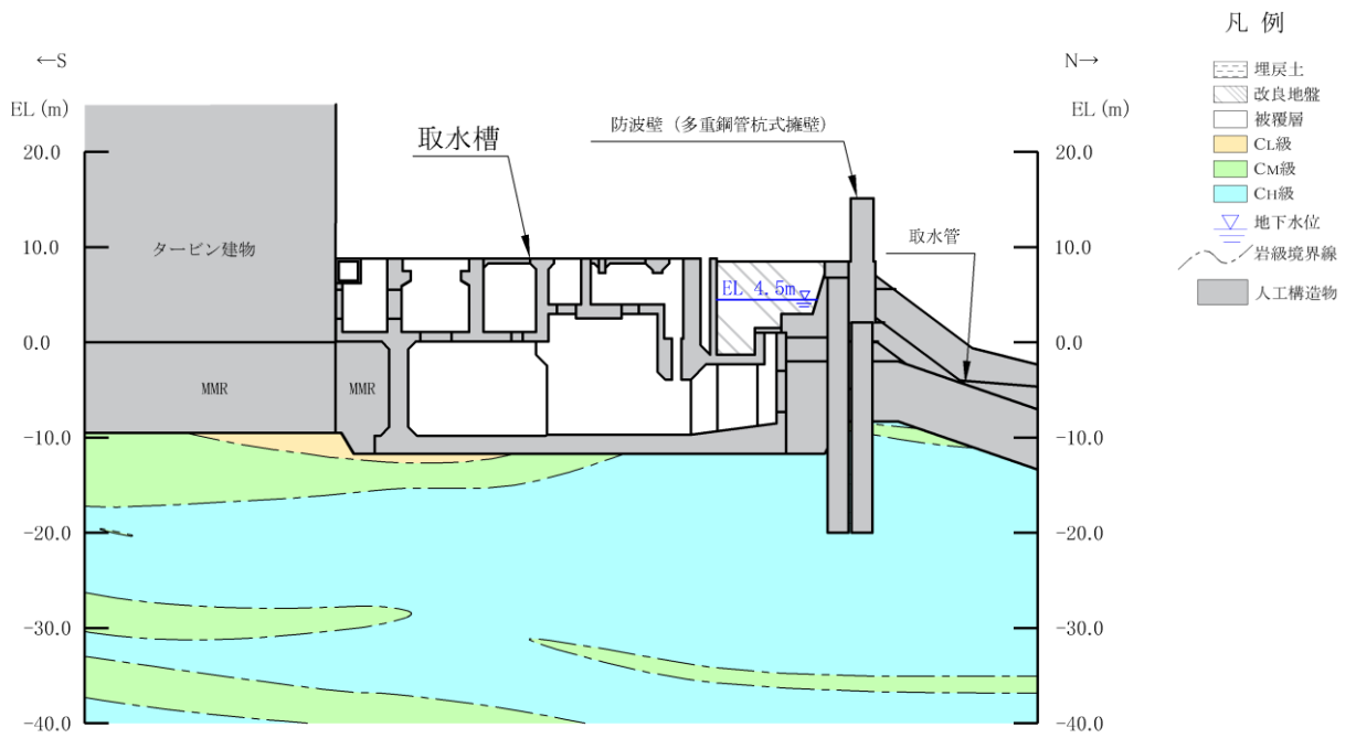
図 3-5 取水槽 地震時荷重算出用地質断面図 (D-D断面)
