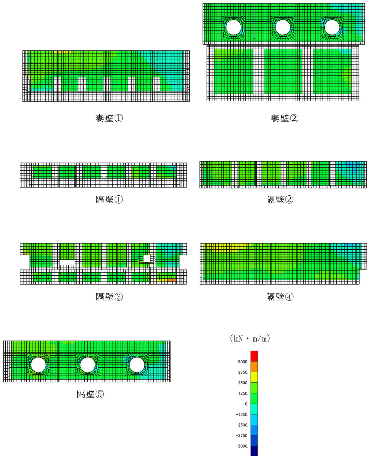
図 4-9 (3) せん断破壊に対する照査値最大時の断面力分布図
