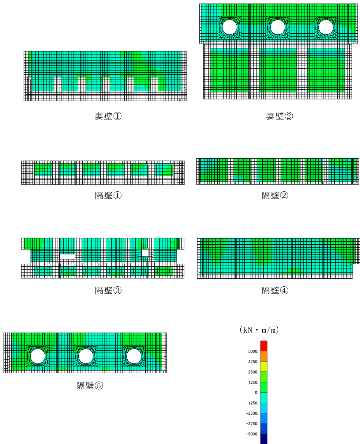
図 4-8 (3) せん断破壊に対する照査値最大時の断面力分布図 (曲げモーメント ( \text{kN} \cdot \text{m} ) : M_y ) (側壁, 解析ケース②, S_s - D (-+) )
